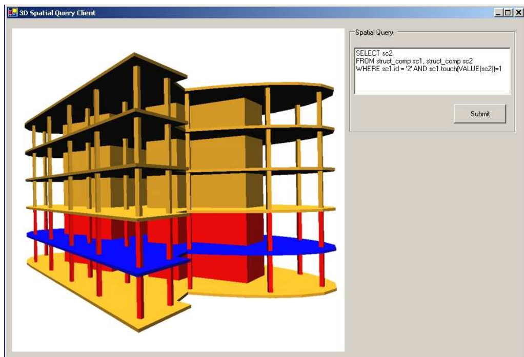
Abbildung 9.13: Die Anwendung des Operators touch für das blau markierte Deckenbauteil (Bauteil 2) liefert die rot markierte Ergebnismenge. Die Anfrage wird von der Datenbank in 7.2s bearbeitet, wobei der in Abschnitt 8.5 beschriebene Algorithmus zum Einsatz kommt, wiederum ohne vorgeschaltete Bounding Box -Tests. Das Hardware-Setup ist identisch zu dem von Abb. 9.13.
