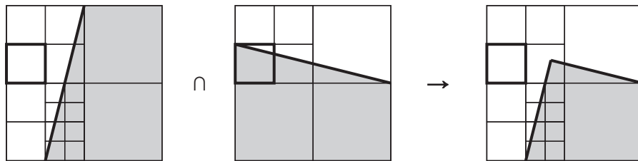
Abbildung 8.6: Verschneidung zweier Oktalbäume während ihres Aufbaus. Durch parallele Abarbeitung der Bäume und direkte Auswertung des Verschneidungsausdrucks können unnötige Verfeinerungen vermieden werden. Als Ergebnis der Verschneidung der umrahmten Zellen in den Eingangsbäumen ergibt sich die Farbbelegung \text{weiß} \cup \text{grau} \Rightarrow \text{weiß} . Eine Verfeinerung des zweiten Eingangsbauers ist an dieser Stelle daher nicht notwendig. Abbildung entnommen aus (Mundani, 2005).
