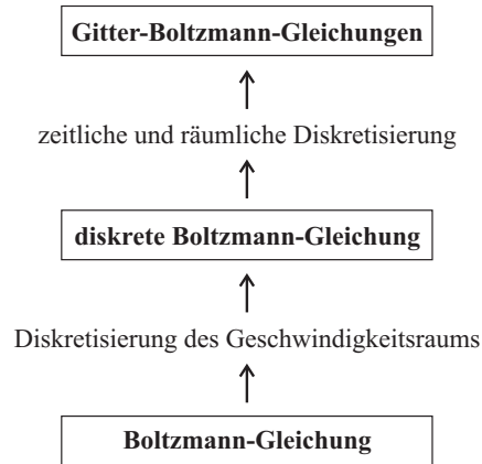
Abbildung 5.1: Zweistufige Diskretisierung der kontinuierlichen Boltzmann-Gleichung. Ergebnis ist die Gitter-Boltzmann-Gleichung.
