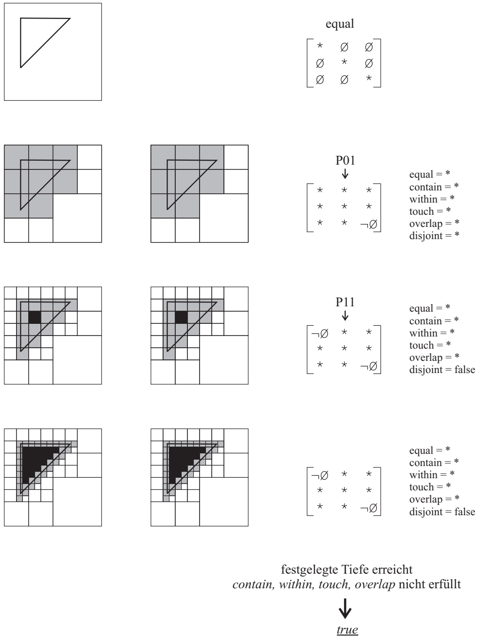
Abbildung 8.32: 2D-Darstellung der Untersuchung einer equal -Situation für nicht-dimensions-reduzierte Objekte auf den Ebenen 2 bis 4. Auch bei beliebiger Verfeinerung werden equal -Situationen nie ganz aufgelöst, da sie mit contain , within , touch und overlap konkurrieren. Daher gilt equal bei Erreichen der maximalen Verfeinerung als erfüllt, wenn kein anderes Prädikat bestätigt werden kann. Dies gilt analog im 3D-Raum für Body -Objekte.
