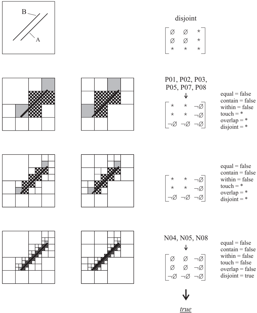
Abbildung 8.36: 2D-Darstellung der Untersuchung einer disjoint -Situation für dimensionsreduzierte Objekte auf den Ebenen 2 bis 4. Die disjoint -Situation wird auf Ebene 4 korrekt aufgelöst. Entsprechend der Prädikatenhierarchie gilt auf den vorhergehenden Ebenen das Prädikat touch . Das Beispiel gilt analog im 3D-Raum für beliebige Kombinationen aus Surface -, Line - und Point -Objekten.
