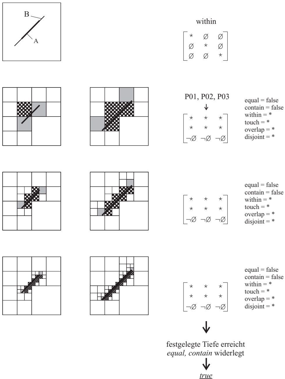
Abbildung 8.39: 2D-Darstellung der Untersuchung einer within -Situation für dimensionsreduzierte Objekte auf den Ebenen 2 bis 4. within -Situationen dimensionsreduzierter Objekte werden nie aufgelöst. Entsprechend wird der positivistische Ansatz in Verbindung mit der Hierarchie der topologischen Prädikate von Abb. 8.23 angewandt: Bei Erreichen der maximalen Verfeinerungsstufe gilt within als erfüllt, wenn equal und contain widerlegt sind. Dies gilt analog im 3D-Raum für beliebige Kombinationen aus Surface -, Line - und Point -Objekten.
