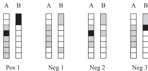
Abbildung 8.16: Drei Beispielkonfigurationen, bei denen die Regeln Pos , Neg1 , Neg2 bzw. Neg3 im Fall von isAboveStrict(A,B) angewendet werden.
