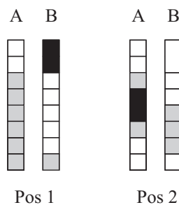
Abbildung 8.17: Beispiele für Konstellationen, bei denen die Regeln Pos1 bzw. Pos2 im Fall von isAbove(A,B) angewendet werden.
