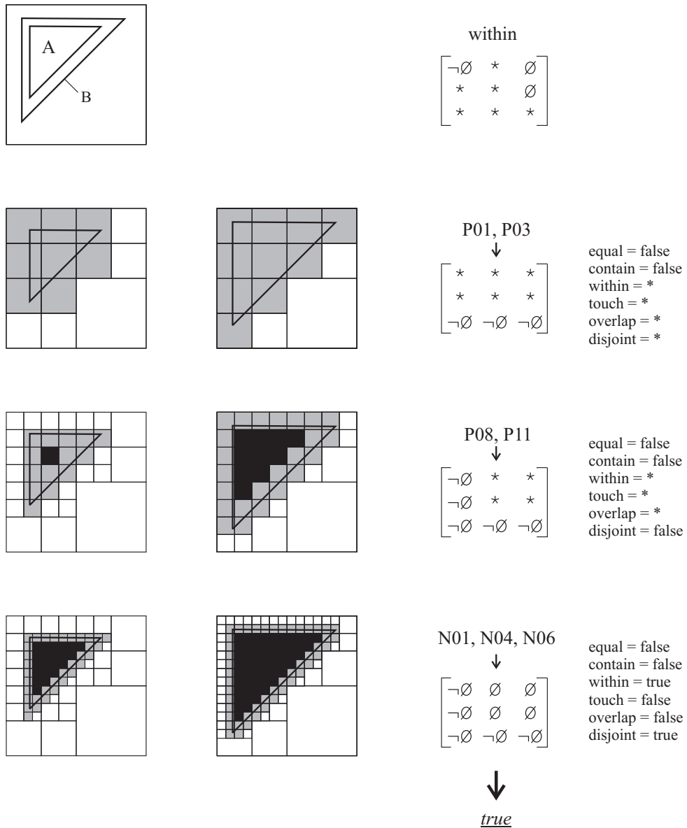
Abbildung 8.31: 2D-Darstellung der Untersuchung einer within -Situation für nicht-dimensi- onsreduzierte Objekte auf den Ebenen 2 bis 4. Die within -Situation für 2D- Regionen wird auf Ebene 4 korrekt aufgelöst. Dank des positivistischen An- satzes in Verbindung mit der Prädikatenhierarchie gilt within jedoch bereits auf den vorhergehenden Ebenen. Das Beispiel gilt analog im 3D-Raum für Body -Objekte.
