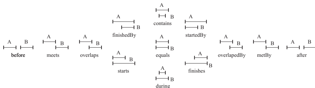
Abbildung 7.16: Die 13 von Allen identifizierte Intervallrelationen in 1D.
