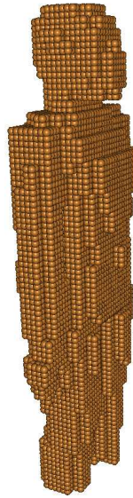
Abbildung 5.4: Ergebnis der Diskretisierung einer Dummy-Geometrie. Aus Gründen der besseren Darstellbarkeit werden die als Hindernis markierten Voxel kugelförmig dargestellt.
