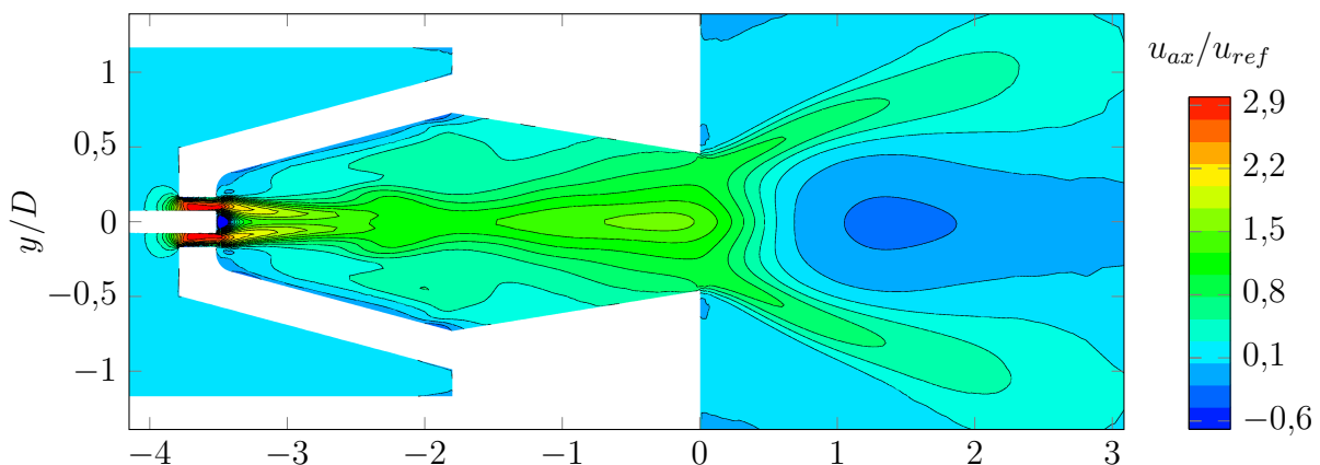
Abbildung 5.7: A 2 EV-Brenners mit zwei Schlitzen, Variante fünf (Nr. 5 in Tabelle 1.1)
