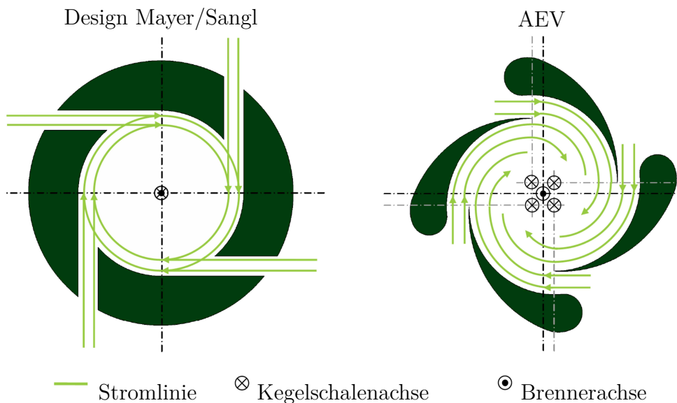
Abbildung 5.1: Prinzip der Drallerzeugung von A 2 EV-Brenner und AEV [63]
