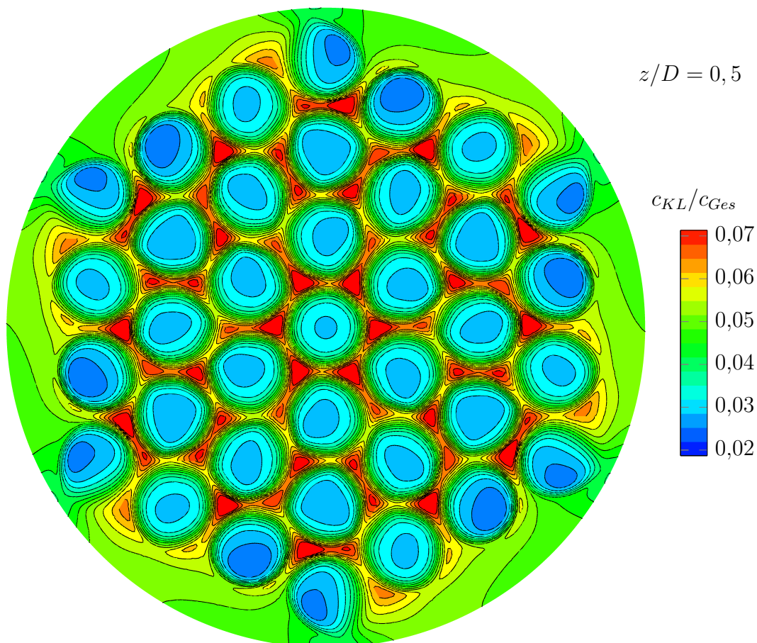
Abbildung 6.16: Kühlluftkonzentration in der gesamten Brennkammer bei Position z/D = 0,5
