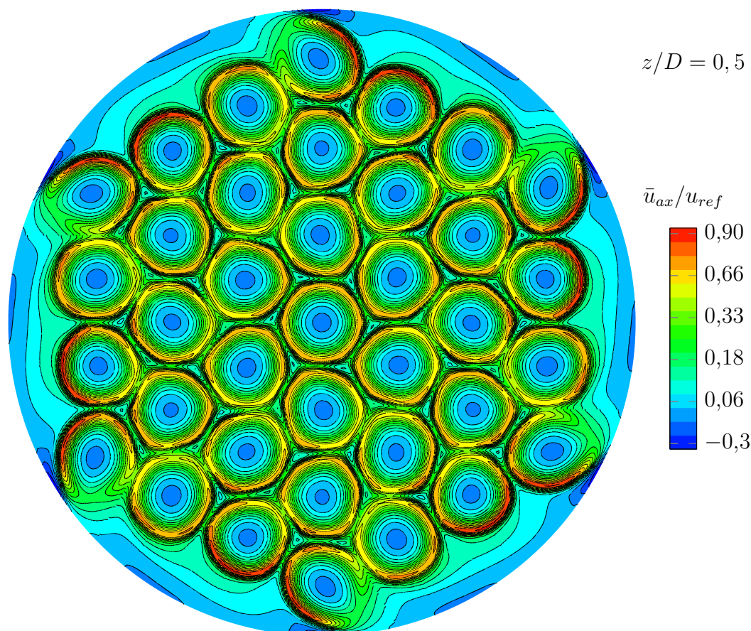
Abbildung 6.10: Axialgeschwindigkeitsfeld in der gesamten Brennkammer bei Position z/D = 0,5
