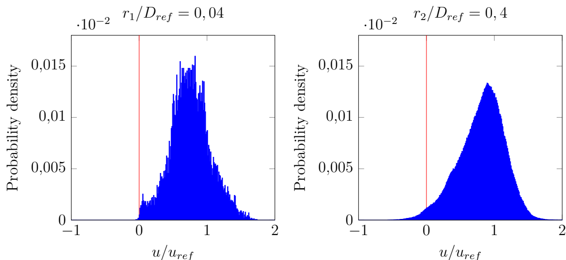
Abbildung 5.46: PDF der Axialgeschwindigkeit am Brenneraustritt des Prototypbrenners ohne Kopfaufsatz innerhalb von r_1/D_{ref} = 0,04 (links) und von r_2/D_{ref} = 0,4 (rechts)
