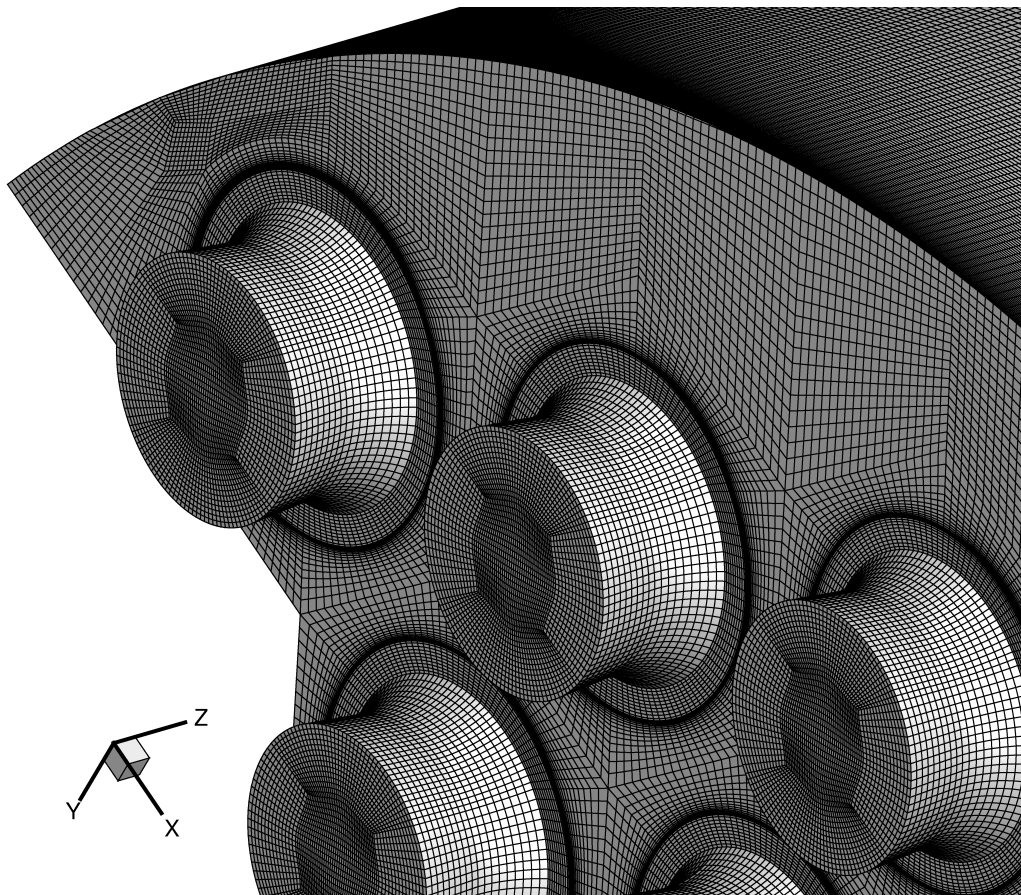
Abbildung 2.14: Numerisches Gitter für die Berechnung der Mehrbrenneranordnung
