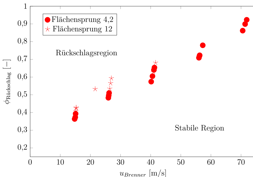
Abbildung 5.35: Rückschlagsgrenzen des kleiner skalierten A 2 EV-Brenners (Nr. 2 in Tabelle 1.1) im kleinen Prüfstand mit kleinem Plenum bei einem Flächensprung von 4,2 und 12 bei p = 1\text{bar} , T_{Luft} = 673\text{K} und H_2 als Brennstoff
