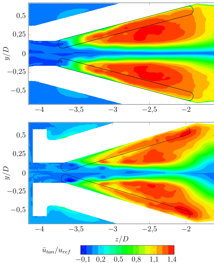
Abbildung 5.28: Mittleres Tangentialgeschwindigkeitsfeld des A 2 EV-Brenners (oben) und des Prototypbrenners (unten) mit auf die Darstellungsebene projizierten Schlitzpositionen
