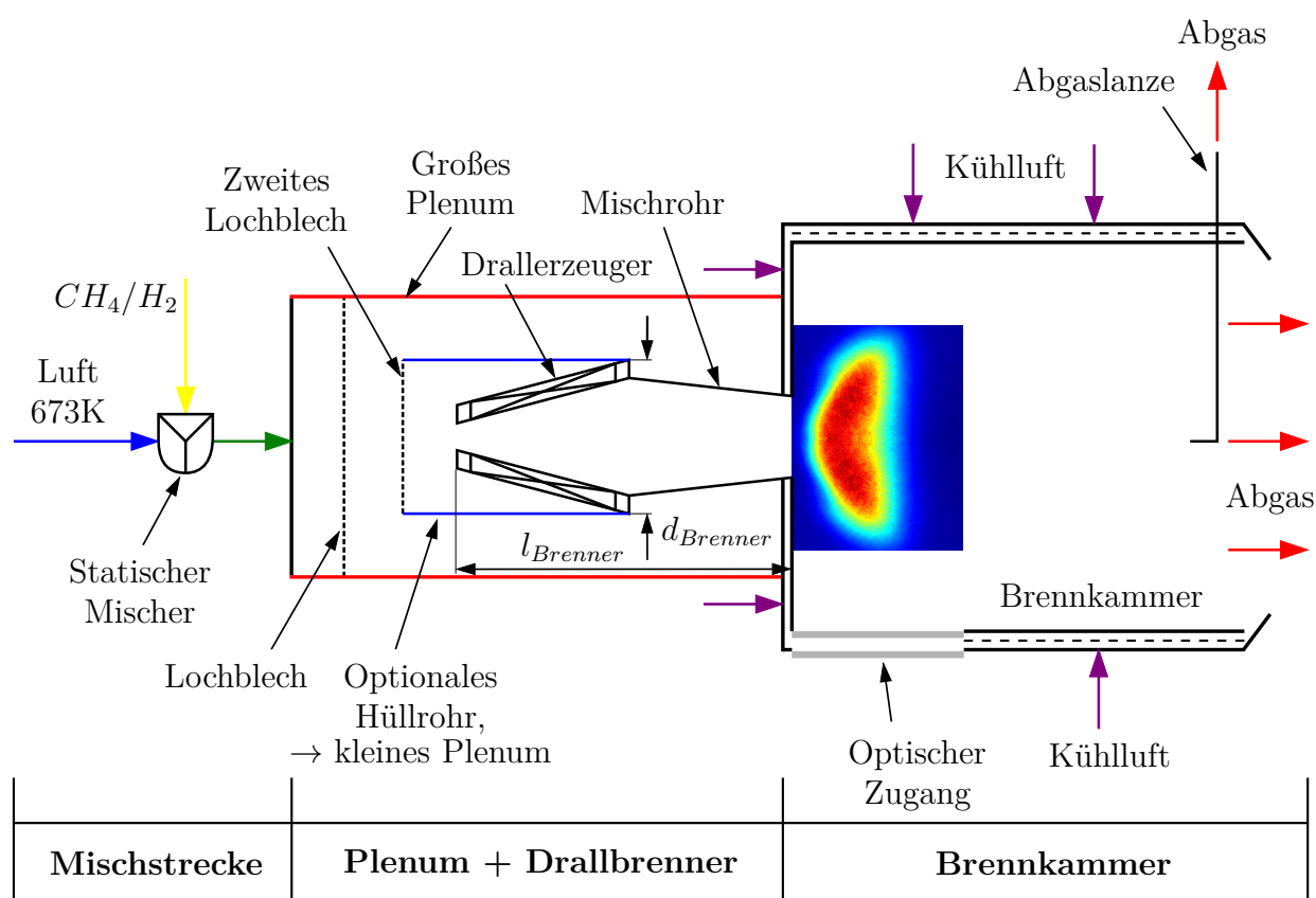
Abbildung 3.2: Schematischer Aufbau des Verbrennungsprüfstands für Brenner in Maschinengröße
