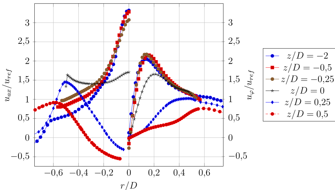
Abbildung 4.7: Profile der normierten mittleren Axial- und Tangentialgeschwindigkeit mit 1% Kernströmung
