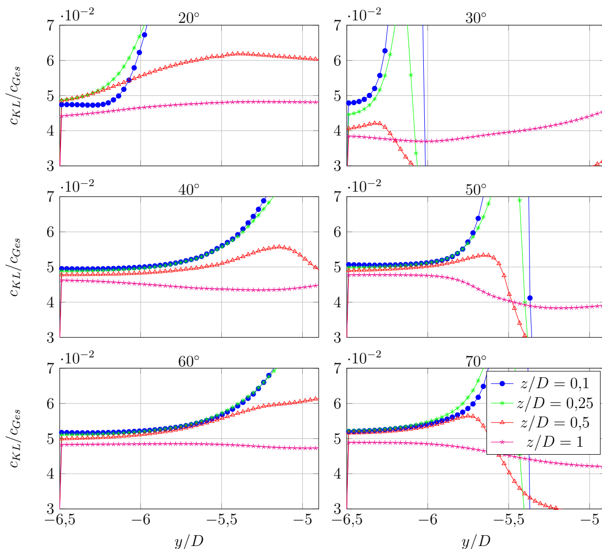
Abbildung 6.17: Profile der Kühlluftkonzentration an verschiedenen Rotationswinkelpositionen
