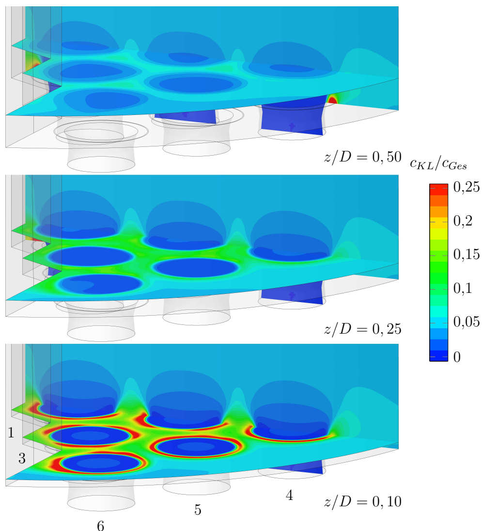
Abbildung 6.13: Kühlluftkonzentration in axialen Schnitten in der Silobrennkammer
