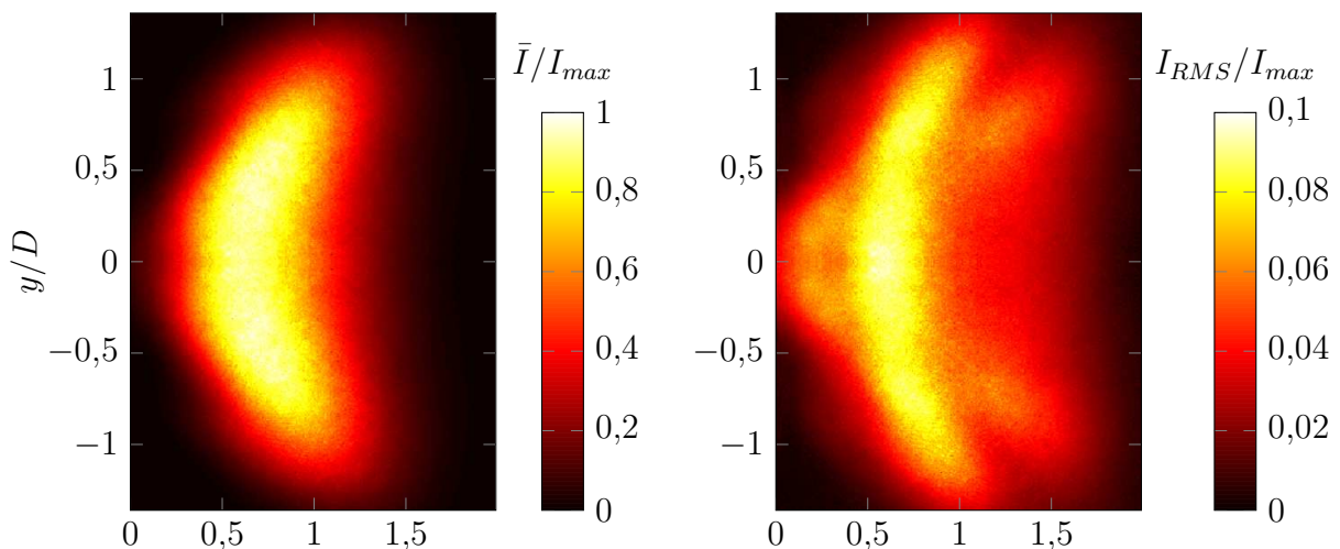
Abbildung 5.16: Normierte mittlere Intensität (links) und normierte RMS-Intensität (rechts) der OH*-Chemilumineszenz von stationären Verbrennungsversuchen des Prototypbrenners mit Erdgas bei T = 673K , u_{ref} = 47m/s und \phi = 0,71
