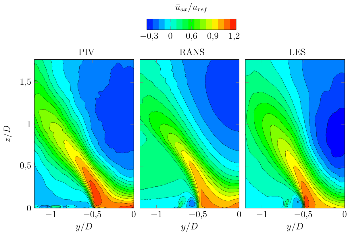
Abbildung 6.3: Mittlere Axialgeschwindigkeit von PIV, RANS und LES in der Brennkammer
