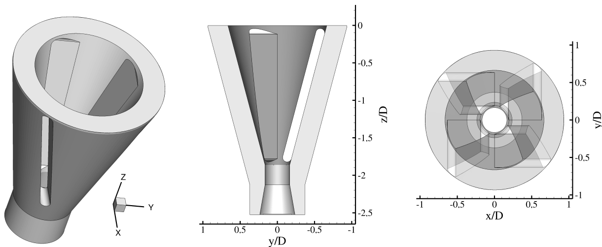
Abbildung 5.10: A 2 EV-Brenner mit 4 Schlitten (Nr. 2 in Tabelle 1.1)
