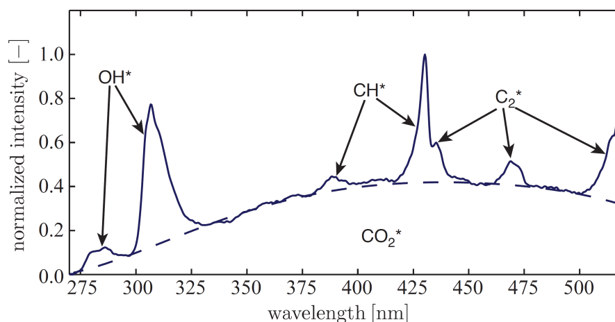
Abbildung 3.4: Typisches Spektrum einer turbulenten Erdgasflamme bei atmosphärischem Druck [44]
