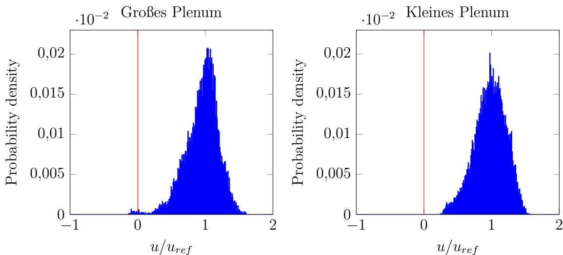
Abbildung 5.44: PDF der Axialgeschwindigkeit innerhalb von r_1 = 0,04 D_{ref} am Brenneraustritt des A 2 EV-Brenners mit großem (links) und kleinem Plenum (rechts)
