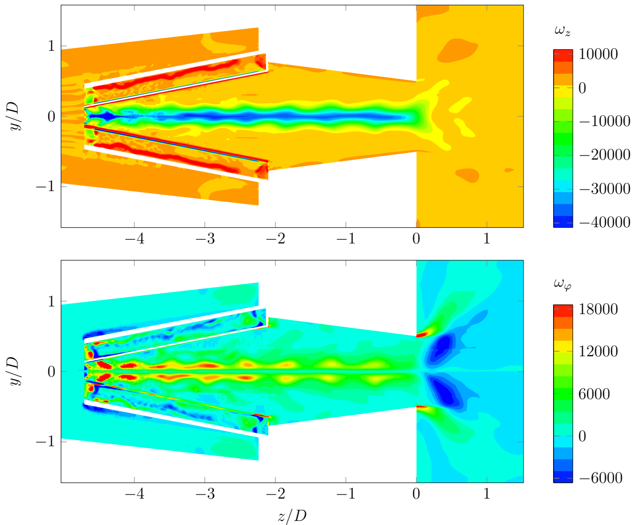
Abbildung 4.8: Axiale und azimuthale Wirbelstärke des modifizierten EV-Brenners
