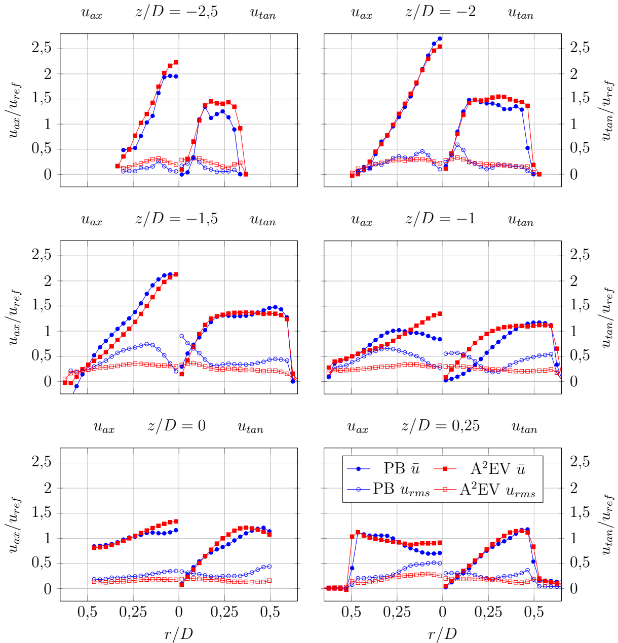
Abbildung 5.24: Profile der normierten mittleren und RMS-, Axial- und Tangentialgeschwindigkeit von Prototyp- (PB) und A 2 EV-Brenner (A 2 EV)
