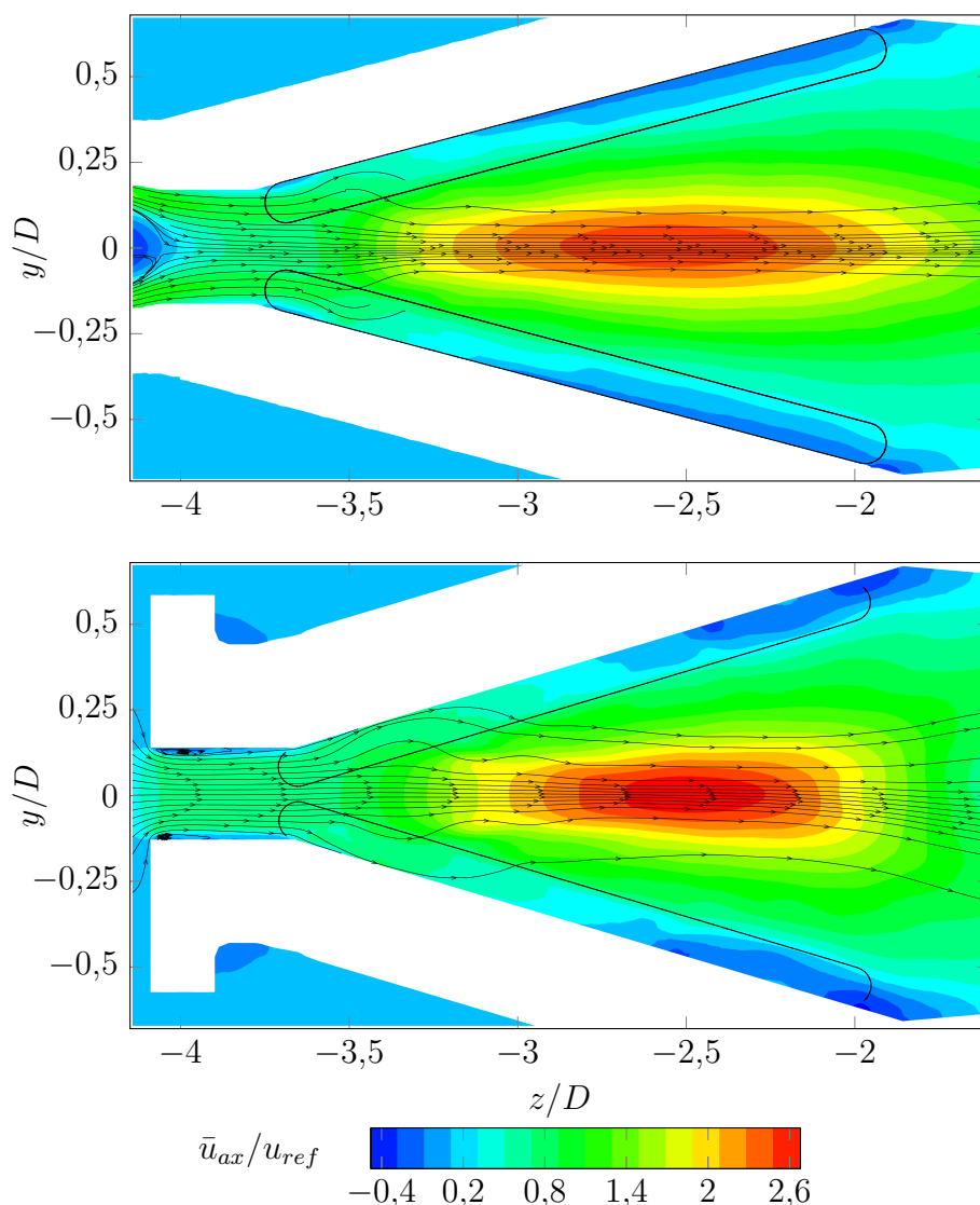
Abbildung 5.27: Mittleres Axialgeschwindigkeitsfeld mit Stromlinien des A 2 EV-Brenners (oben) und des Prototypbrenners (unten) mit auf die Darstellungsebene projizierten Schlitzpositionen
