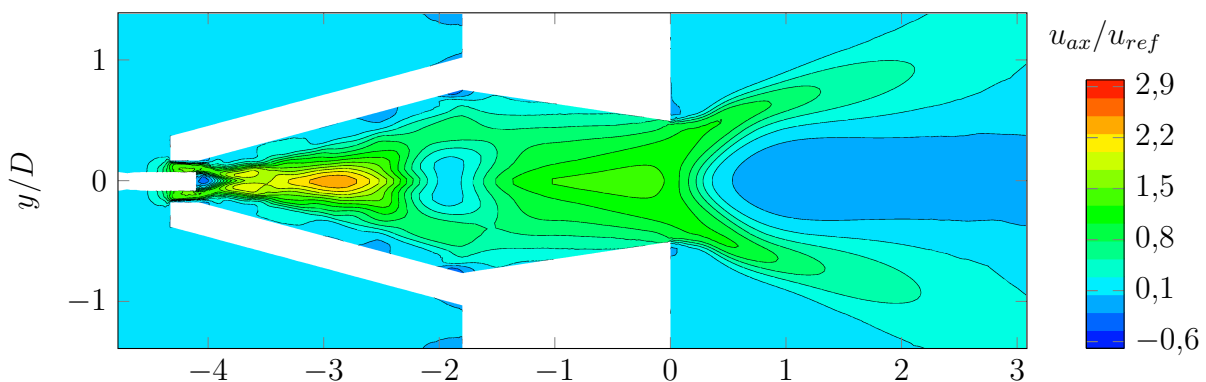
Abbildung 5.6: Variante vier des A 2 EV-Brenners mit zwei Schlitzen mit vorzeitigem Wirbelaufplatzen (Nr. 4 in Tabelle 1.1)
