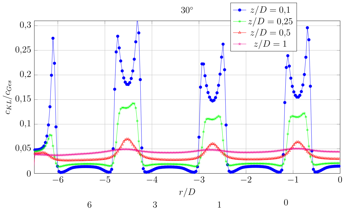
Abbildung 6.14: Profile der Kühlluftkonzentration an verschiedenen axialen Positionen durch Brenner 6, 3, 1, und 0
