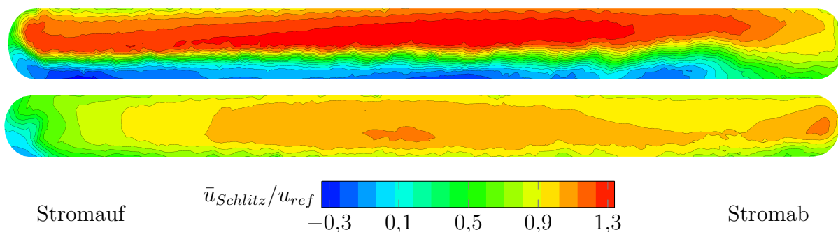
Abbildung 5.29: Mittlere Schlitzgeschwindigkeitsfeld des A 2 EV-Brenners (oben) und Prototypbrenners (unten), Hauptströmungsrichtung von links nach rechts
