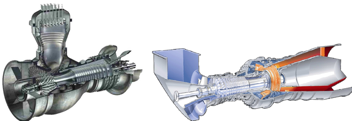
Abbildung 2.7: Gasturbine mit Silobrennkammer (links, Quelle: Alstom Power) und mit Ringbrennkammer (rechts, Quelle: Siemens AG)
