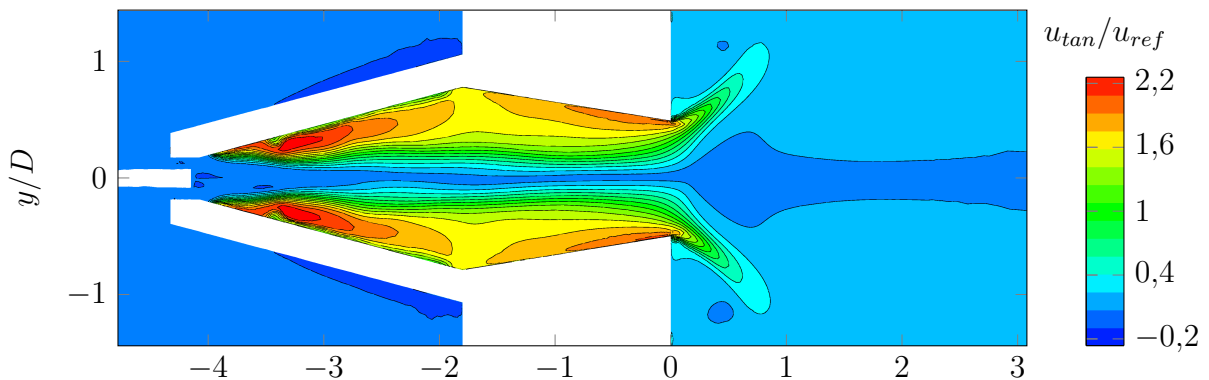
Abbildung 5.4: Tangentialgeschwindigkeit des A 2 EV-Brenners mit zwei Schlitzten, Variante drei (Nr. 3 in Tabelle 1.1)
