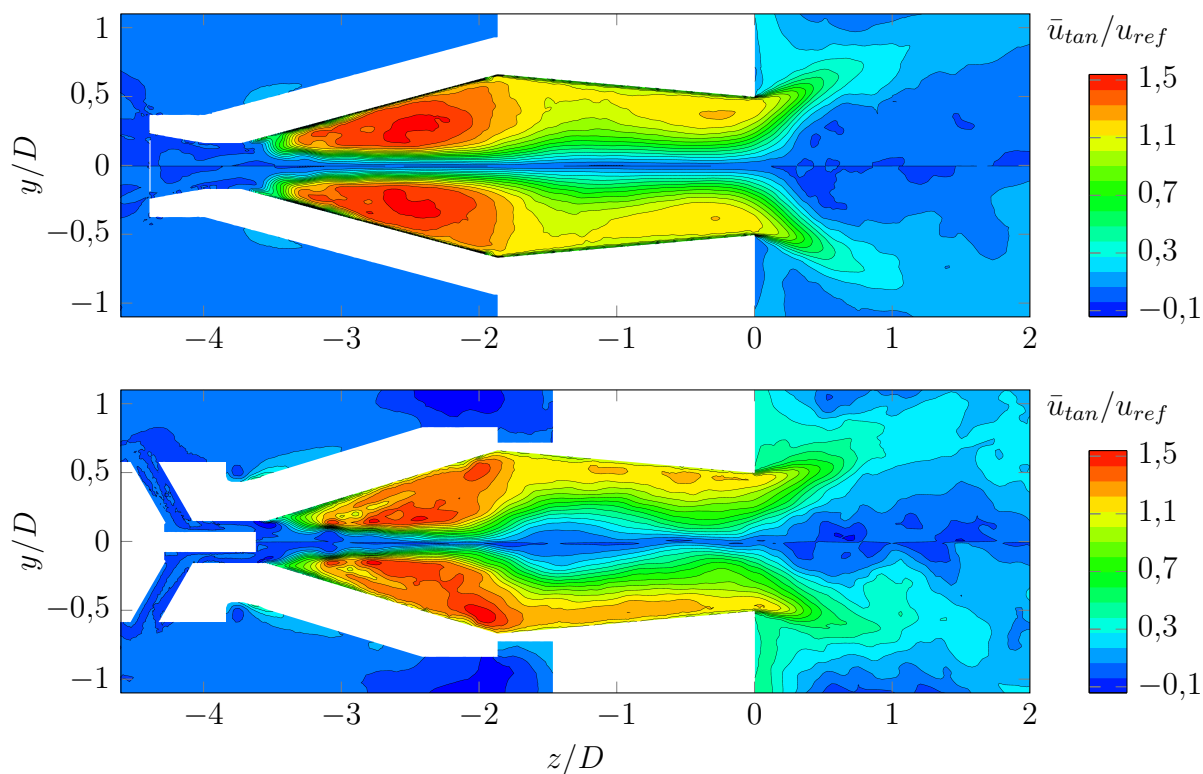
Abbildung 5.22: Mittleres Tangentialgeschwindigkeitsfeld des A 2 EV-Brenners (oben) und des Prototypbrenners (unten)
