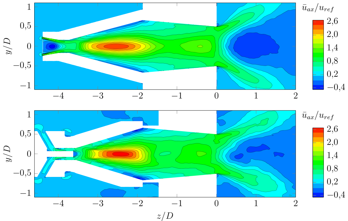
Abbildung 5.21: Mittleres Axialgeschwindigkeitsfeld des A 2 EV-Brenners (oben, Nr. 2 in Tabelle 1.1) und des Prototypbrenners (unten, Nr. 7 in Tabelle 1.1)
