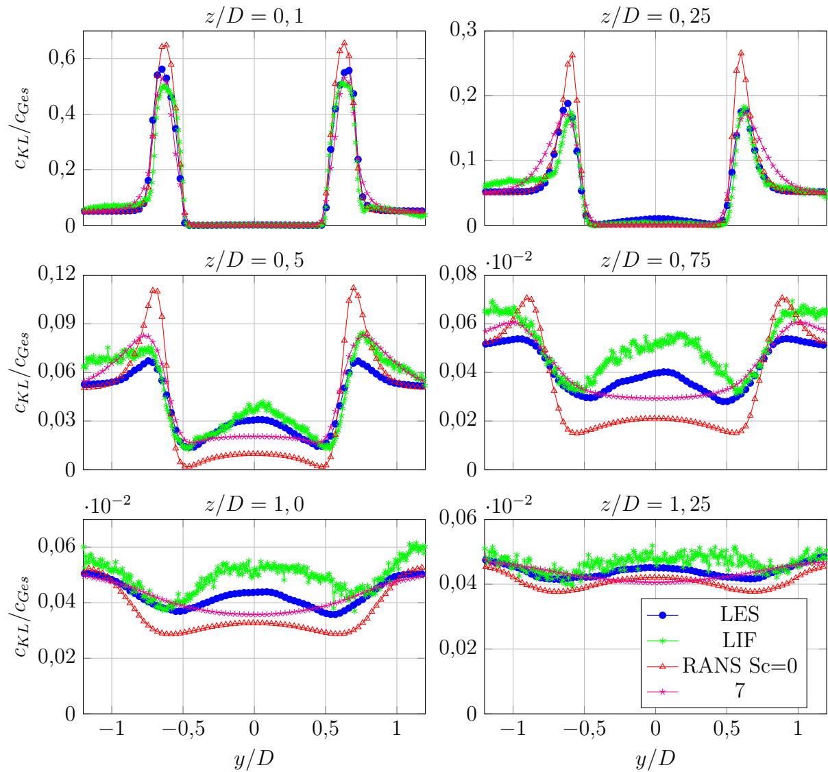
Abbildung 6.6: Profile der mittleren Kühlluftkonzentration an verschiedenen axialen Positionen von LES, RANS und Experiment (PIV)
