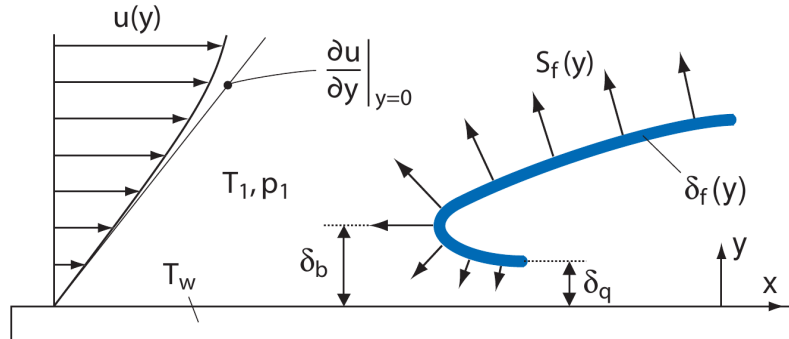
Abbildung 2.10: Schematische Darstellung des Flammenrückschlags durch die Wandgrenzschicht nach dem Gradientenmodell, [15], [47]
