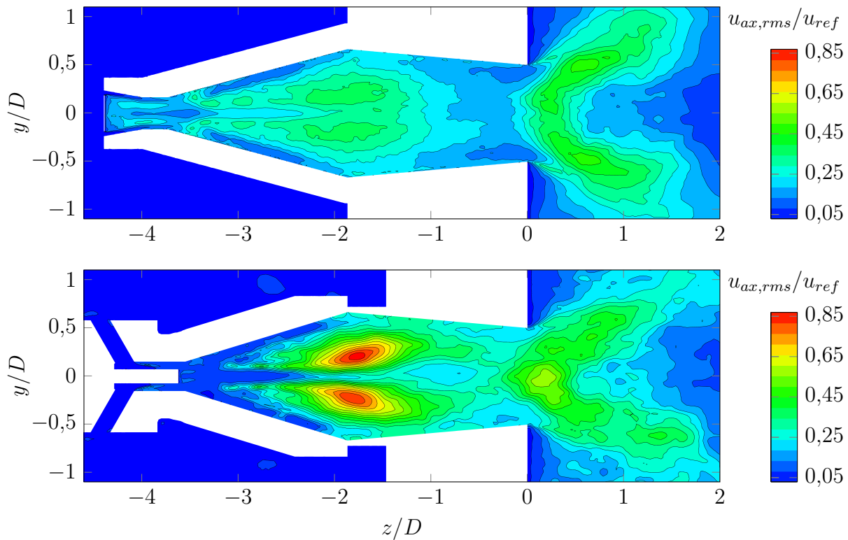
Abbildung 5.23: RMS der Axialgeschwindigkeit des A 2 EV-Brenners (oben) und des Prototypbrenners (unten)
