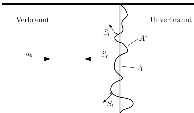
Abbildung 2.9: Schematische Darstellung der turbulenten Flammengeschwindigkeit, basierend auf [79]
