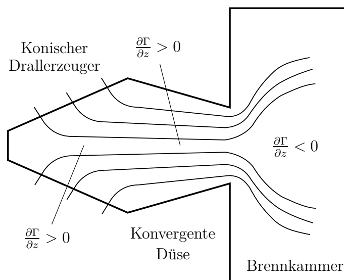
Abbildung 2.5: Schematische Darstellung der Stromlinien und entsprechendem axialen Gradient der Zirkulation des Drallerzeugerkonzepts A 2 EV
