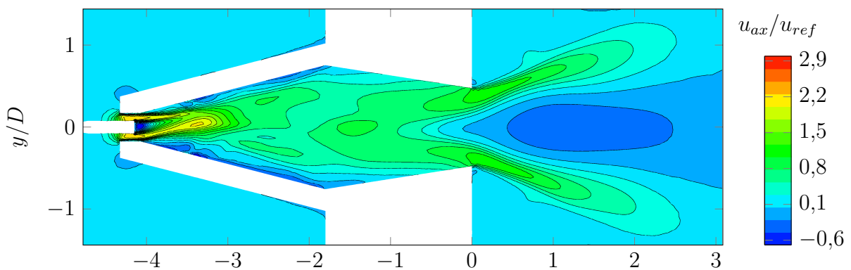
Abbildung 5.5: Asymmetrischer Zentralwirbel im Axialgeschwindigkeitsfeld des A 2 EV-Brenners mit zwei Schlitzten, Variante drei (Nr. 3 in Tabelle 1.1)
