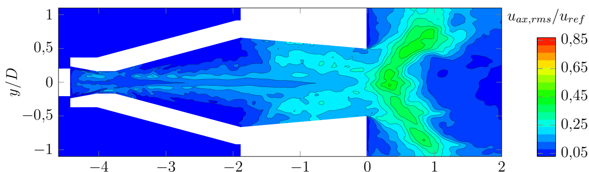
Abbildung 5.34: RMS der Axialgeschwindigkeit des A 2 EV-Brenners mit abgerundeten Schlitten
