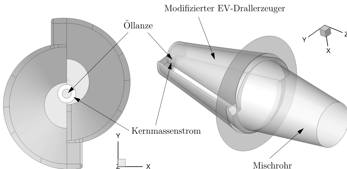
Abbildung 4.4: EV-Brenner mit Mischrohr (Nr. 1 in Tabelle 1.1) im Schnitt (links) und als halb transparentes Modell (rechts)
