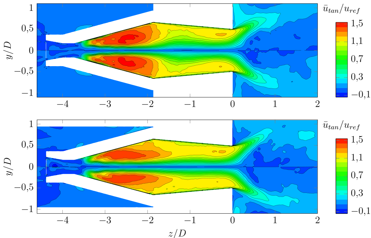
Abbildung 5.40: Mittleres Tangentialgeschwindigkeitsfeld des A 2 EV-Brenners mit großem (oben) und kleinem Plenum (unten)
