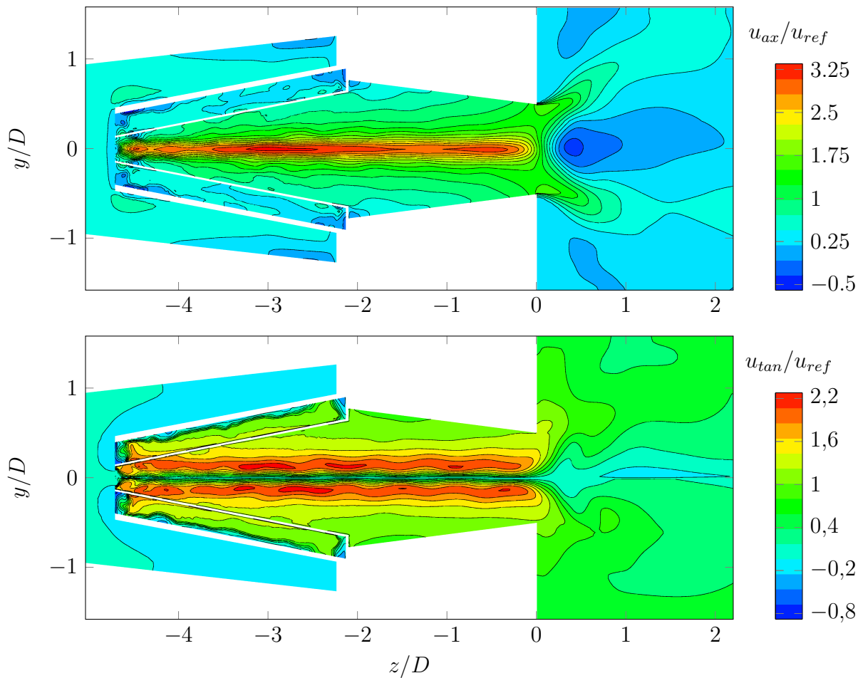
Abbildung 4.6: Normierte mittlere Axial- und Tangentialgeschwindigkeit mit 1% Kernströmung des modifizierten EV-Brenners
