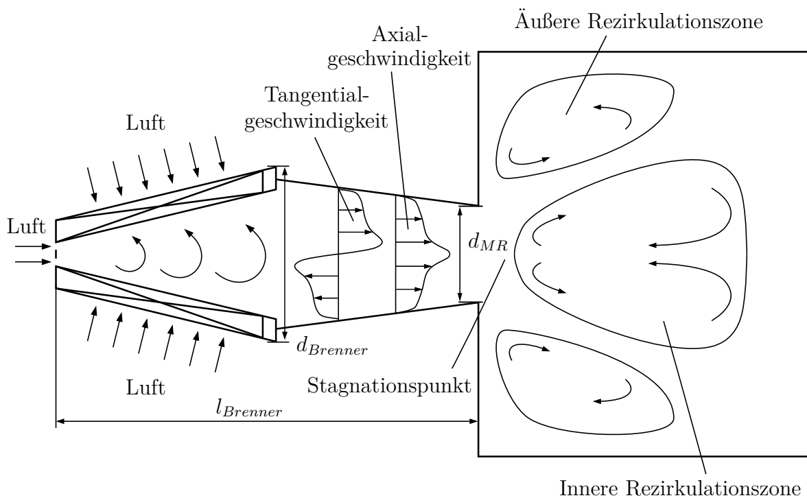
Abbildung 4.5: Prinzip des modifizierten EV-Brenners mit Mischrohr und wesentliche Charakteristika des Strömungsfelds
