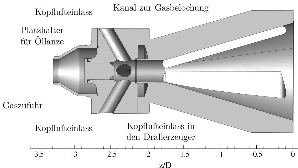
Abbildung 5.14: Prototyp im Schnitt
