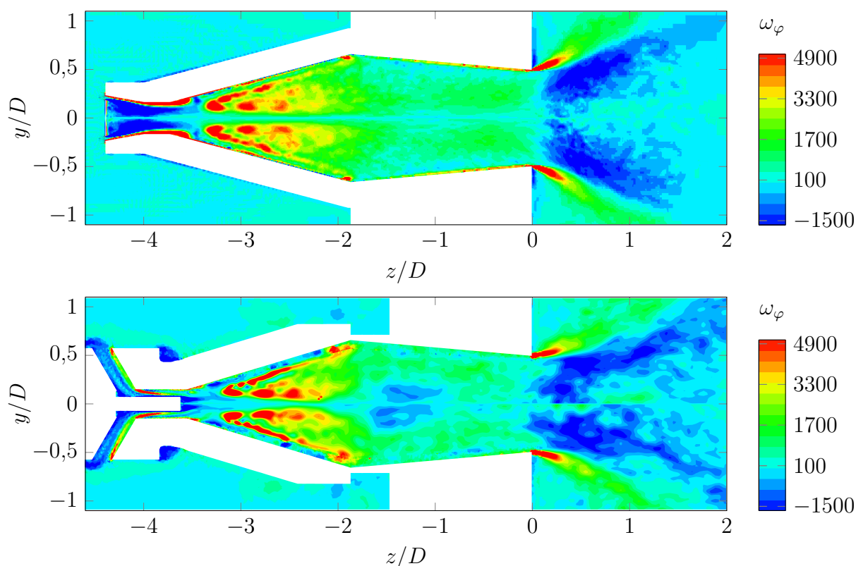
Abbildung 5.25: Azimutale Wirbelstärke des A 2 EV-Brenners (oben) und des Prototypbrenners (unten)
