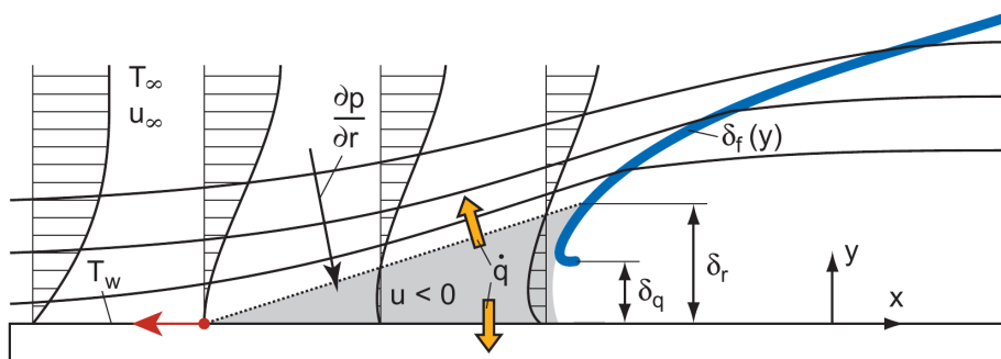
Abbildung 2.11: Schematische Darstellung des Flammenrückschlags durch die Wandgrenzschicht nach dem Modell von Eichler, [15]
