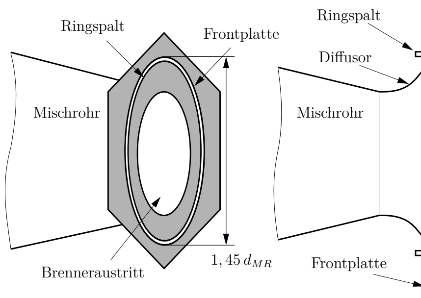
Abbildung 6.2: Ringspaltinjektor für die Kühlluftindüsung (links) und Diffusor (rechts)
