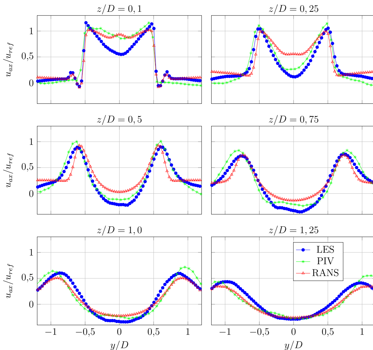
Abbildung 6.4: Profile der mittleren Axialgeschwindigkeit an verschiedenen axialen Positionen von LES, RANS und Experiment (PIV)
