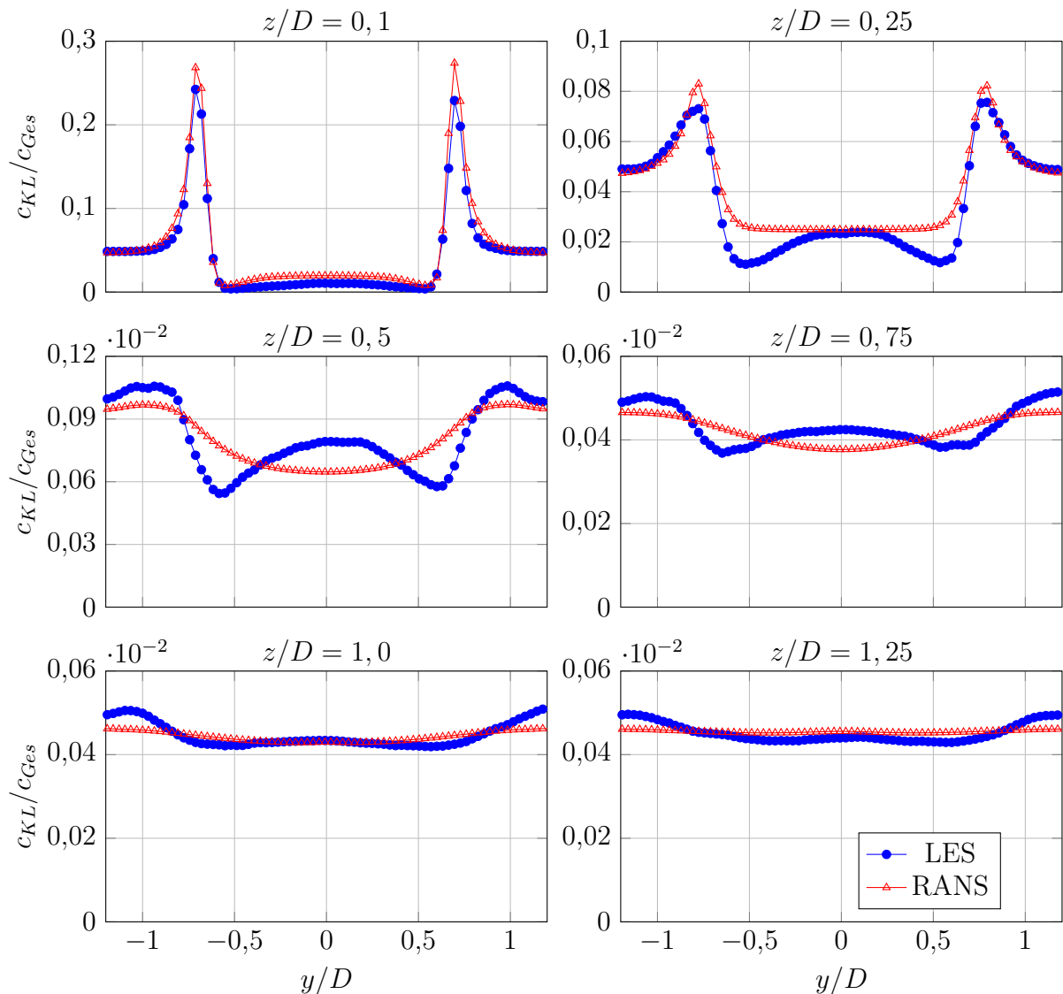
Abbildung 6.9: Profile der mittleren Kühlluftkonzentration an verschiedenen axialen Positionen von LES und RANS der Konfiguration mit Diffusor
