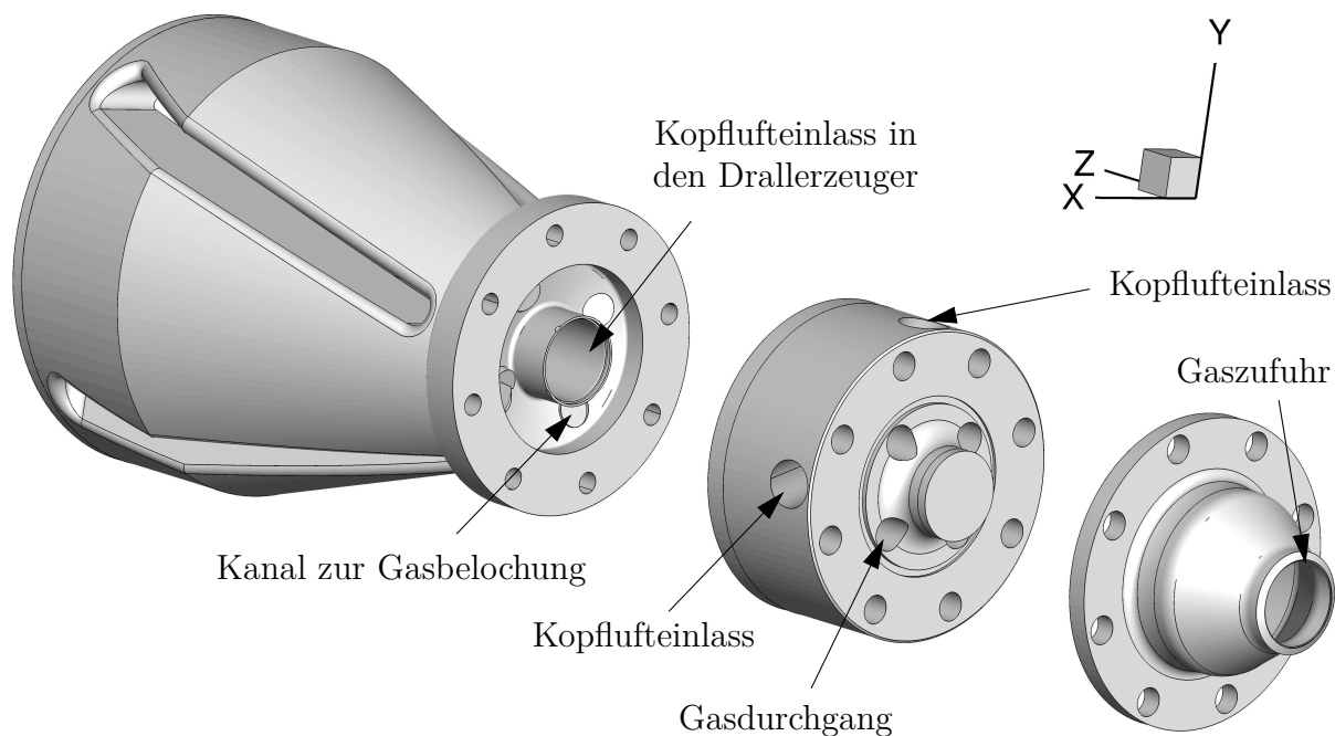
Abbildung 5.15: Prototyp mit Komponenten in Explosionsansicht
