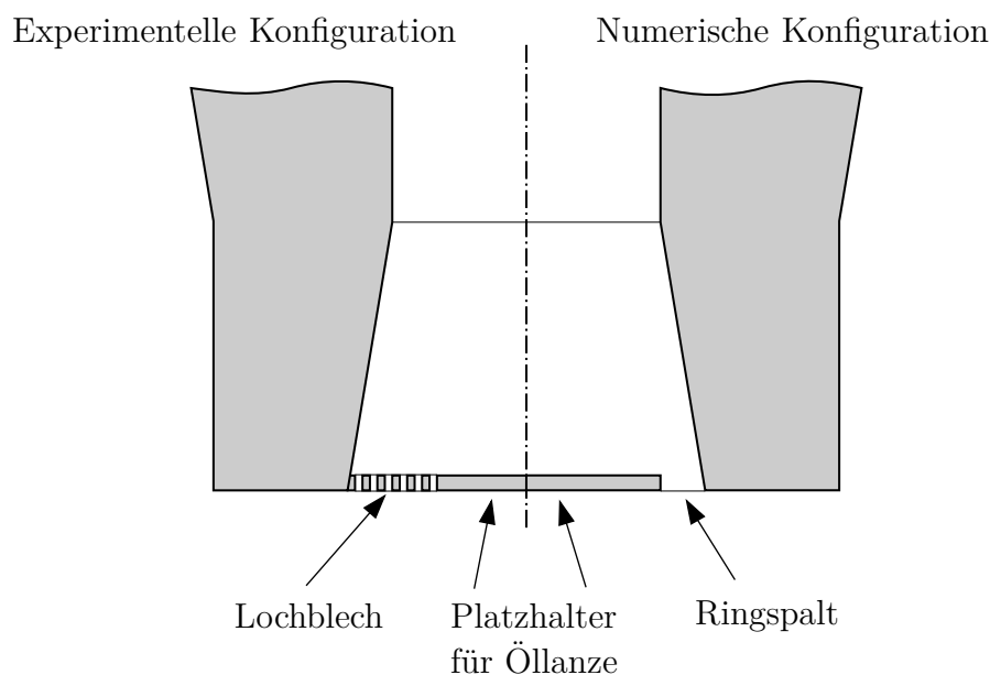
Abbildung 5.11: Halbschnitte der experimentellen (links) und numerischen (rechts) Konfiguration des Kopfeinlasses des A 2 EV-Brenners mit 4 Schlitzen
