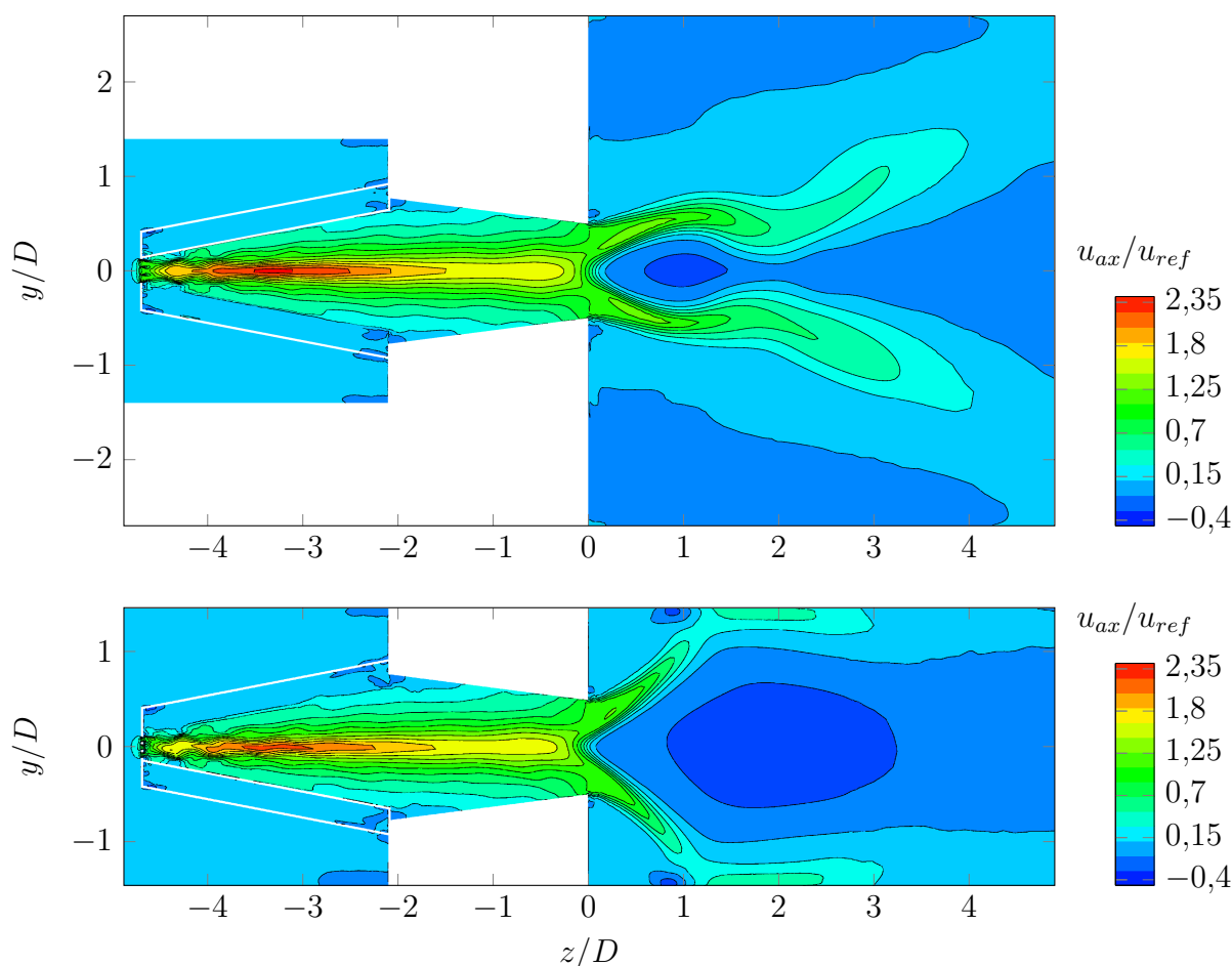
Abbildung 4.10: Axialgeschwindigkeitsfeld des modifizierten EV-Brenners in einer Brennkammer mit großem (oben) und kleinem (unten) Querschnittsprung
