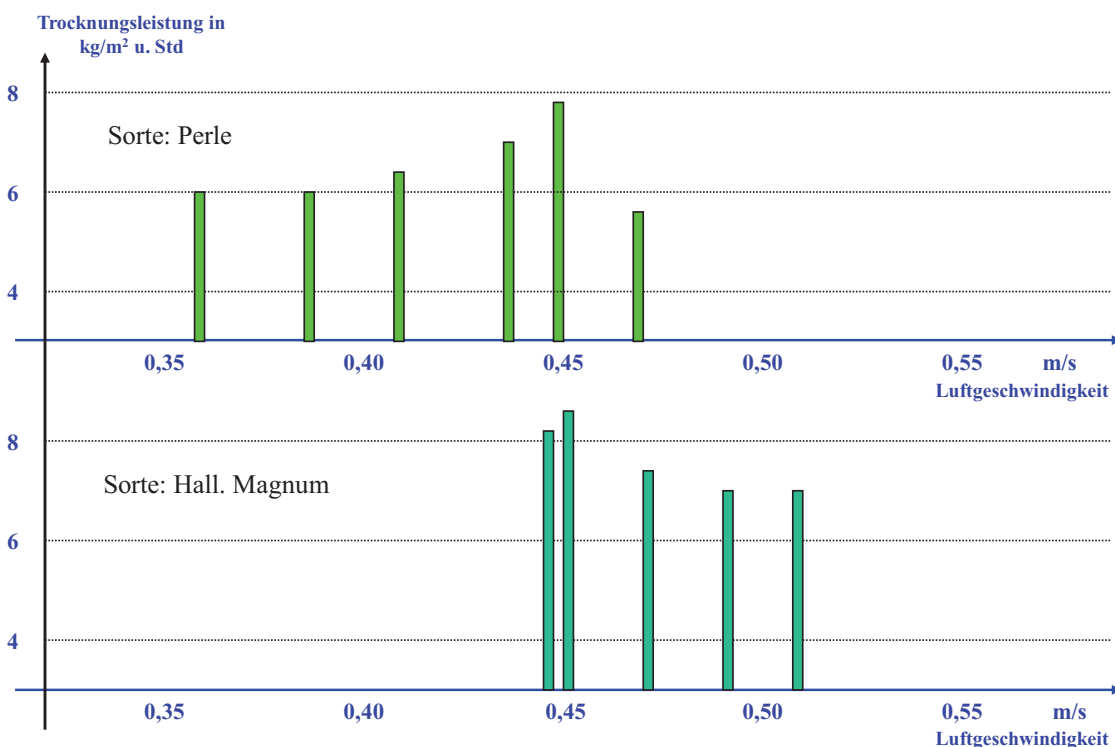
Trocknungsleistung bei Perle und Hall. Magnum in Abhängigkeit von der Luftgeschwindigkeit
