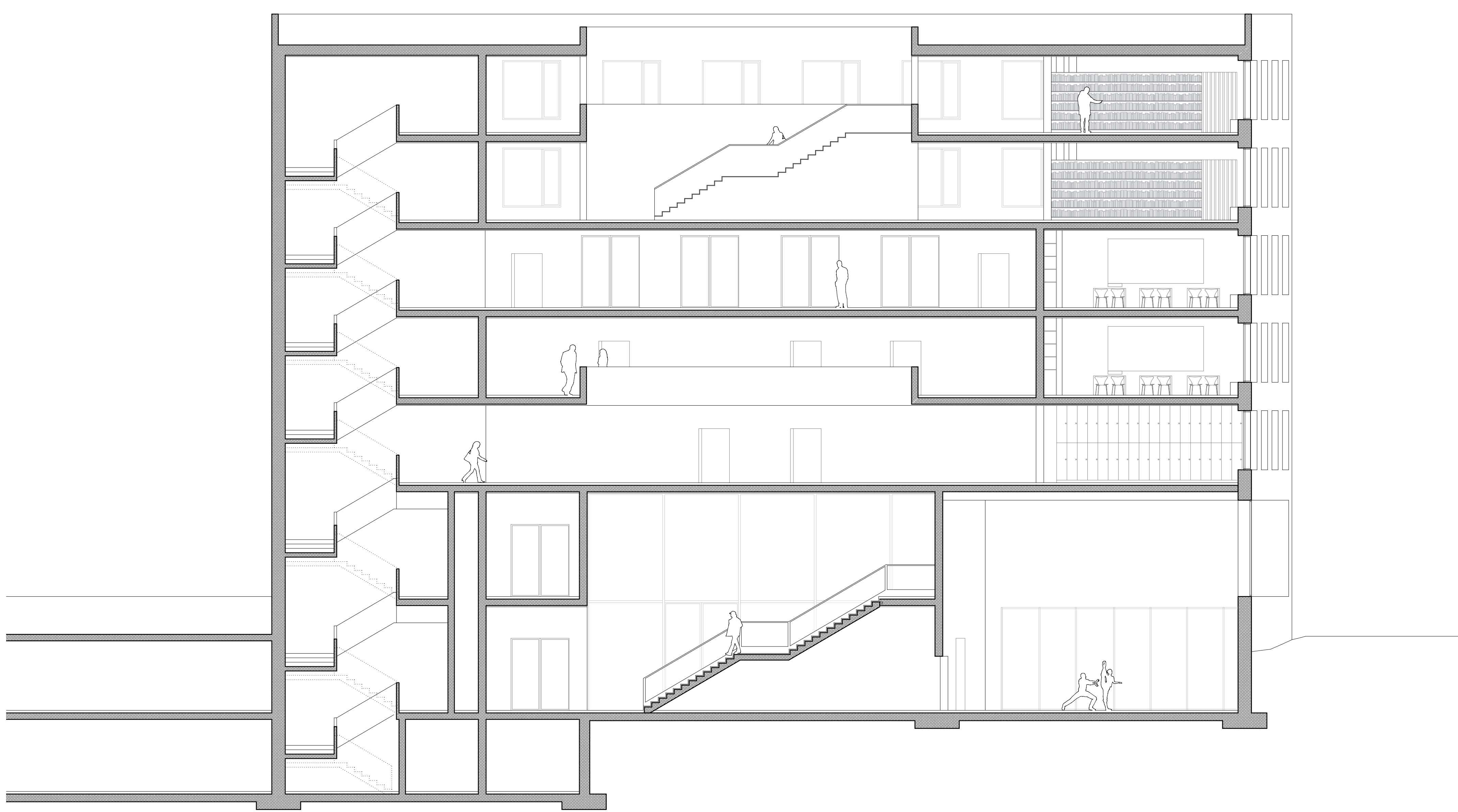
Schnitt BB 1:100
