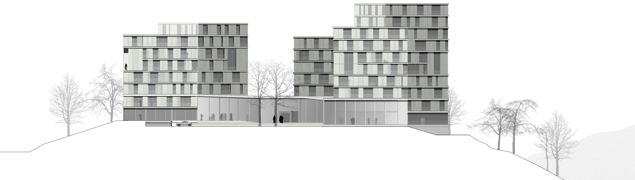
ANSICHT W
