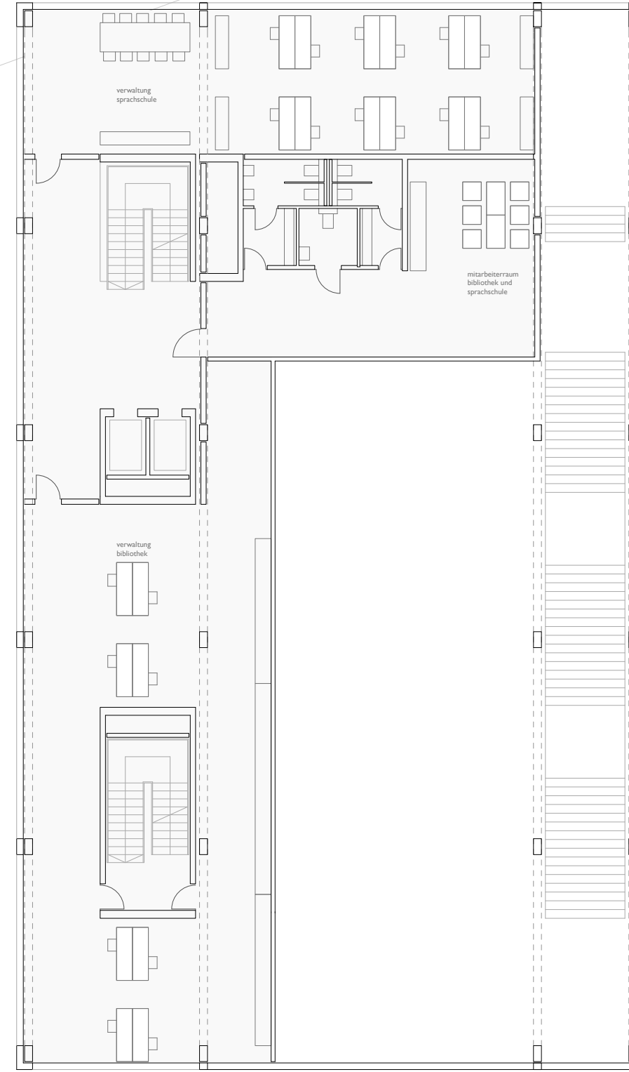
Grundriss Straßenebene Zwischengeschoss I_200
