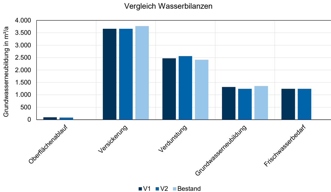
Abbildung 20 Vergleich der Wasserbilanzierungen für ein Kalenderjahr des Bestands und der Entwurfsvarianten V1a, V1b und V2
