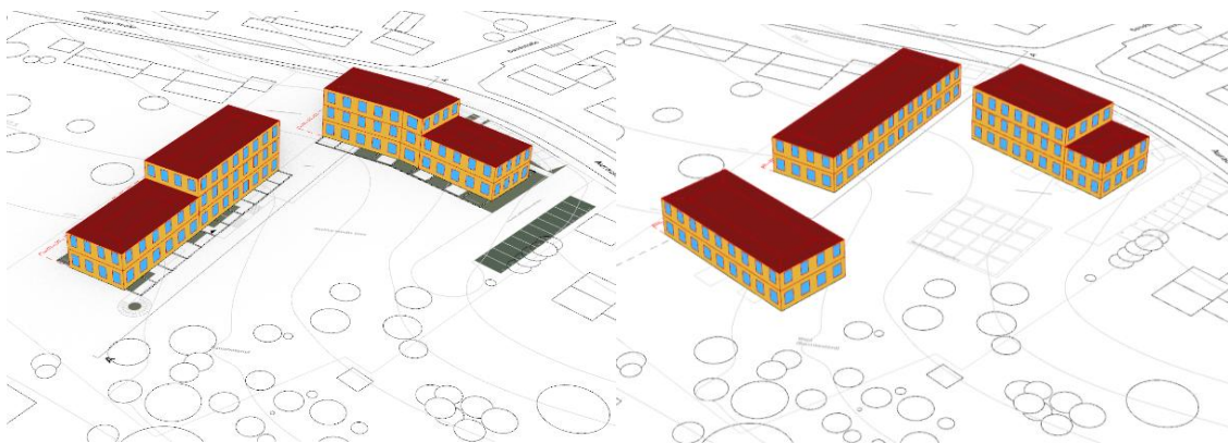
Abbildung 11 Darstellung der beiden Simulationsmodelle für die Varianten V1 (links) und V2 (rechts)
