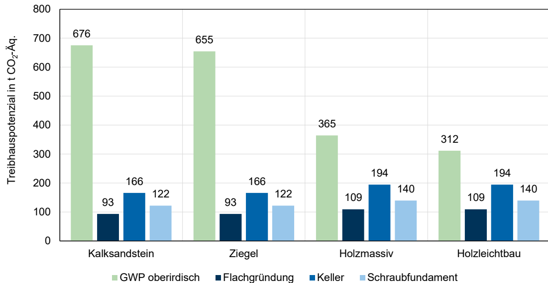
Abbildung 15 Treibhauspotenzial (GWP) für verschiedene Gründungsvarianten und Bauweisen, dargestellt für Entwurfsvariante V1
