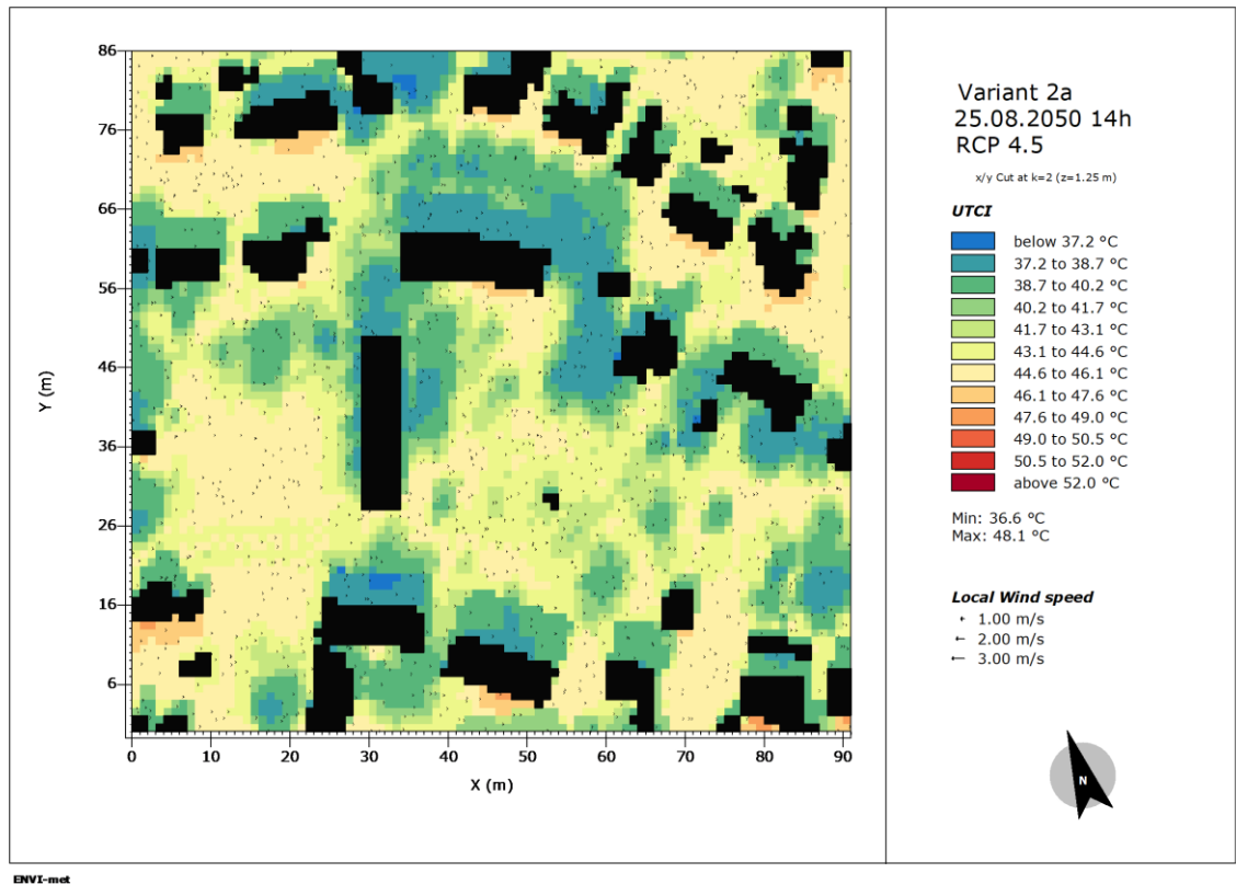
Abbildung 13 Darstellung einer ausgewählten Entwurfsvariante hinsichtlich den empfundenen Außenraumtemperaturen (UTCI) [Lüt24]
