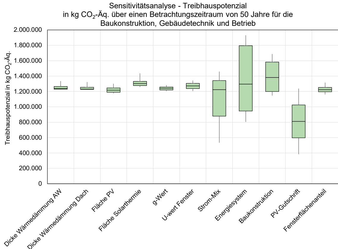
Abbildung 12 Sensitivitätsanalyse zu ausgewählten Gebäudeparametern und deren Einfluss auf das Treibhauspotenzial
