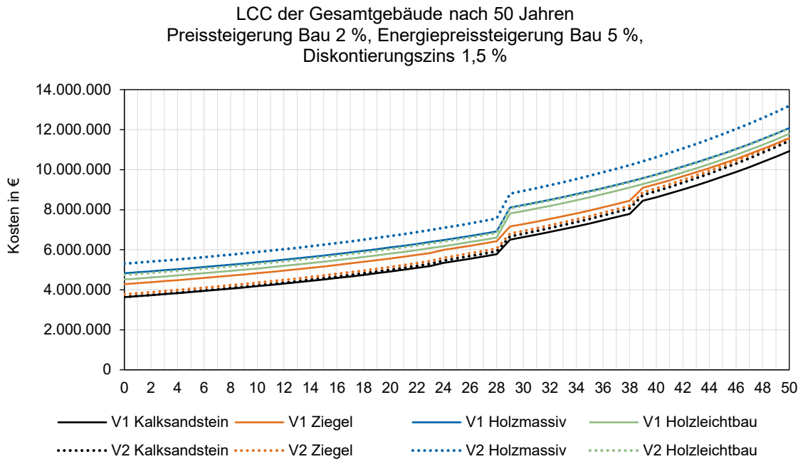
Abbildung 9 Vergleich der Lebenszykluskosten für die analysierten Entwurfsvarianten
