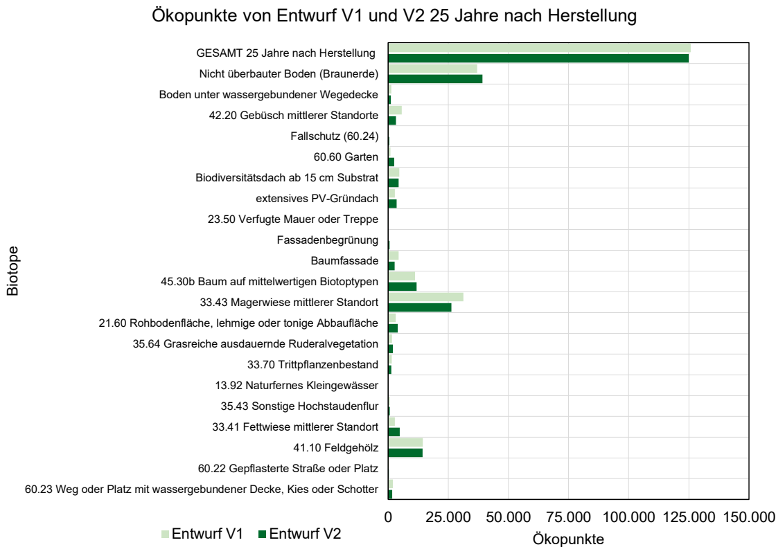
Abbildung 18 Vergleich von Fassadenbegrünungen mit Baumfassaden (Entwurf V1a) und Kletterpflanzen (Entwurf V1b) 25 Jahre nach Herstellung.
