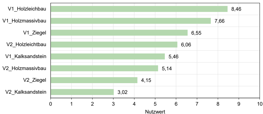
Abbildung 14 Nutzwerte der finalen Entwurfsvarianten V1 und V2
