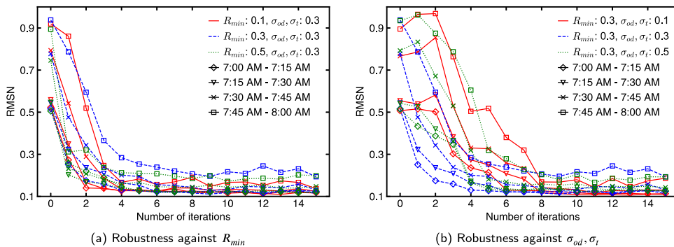
Fig. 18. Demand scenarios sensitivity (scenario: Red = 0.7, Rand = 0.3).
