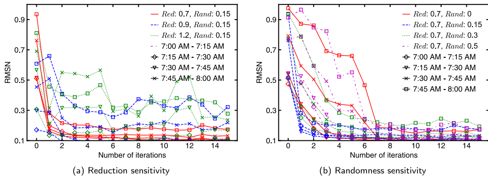
Fig. 14. Demand scenarios sensitivity (method 6).
