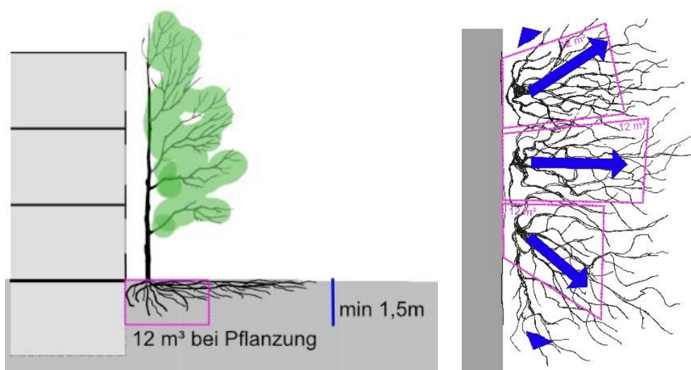
Abbildung 34: Schnitt - Wurzelentwicklung weg vom Gebäude (links); Aufsicht - Wurzelraumdimensionierung und -ausbreitung, unterirdisch, schematisch an einer Baumfassade mit 3 Bäumen (rechts) (Lisa Höpfl)
