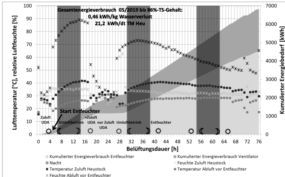
Abb. 1: Trocknungsverlauf und Energieverbrauch bei Entfeuchtereinsatz auf einem Praxisbetrieb 05/19
