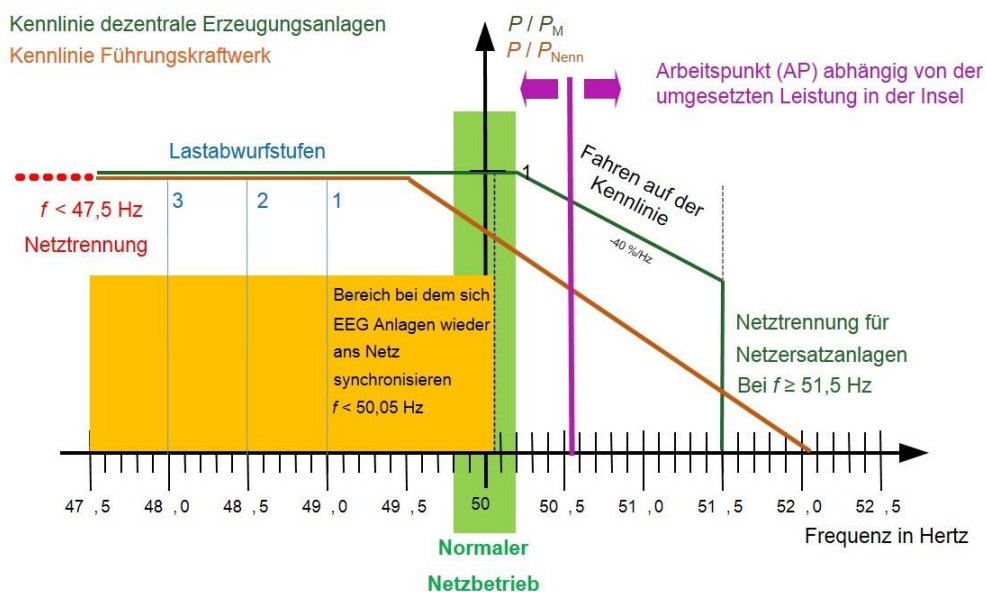
Abbildung 1: Regelungskonzept für Inselnetzbetrieb.
