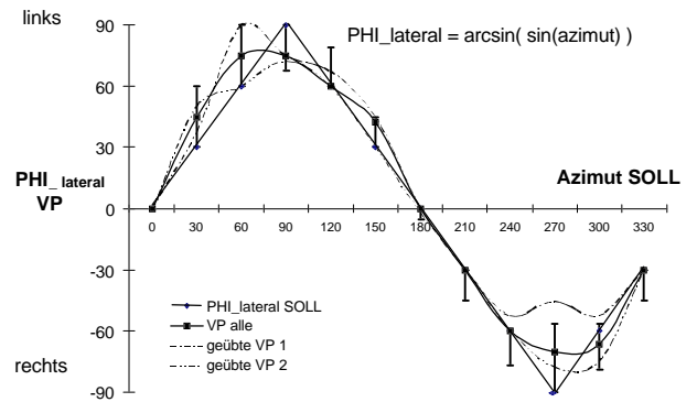
Abb. 6 : Maß für die seitliche Auslenkung
