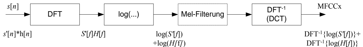
Abb. 3.16: Ablauf der Berechnung von MFCC-Koeffizienten
