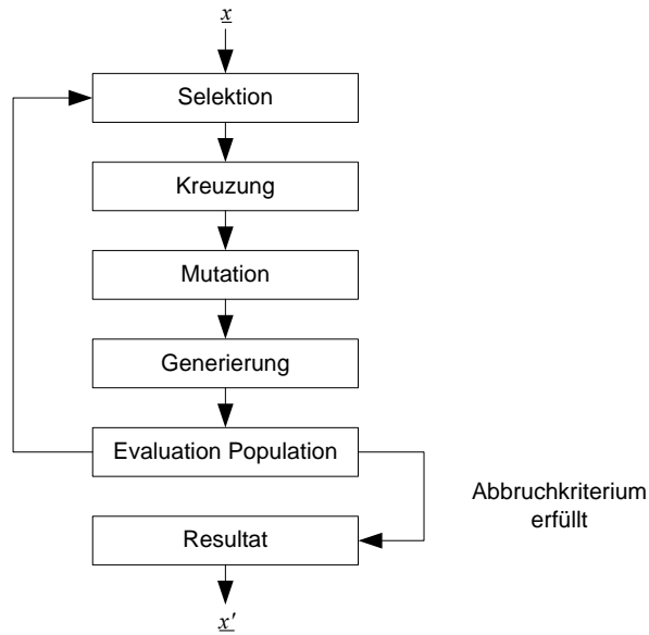
Abb. 3.32: Ablauf der hybriden Generierung und Selektion mit GA
