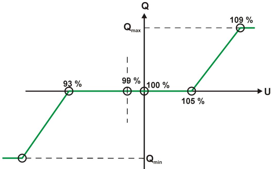
Abbildung 82: asymmetrische/verschobene Q(U)-Kennlinie
