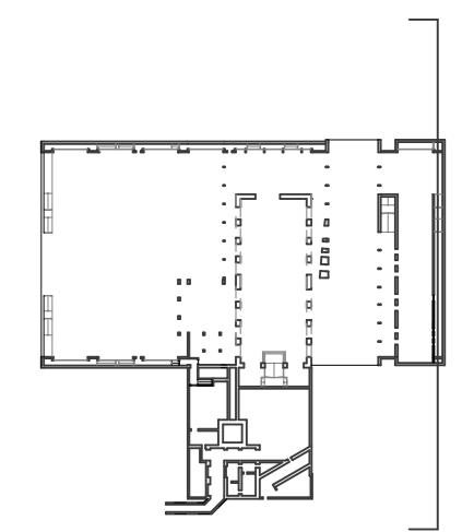
SCHNITT INSTITUTSGEBÄUDE HIMMELSTREPPE 1_200
