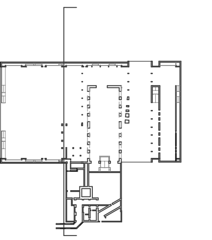
SCHNITT SITZSTUFEN AUSSTELLUNG 1_200
