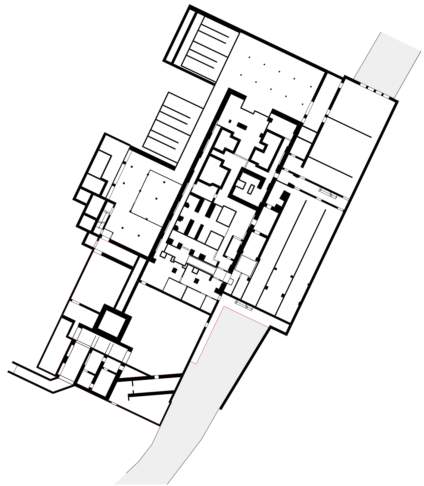
GRUNDRISS UNTERGESCHOSS BESTAND 1_500
