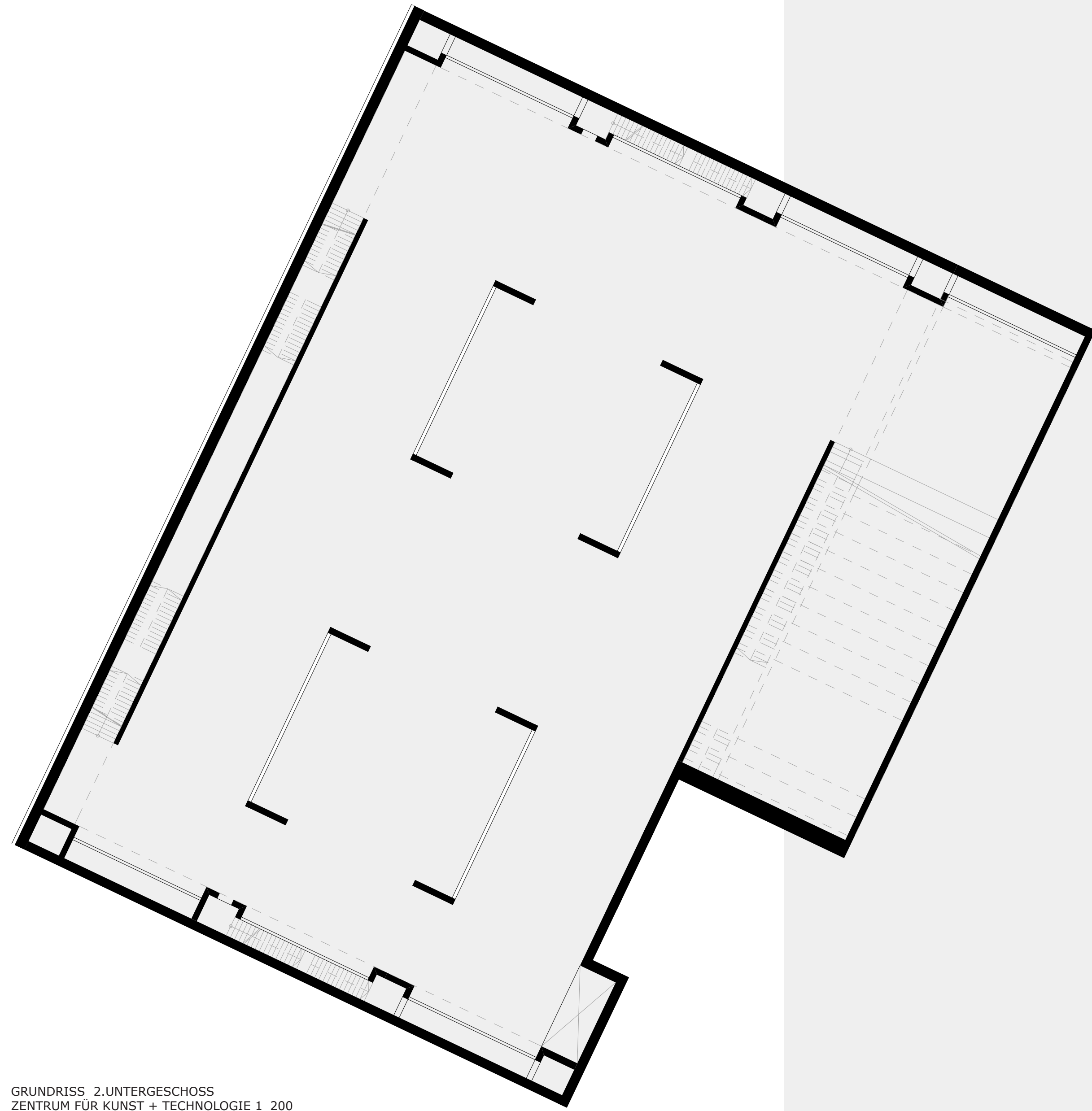
GRUNDRISS 2. UNTERGESCHOSS ZENTRUM FÜR KUNST + TECHNOLOGIE 1_200
