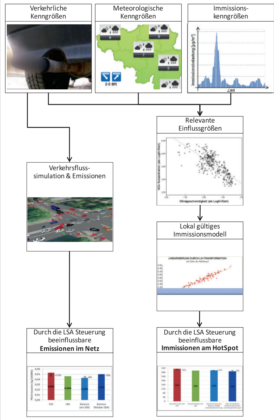
Bild 6: Bearbeitungsablauf für die Verarbeitung der Umweltkenngrößen
