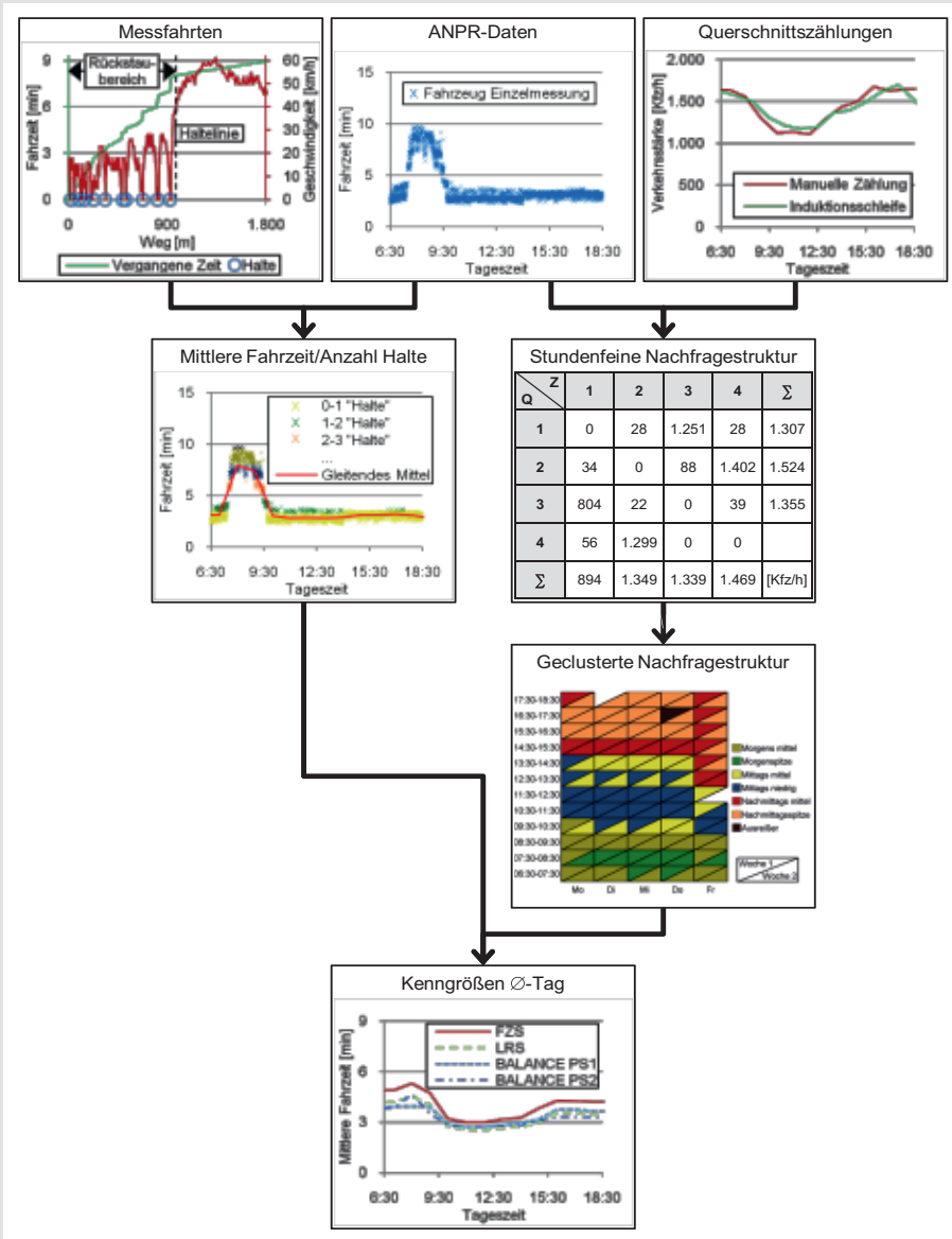
Bild 4: Bearbeitungsablauf für die Verarbeitung der verkehrlichen Kenngrößen
