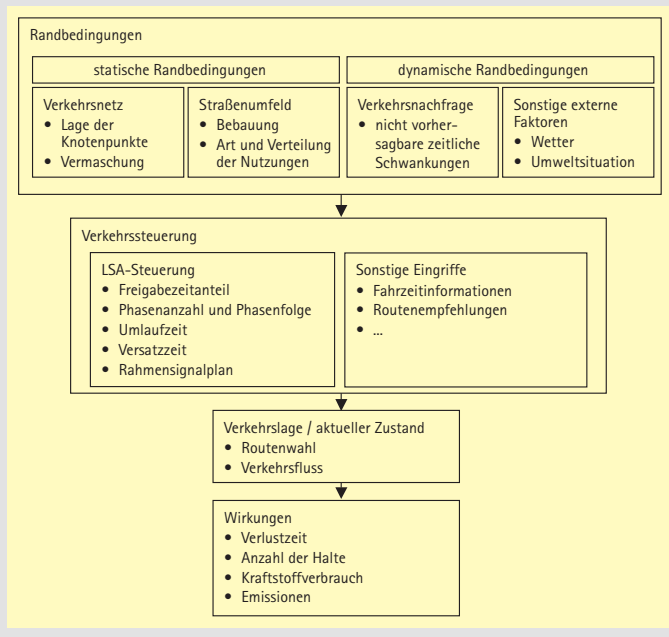
Bild 1: Wirkungszusammenhänge bei der Lichtsignalsteuerung
