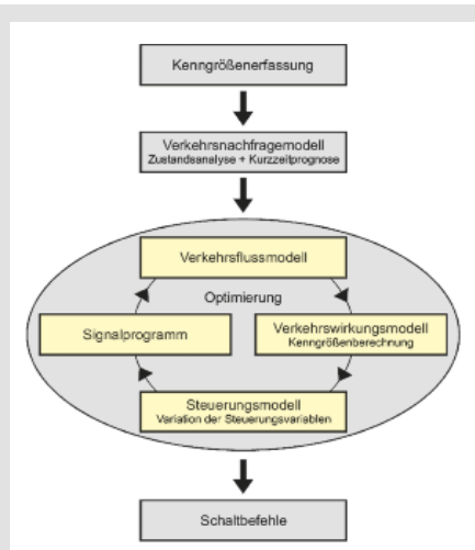
Bild 3: Modellbasierte Umsetzung eines Steuerungsverfahrens, nach RiLSA [FGSV 2010]
