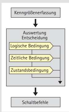
Bild 2: Regelbasierte Umsetzung eines Steuerungsverfahrens, nach RiLSA [FGSV 2010]
