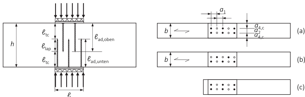
Abbildung 8: Querdrukverstärkungen zur Lastdurchleitung - Prüfkörperkonfiguration
