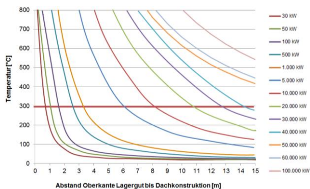
Abb. 5: kritische Plumetemperaturen in Abhängigkeit der Brandlast ohne Berücksichtigung der Heißgasschicht
