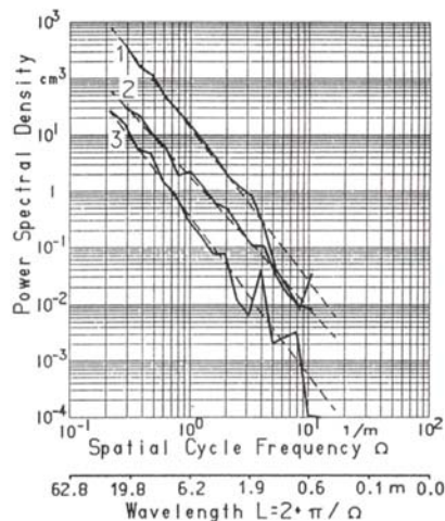
Abb. 8: Messprotokolle deutscher Fahrstraßen, doppeltlogarithmische Darstellung der spektralen Unebenheitsdichte [Schu-91]
