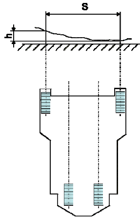
Abb. 2: Definition des maximalen Höhenunterschieds quer zur Fahrtrichtung ([DIN 15185], Bild 1)
