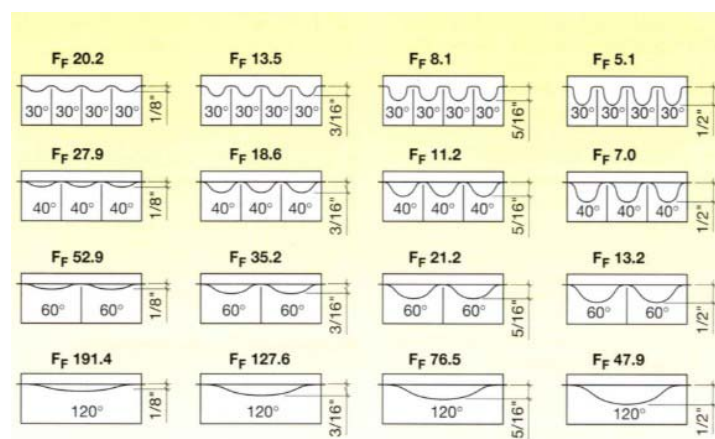
Abb. 3: Klassifikation von Bodenprofilen aufgrund der Welligkeit nach [ACI-117], [GüSc-05]
