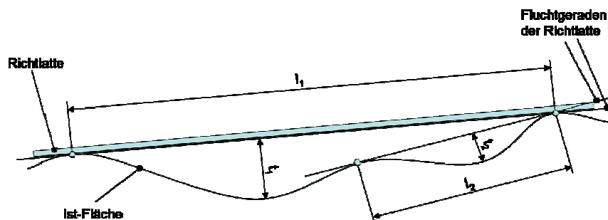
Abb. 1: Definition der Ebenheitstoleranz ([DIN-18202], Bild 6)
