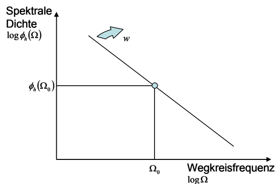
Abb. 7: Doppeltlogarithmische Darstellung der spektralen Dichte über die Wegkreisfrequenz
