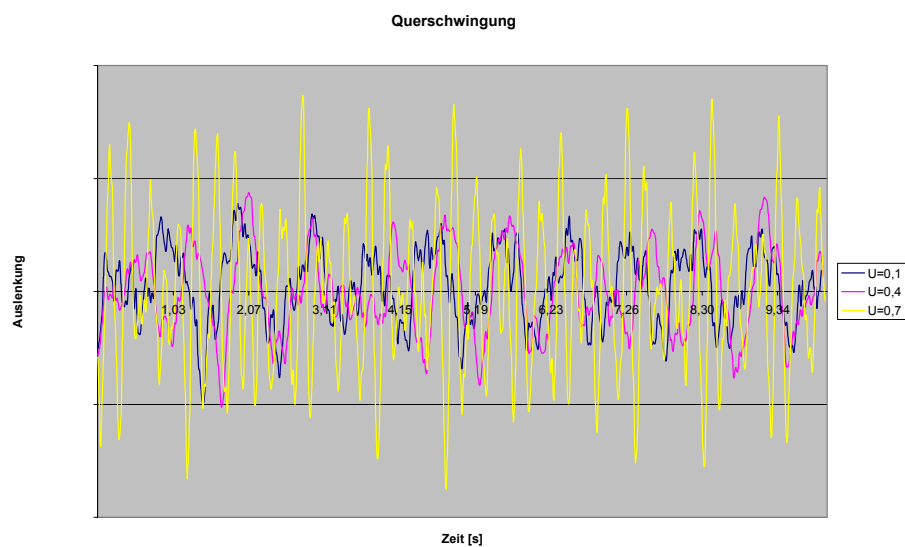
Abb. 10: Querschwingungsamplitude bei unterschiedlichen Böden (U=0,1, U=0,4, U=0,7)
