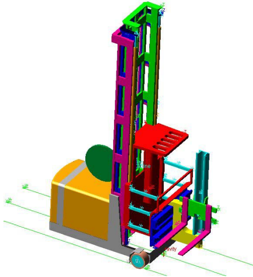
Abb. 4: Mehrkörpermodell eines Schmalgangstaplers
