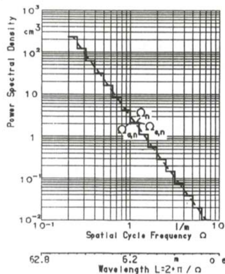
Abb. 9: Diskretisierung der spektralen Dichte [Schu-91]
