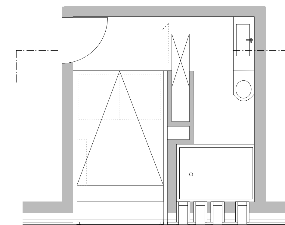
ZIMMERGRUNDRISS M 1 | 50
