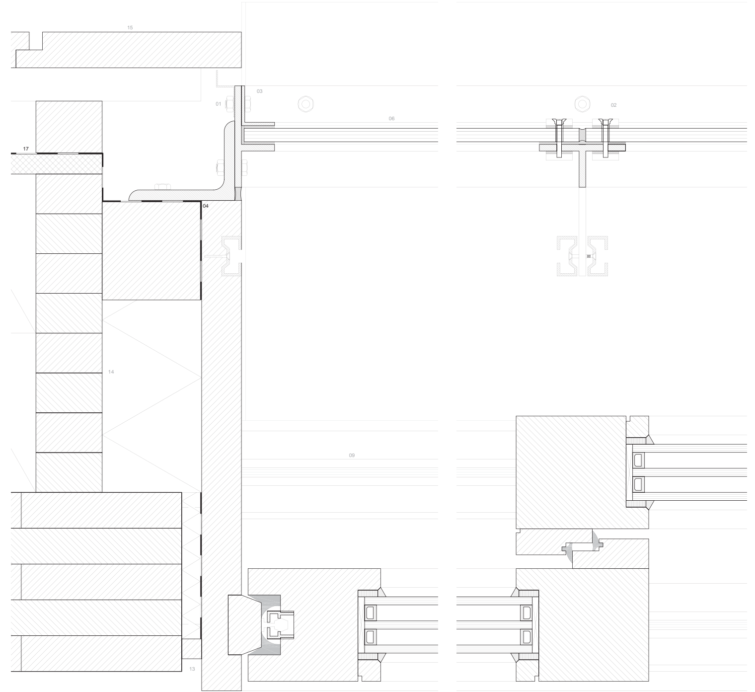
Grundriss M 1:1
