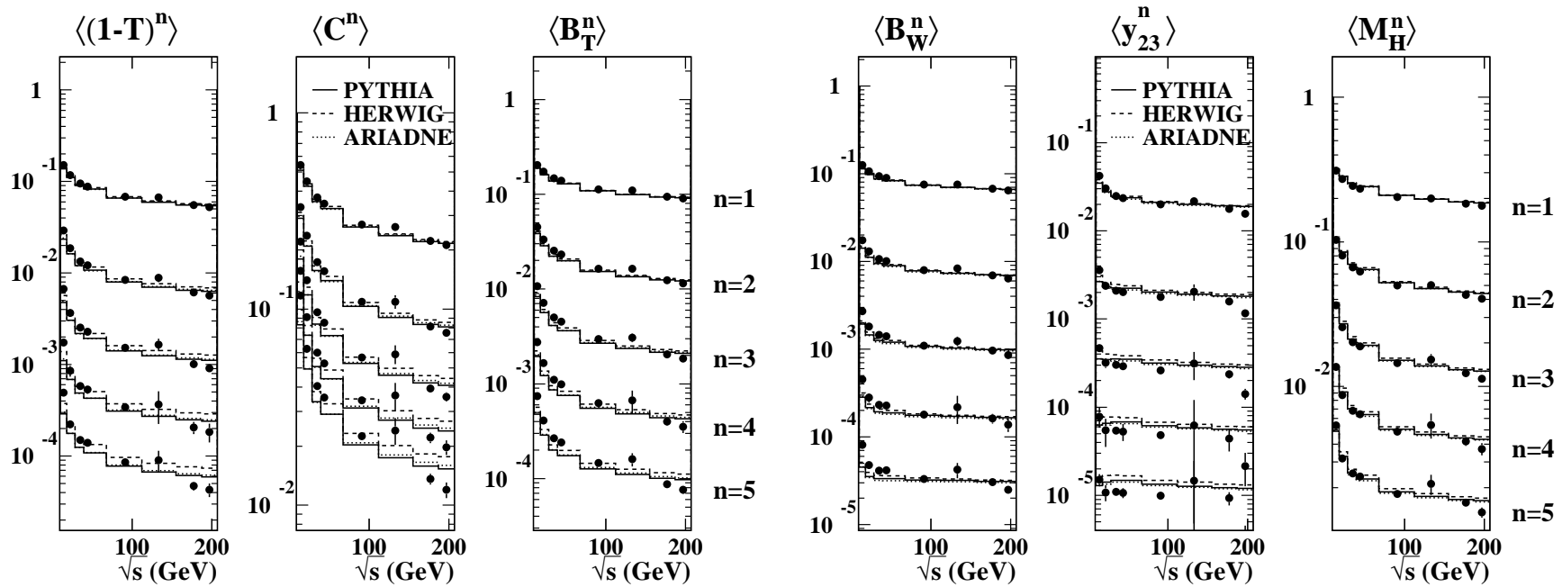
Abbildung A.1: Momente von Thrust, \langle(1-T)^n\rangle , C -Parameter, \langle C^n\rangle , Total Jet Broadening, \langle B_T^n\rangle , Wide Jet Broadening, \langle B_W^n\rangle , Durham Zweijet-Flipparameter, \langle y_{23}^n\rangle , und Heavy Jet Mass, \langle M_H^n\rangle , für n = 1 \dots 5 auf Detektorniveau an acht repräsentativen Energiepunkten – 14.0 GeV, 22.0 GeV, 35.0 GeV, 43.8 GeV, 91.3 GeV (Jahr 2000), 130.3 GeV, 188.6 GeV und 206.6 GeV. Die Fehlerbalken zeigen die statistischen Fehler. Die Vorhersagen des Monte Carlo Modells PYTHIA, HERWIG und ARIADNE sind – wie beschrieben im Text – mit Linien überlagert.
