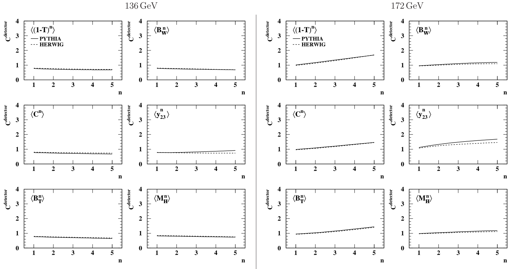
Abbildung 4.9: Detektorkorrekturen bei \sqrt{s} = 136 \text{ GeV} und \sqrt{s} = 172 \text{ GeV} , berechnet mittels PYTHIA und HERWIG.
