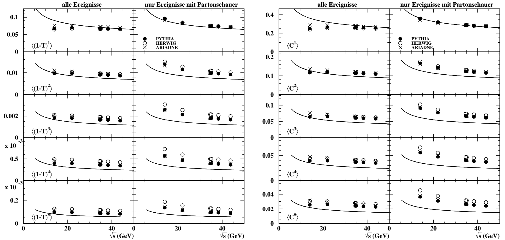
Abbildung D.1: Vorhersagen der Monte Carlo Modelle PYTHIA, HERWIG und ARIADNE für die Momente von Thrust, \langle(1-T)^n\rangle , und C -Parameter, \langle C^n\rangle , für n = 1 \dots 5 auf Partonniveau an vier JADE-Energiepunkten – 14.0 GeV, 22.0 GeV, 35.0 GeV und 43.8 GeV. Verwendet werden alle Ereignisse, oder nur die Ereignisse mit Partonschauer. Die Linie zeigt die NLO-Vorhersage mit zugrundegelegtem Wert von \alpha_s(M_{Z^0}) = 0.12 .
