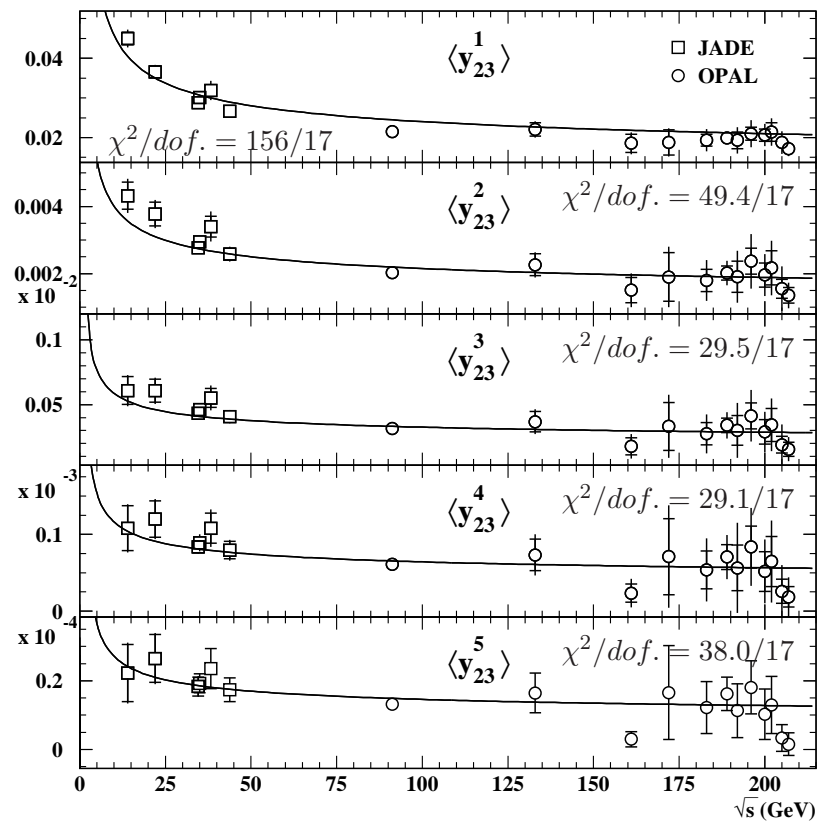
Abbildung 5.15: Fits der NLO-Vorhersage an JADE- und OPAL-Messungen von Momenten des Durham Zweijet-Flipparameters sowie der Heavy Jet Mass. Eingezeichnet sind die im Fit verwendeten statistischen Fehler (innere Balken) sowie Gesamtfehler inklusive der experimentellen Systematik. Die durchgezogene Linie gibt die mit der Schwerpunktsenergie laufende NLO-Vorhersage wieder mit dem angepassten Wert ihres Parameters \alpha_s(M_{Z0}) .
