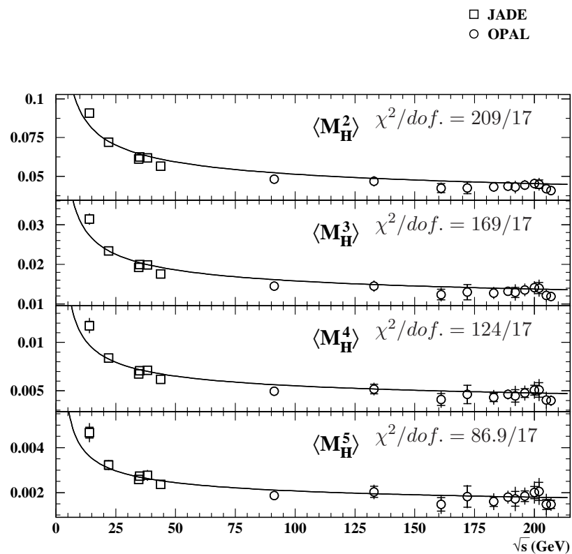
Abbildung 5.15: Fits der NLO-Vorhersage an JADE- und OPAL-Messungen von Momenten des Durham Zweijet-Flipparameters sowie der Heavy Jet Mass. Eingezeichnet sind die im Fit verwendeten statistischen Fehler (innere Balken) sowie Gesamtfehler inklusive der experimentellen Systematik. Die durchgezogene Linie gibt die mit der Schwerpunktsenergie laufende NLO-Vorhersage wieder mit dem angepassten Wert ihres Parameters \alpha_s(M_{Z0}) .
