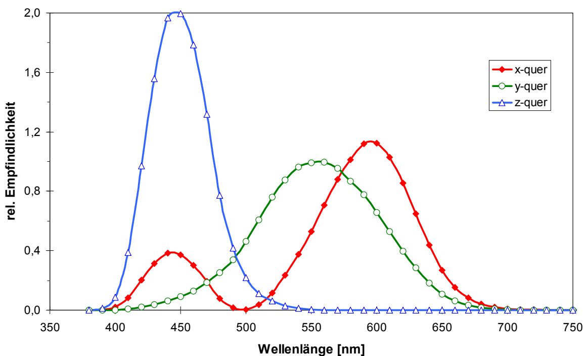
Abbildung 4: Normspektralwerte nach CIE; 10^\circ Normalbeobachter
