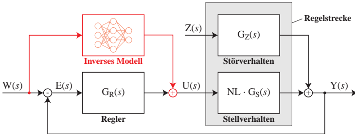
Abbildung 2.6: Geschlossener Regelkreis mit nichtlinearem Stellverhalten NL \cdot G_S(s) und einem inversen Prozeßmodell als Vorsteuerung zur Unterstützung eines konventionellen Reglers.
