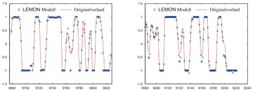
Abbildung 6.7: Ausschnitte aus den Vorhersagen der LEMON-Hysterese-Modelle mit der Trainingstrajektorie als Eingabe. Links ist das Modell mit verschiedenen lokalen Modell-Prototypen gezeigt. Rechts das Modell mit RBF-Netzen. Es wurde jeweils der beste Ausschnitt gewählt.
