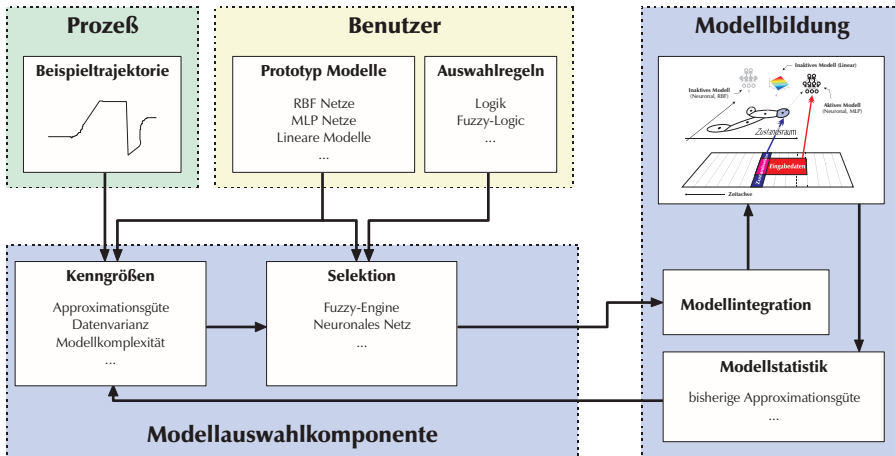
Abbildung 5.14: Kombination von ellipsoiden Karten und lokaler Modellbildung mit Benutzer-gesteuerter Modellauswahl.
