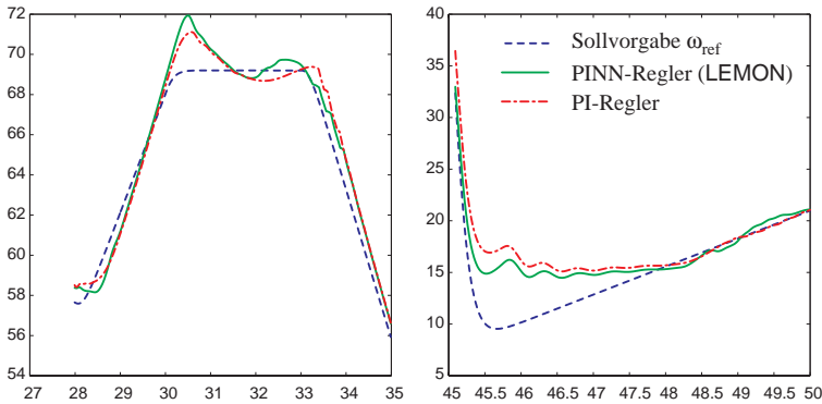
Abbildung 6.12: Ergebnis einer Prüfstandsimulation mit PINN-Regler und LEMON.
