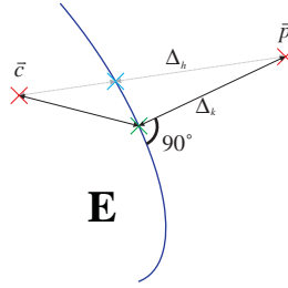
Abbildung 5.3: Näherung des Lotabstandes \Delta_k auf die Ellipsoidoberfläche durch \Delta_h , den Abstand zum Schnittpunkt der Verbindungslinie zum Zentrum.
