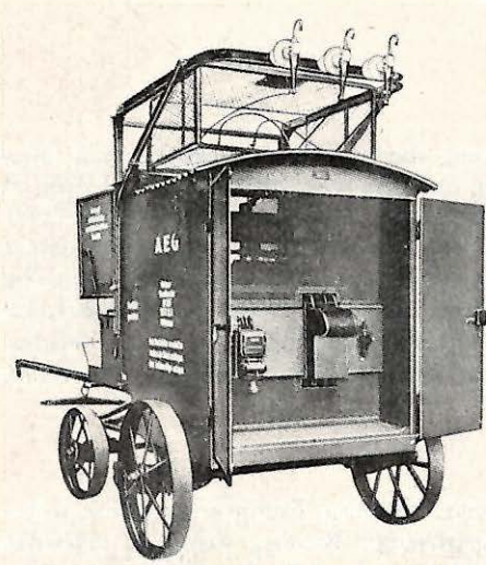
Abb. 2: Transformatorwagen mit niedergelegtem Mast 1930
