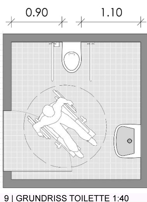
9 | GRUNDRISS TOILETTE 1:40
