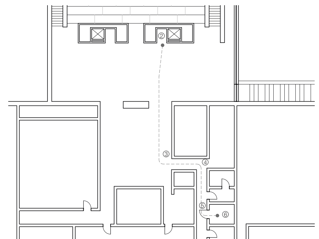
Grundriss UG 1:250
