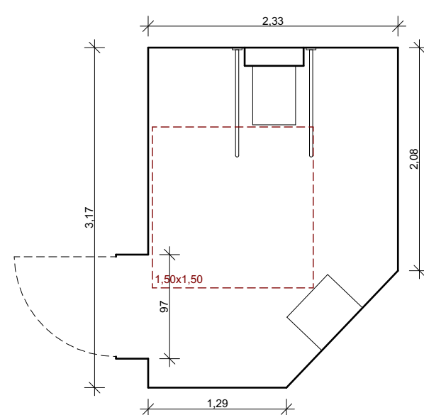
Grundriss WC - M: 1.50
