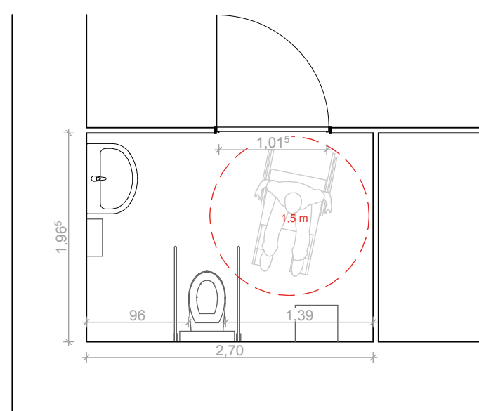
Grundriss Behinderten - WC 1:50
