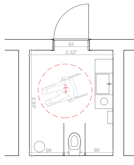
Grundriss Behinderten - WC 1:50
