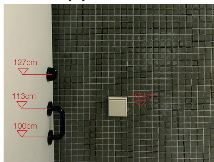
9 Lichtschalter und Türgriff
