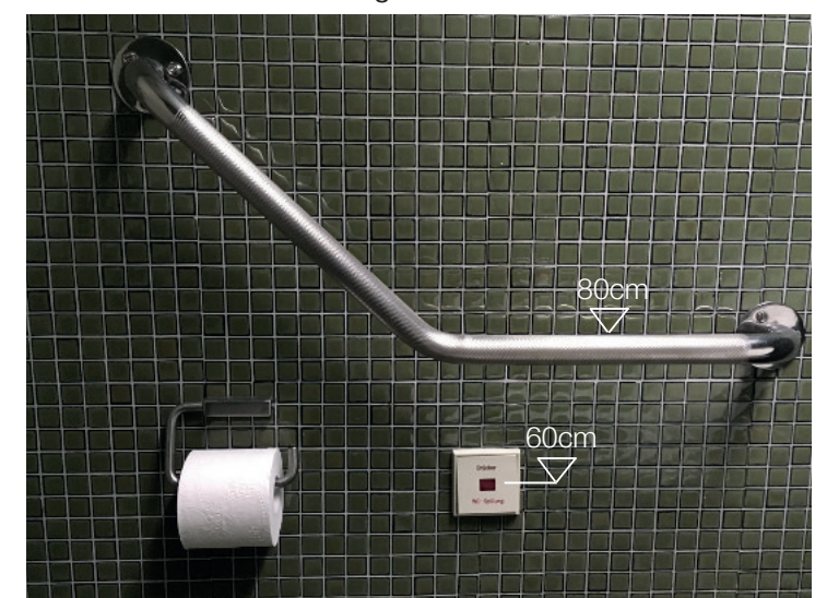
10 Stützgriff und WC-Drückerplatte
