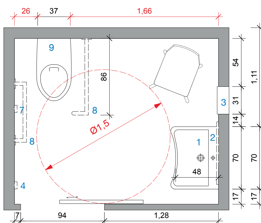
11 Grundriss 1:25
