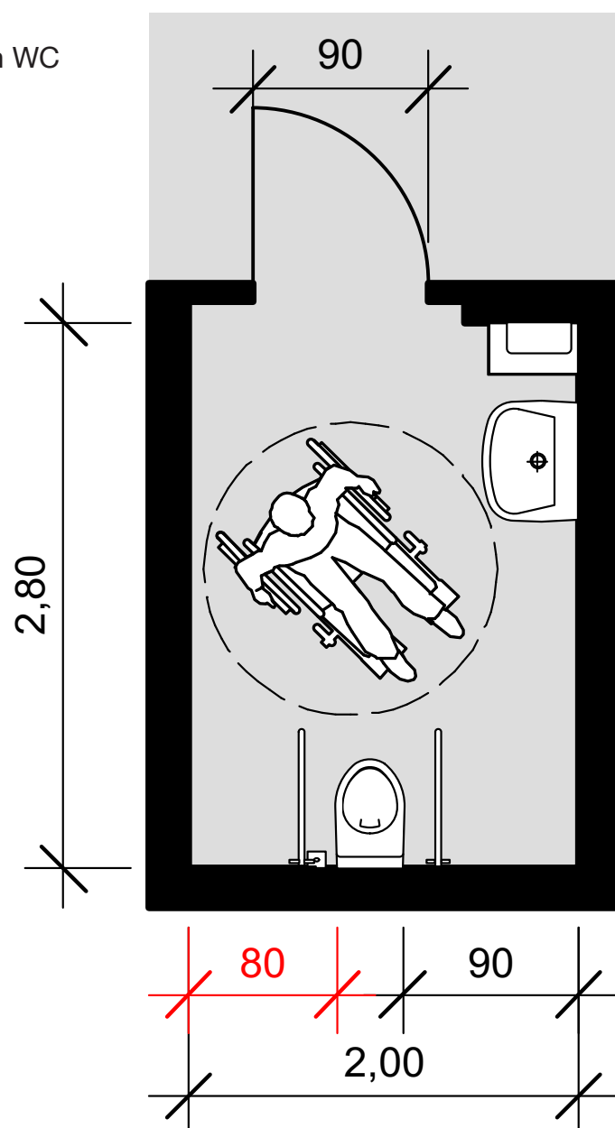
Grundriss EG
