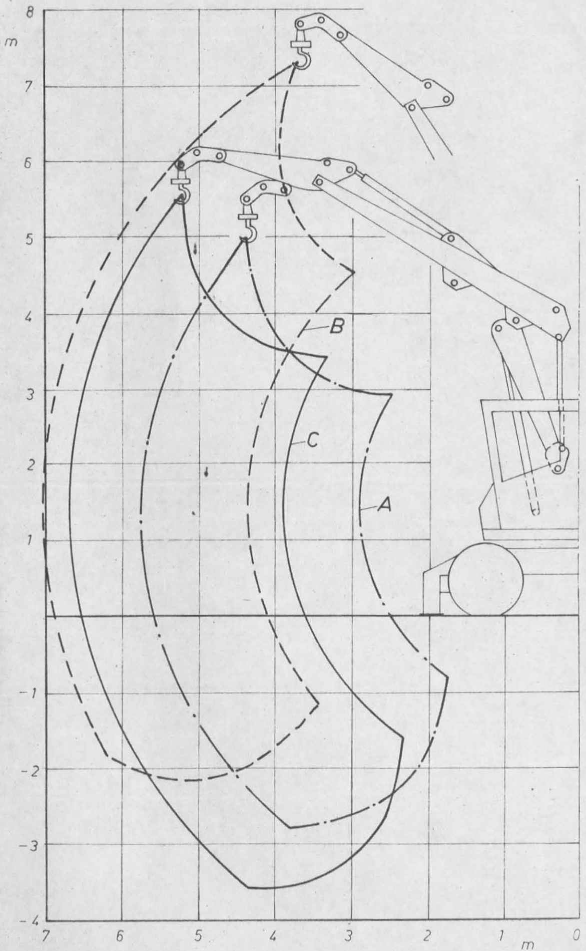
Bild 1 Reichweitendiagramm T 185
