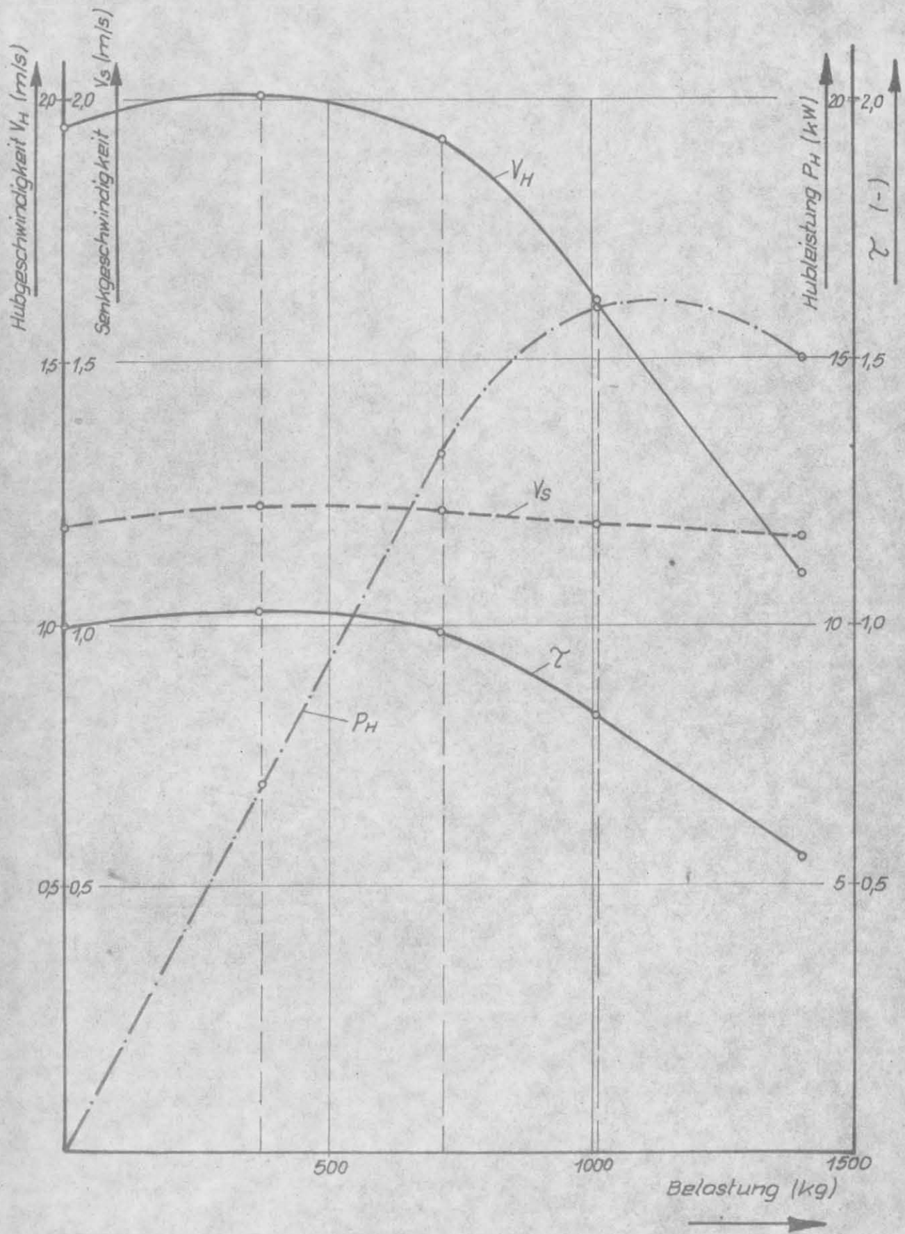
Bild 3: Hubcharakteristik T 185 (Montagevariante 110A)
