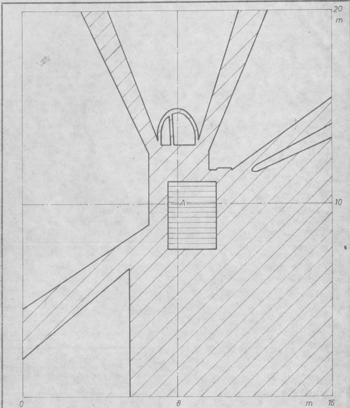
Sichtverhältnisse nach TGL 24626/14
