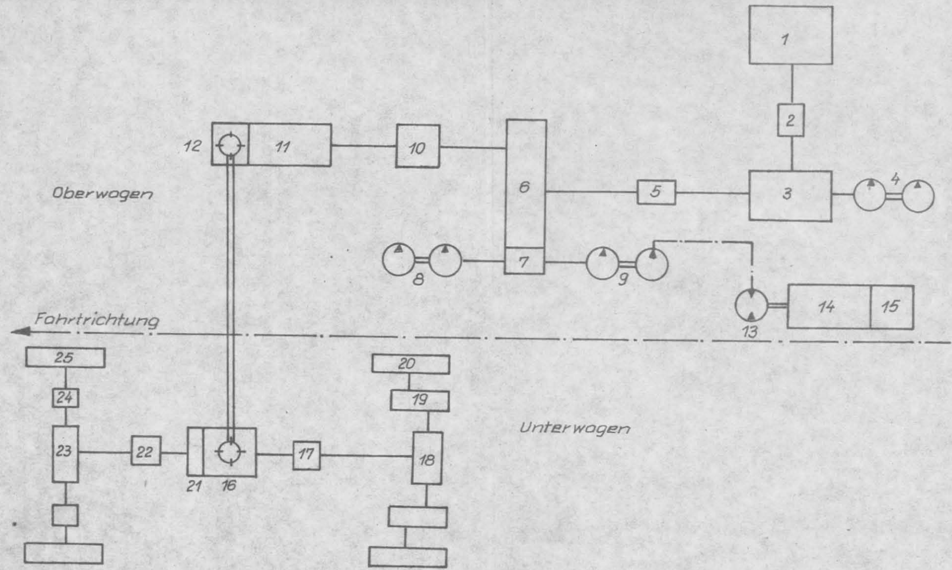
Bild 2: Antriebschema T 185
