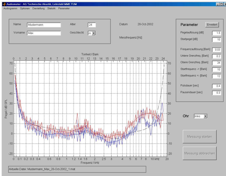
Abb. 2: Graphische Oberfläche der Steuerungssoftware des Audiometers. Neben der Eingabemöglichkeit für die Versuchspersonendaten (links oben) befinden sich rechts Einstellmöglichkeiten für die Meßparameter. In den darunter liegenden Feldern kann das zu messende Ohr ausgewählt und die Messung gestartet werden. Zentral sichtbar ist die Meßkurve, die fortschreitend aktualisiert wird. Nach erfolgter Messung kann die Mittelwertkurve berechnet und angezeigt werden. Die mittlere Ruhehörschwelle nach Terhardt [2] kann eingeblendet werden.
