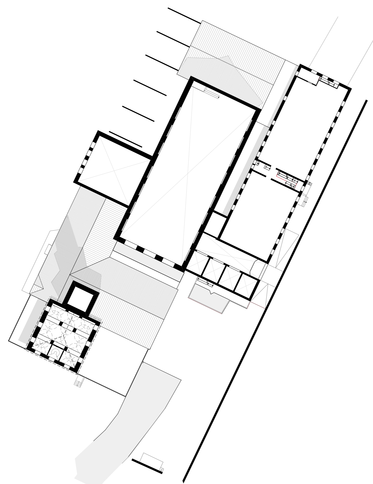
GRUNDRISS 1.OBERGESCHOSS BESTAND 1_500
