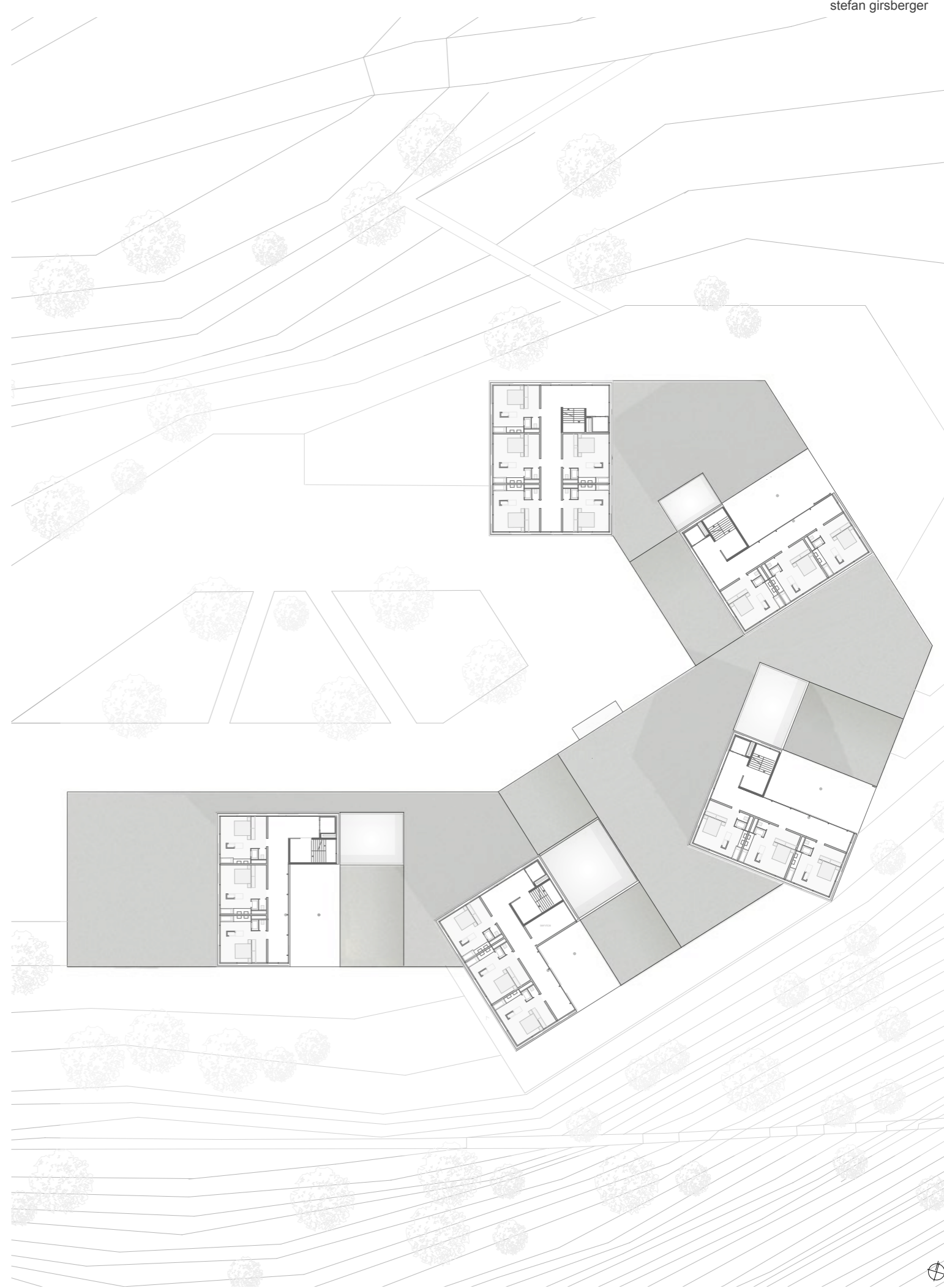
GRUNDRISS OG2 1:200
