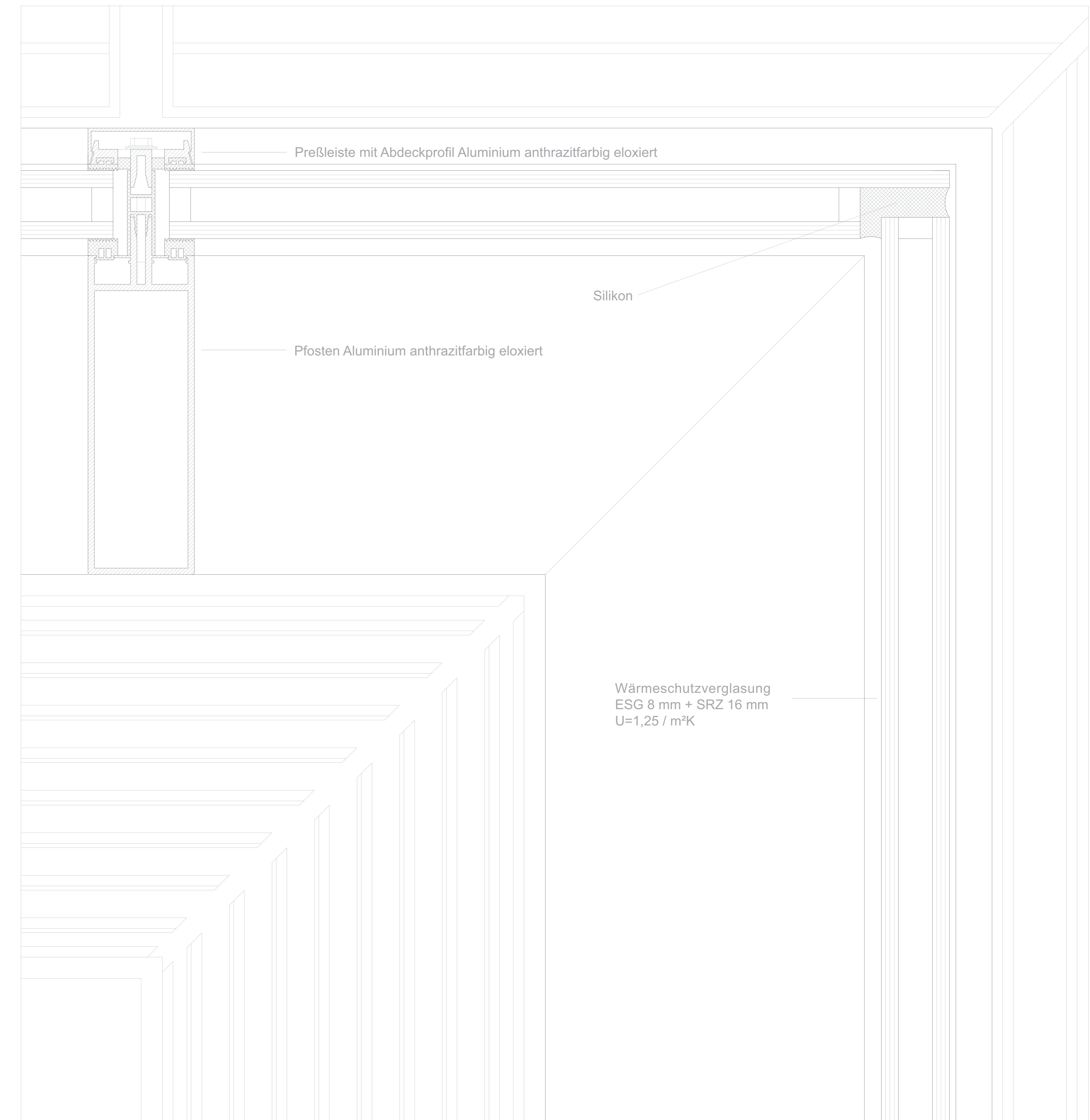
Detail M 1:1 Ecke Fassade West
