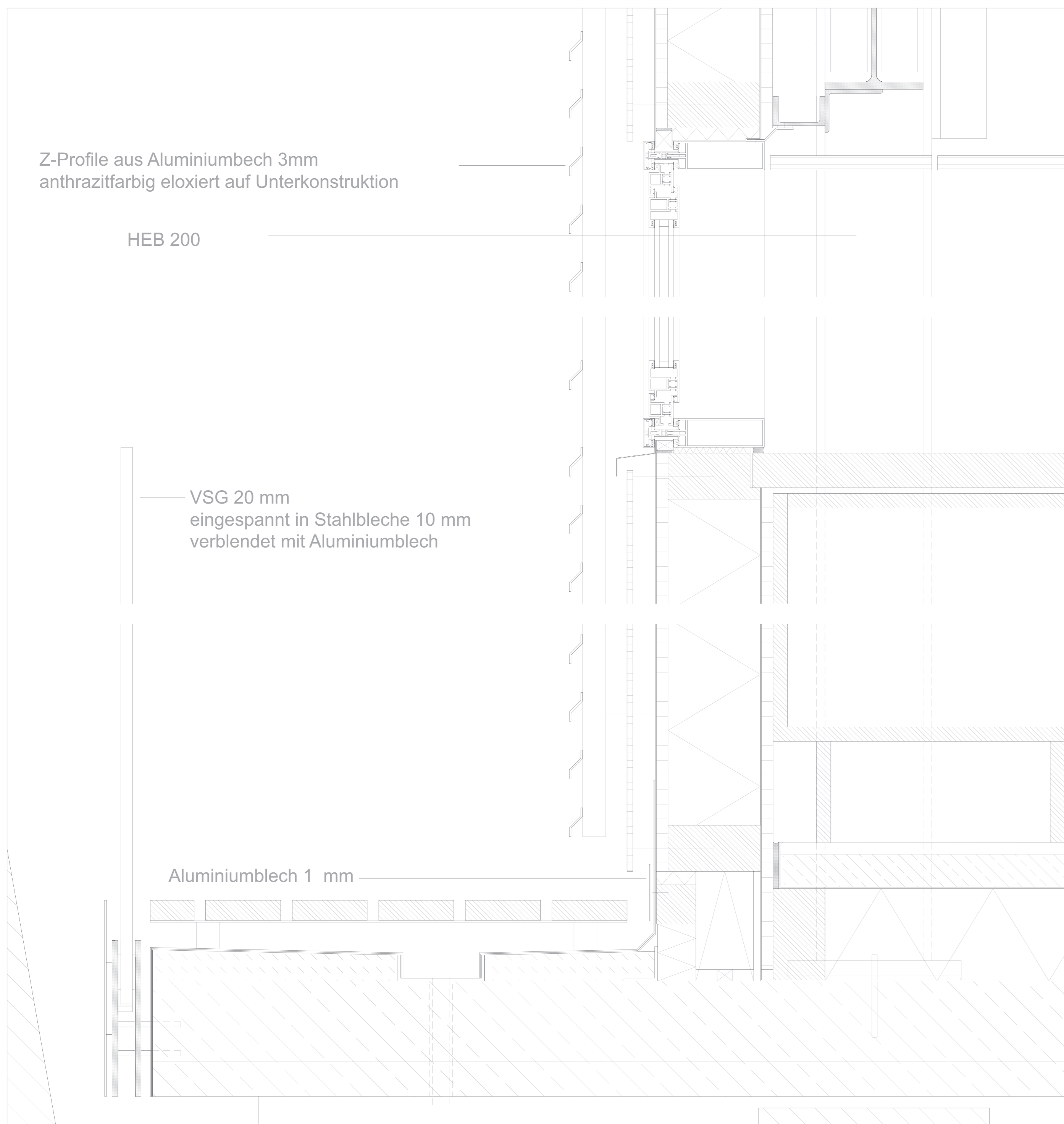
Vertikalschnitt M 1:5 Fassade Küche Horizontalschnitt M 1:5 Fassade Küche
