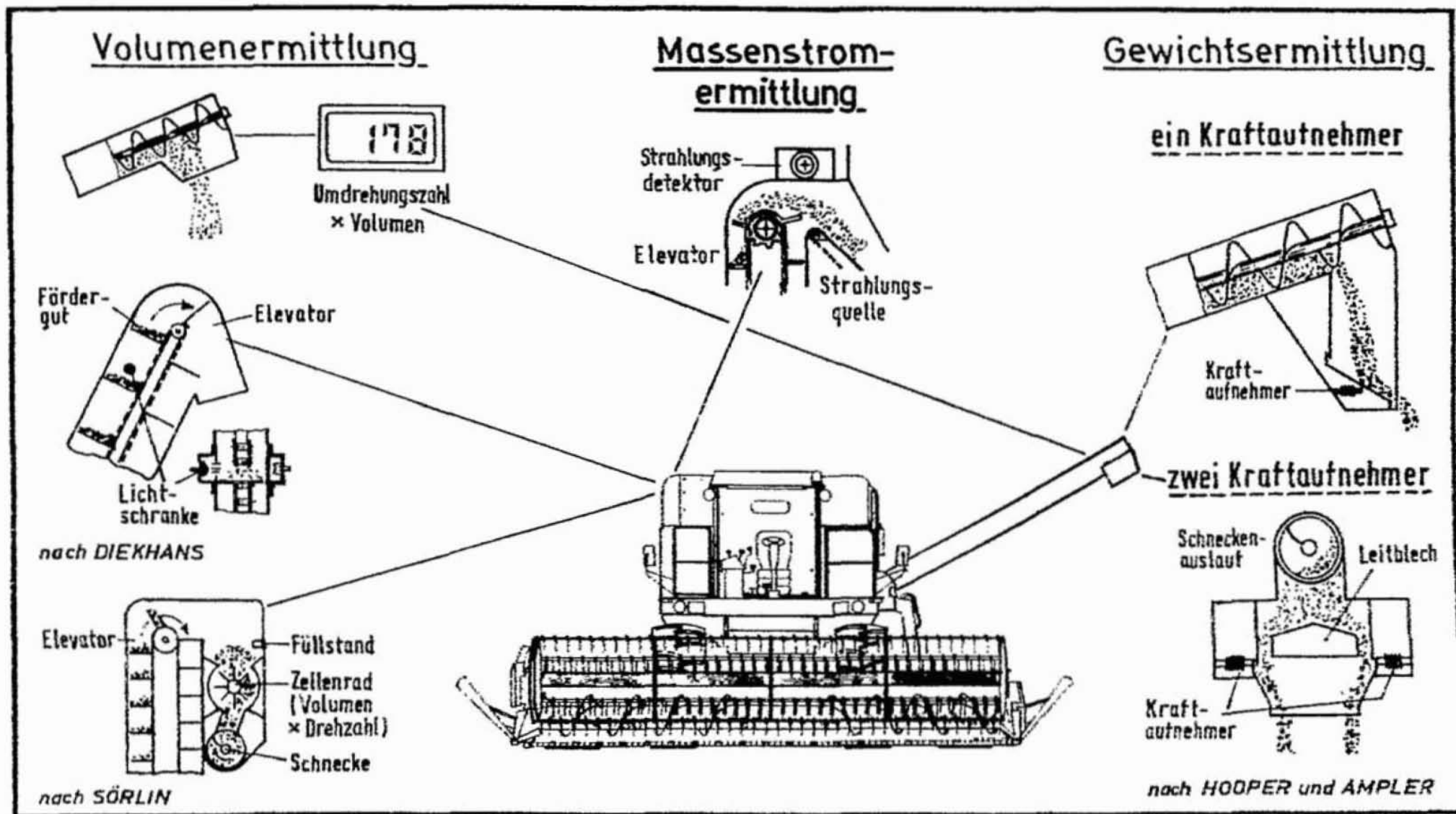
Abbildung 97: Systeme der Ertragsermittlung in Mähdreschern [19].
