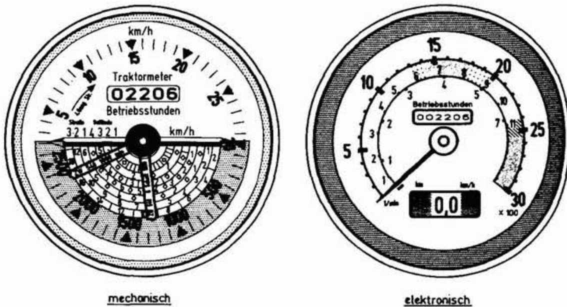
Abbildung 34: Mechanisches und elektronisches Traktometer.
