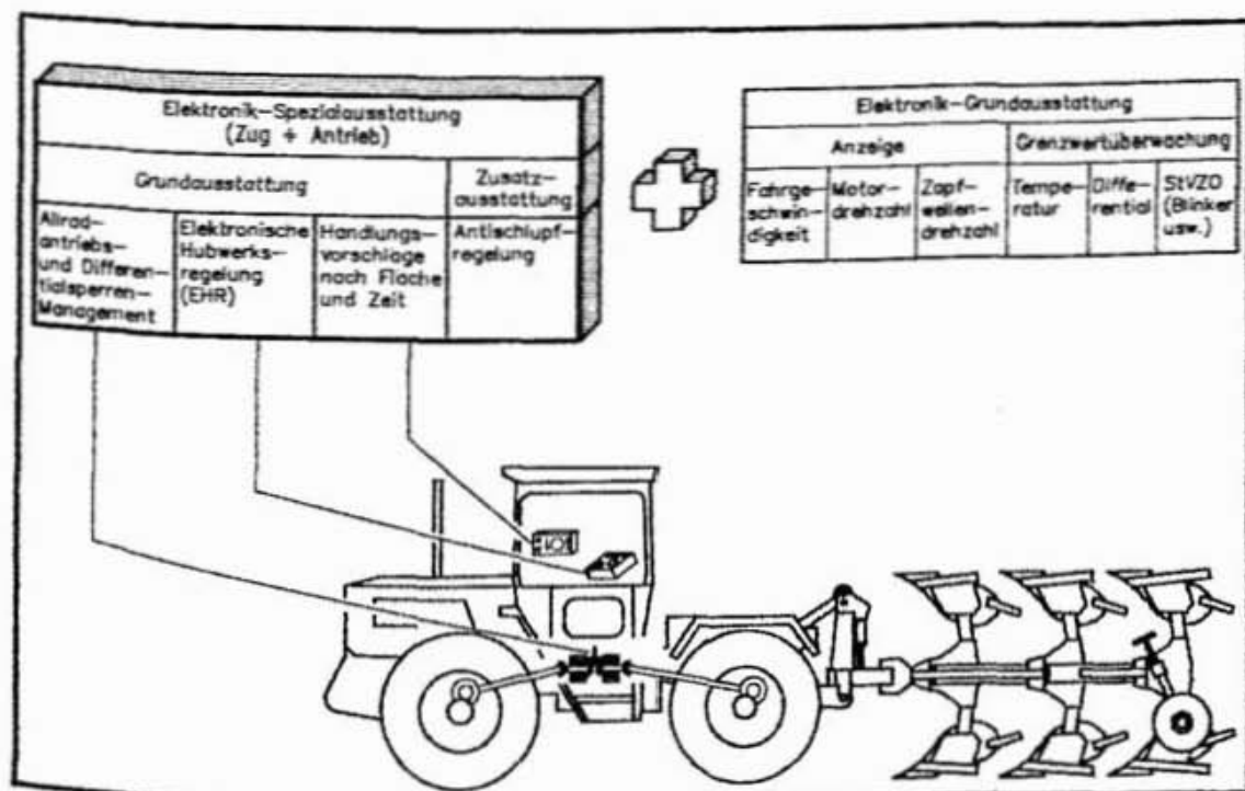
Abbildung 47: Sinnvolle Elektronikanwendungen beim Traktor für schwere Zugarbeiten.
