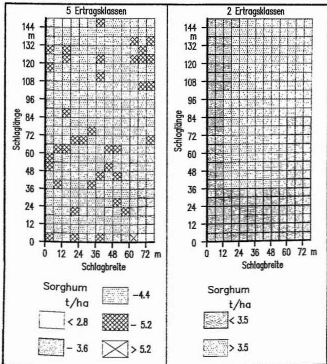
Abbildung 78: Kartierung nach Ernteertrag [14].
