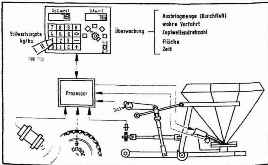
Abbildung 73: Funktion des elektronisch gesteuerten wegabhängigen Wurfstreuers.
