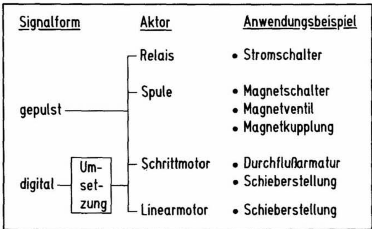
Abbildung 10: Signale, Techniken und Anwendungsbereiche für Aktoren.
