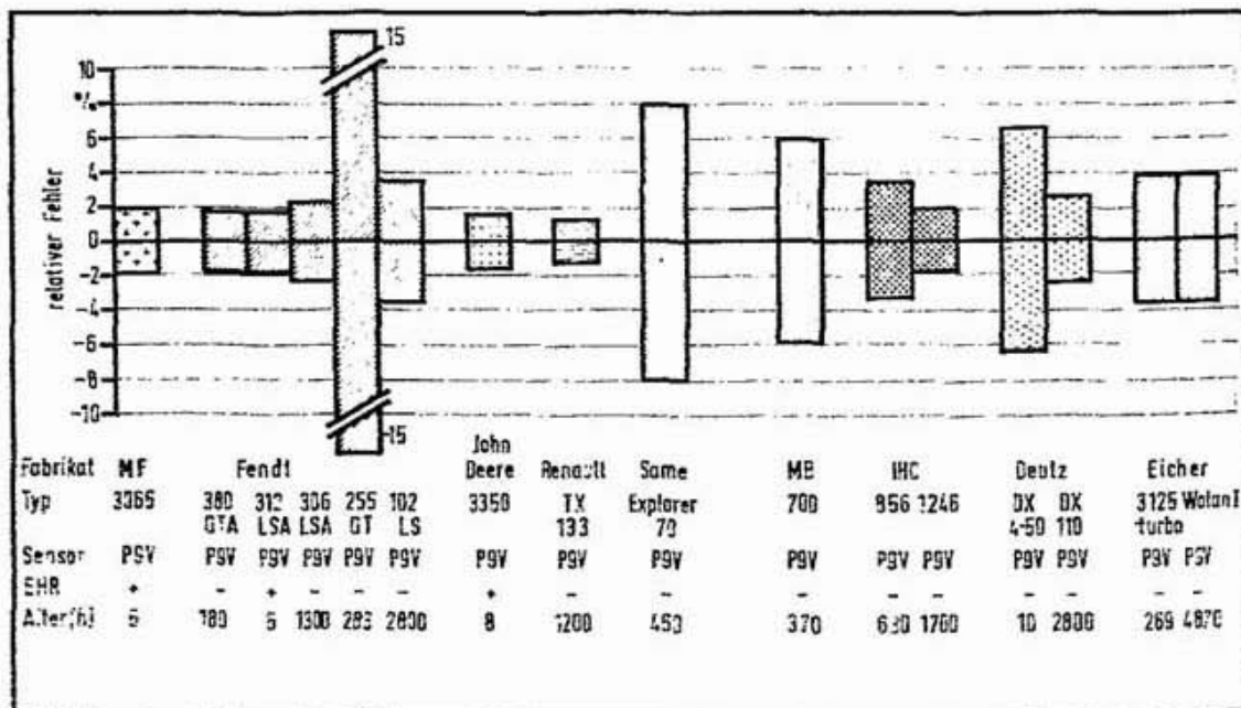
Abbildung 71: Fehler bei Hydraulikdruckmeßsystemen zur Gewichtsermittlung in der Traktordreipunkthydraulik.
