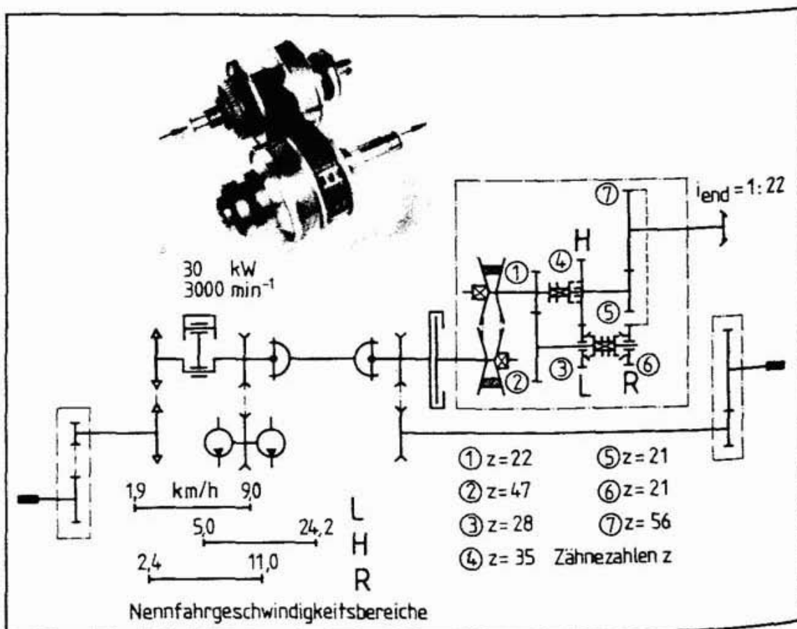
Abbildung 28: Kettenwandler in einem Getriebe zum stufenlosen Fahrtrieb [21].
