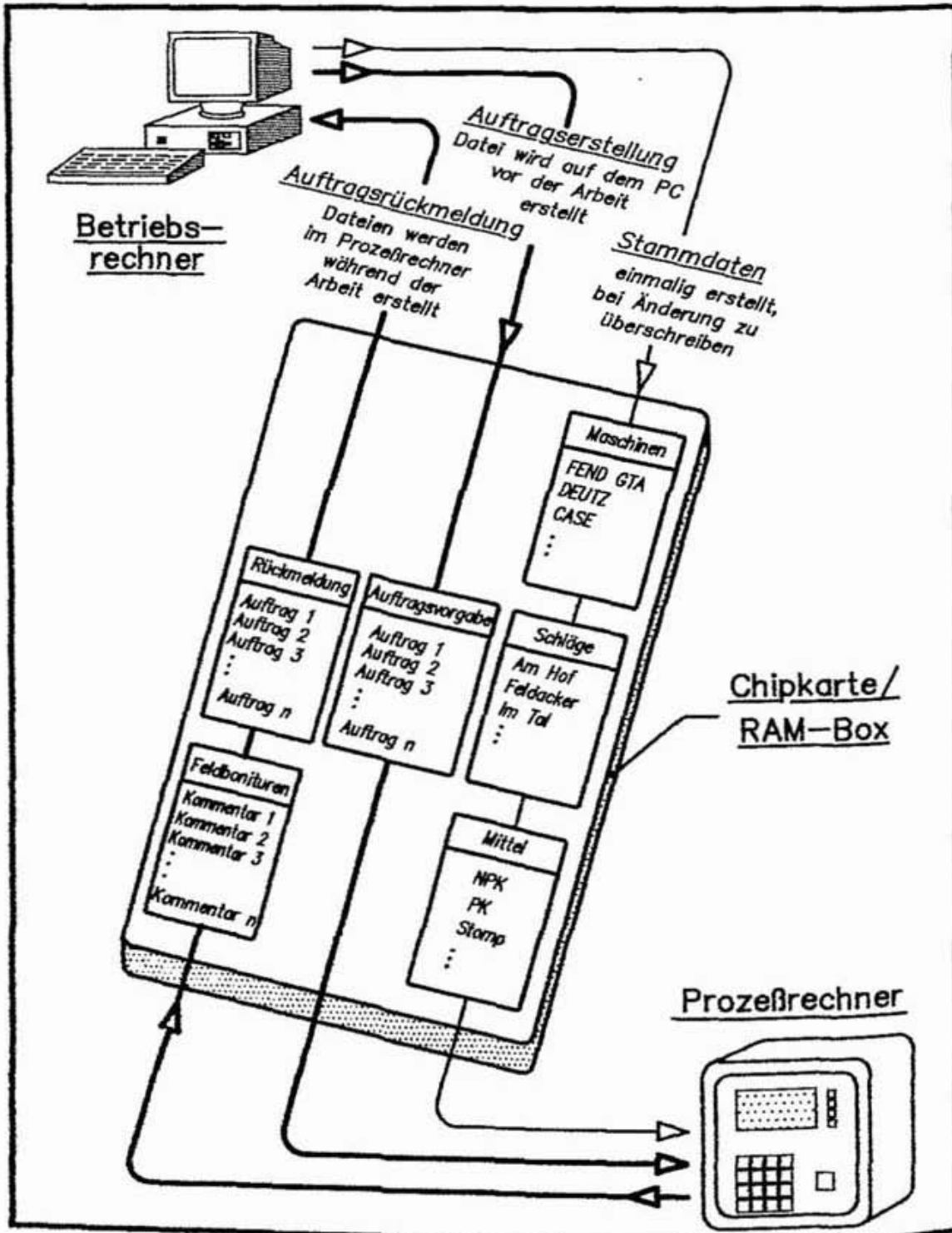
Abbildung 45: Schema eines Datenübergabeprotokolls für die Maschinensteuerung [8].
