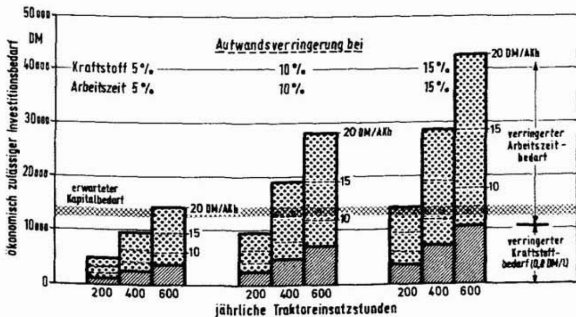
Abbildung 27: Ökonomisch zulässiger Investitionsbedarf für elektronisch schaltbare Getriebe (Traktor mit 125 kW; Dieserverbrauch 24,6 l/h; Kapitalisierungsfaktor = 6,03 aus AfA = 12 Jahre; Zins = 7 %; Reparatur = 4 %.)
