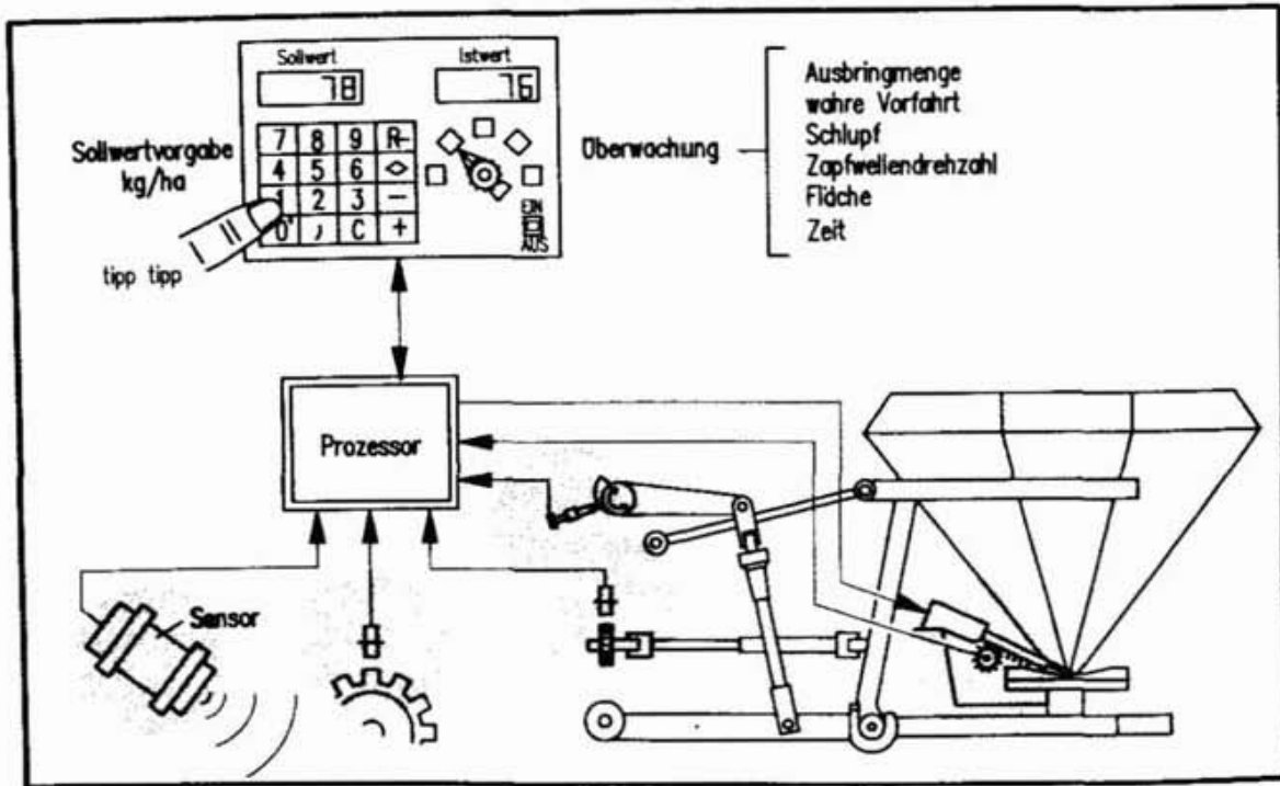
Abbildung 13: Elektronische Regelung (schematisch).
