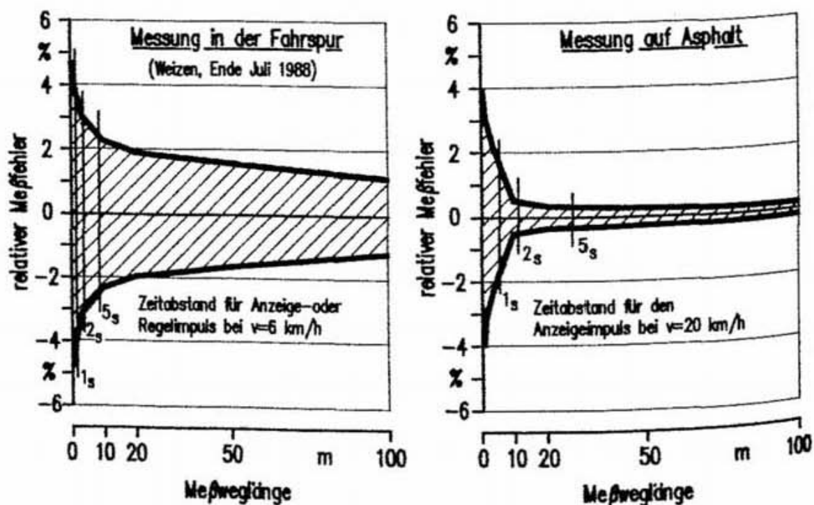
Abbildung 56: Meßgenauigkeit berührungslos arbeitender Wegsensoren.
