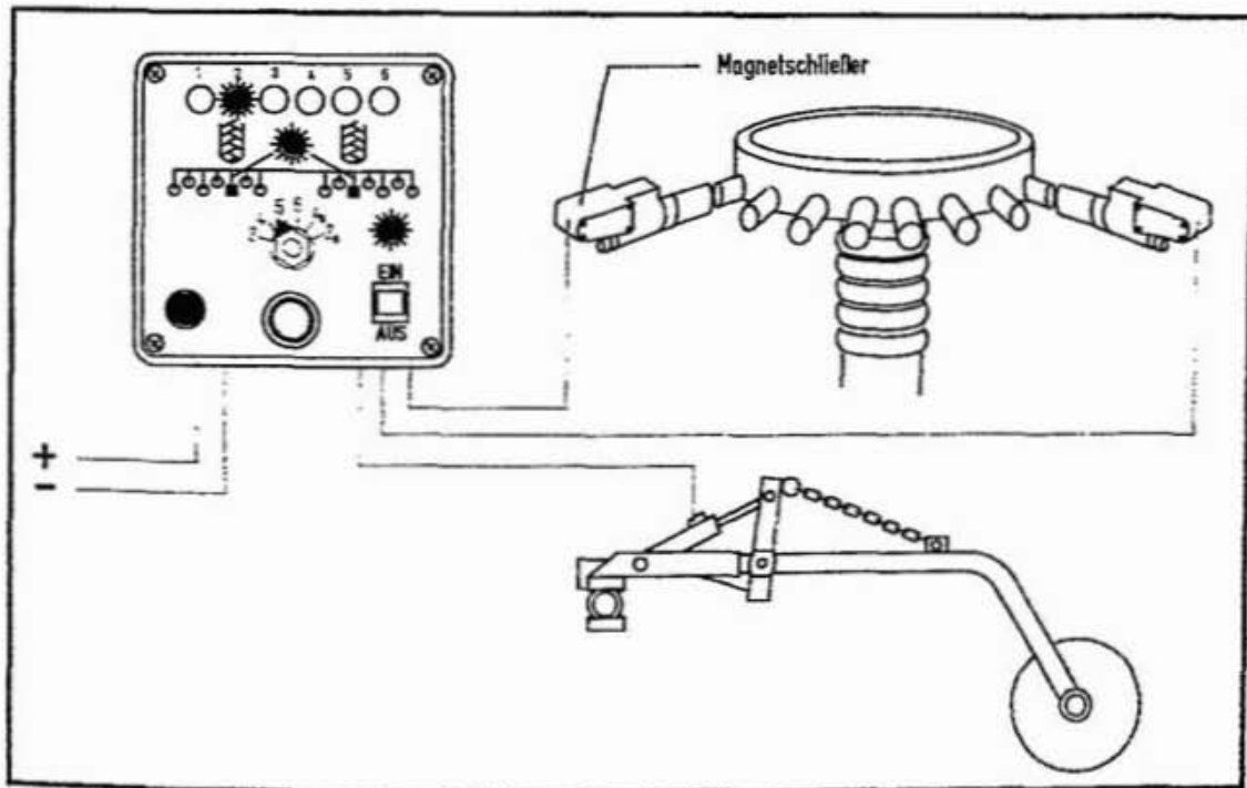
Abbildung 63: Schematische Darstellung einer elektronischen Fahrgassenschaltung [9].
