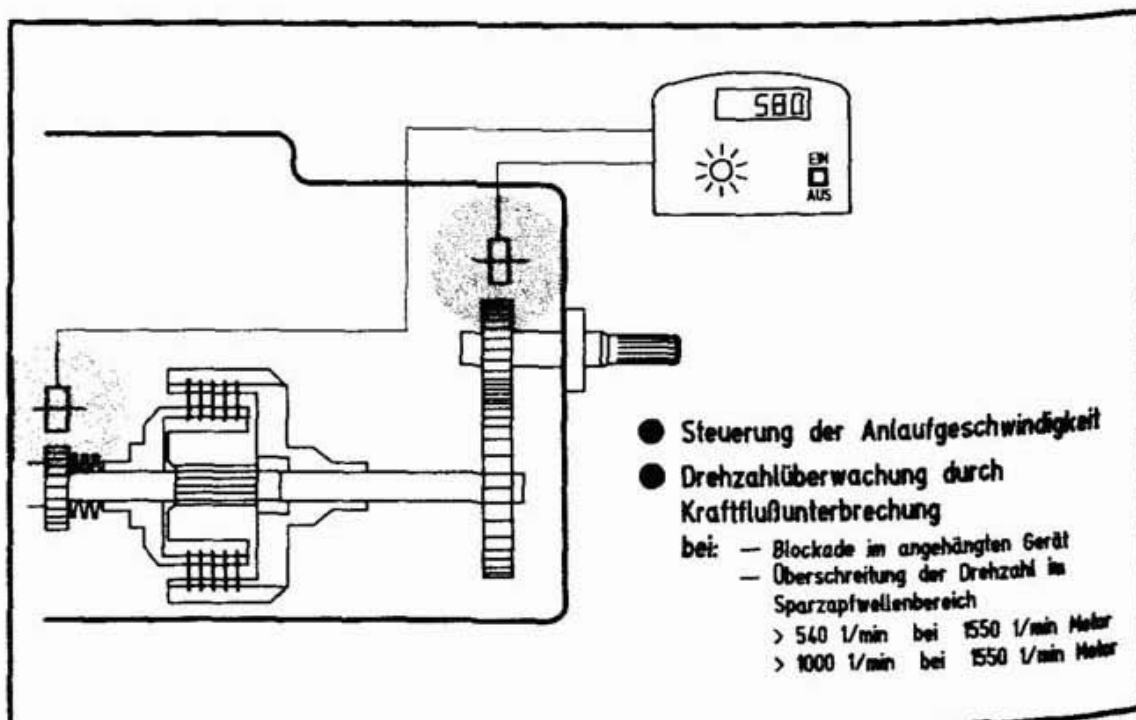
Abbildung 31: Elektronische Zapfwellenüberwachung.
