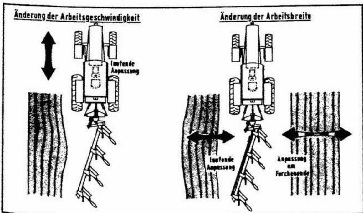
Abbildung 61: Möglichkeiten der elektronischen Pflugsteuerung.
