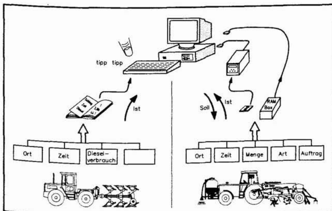
Abbildung 44: Datenübergabe zwischen Traktor und Betriebsrechner.
