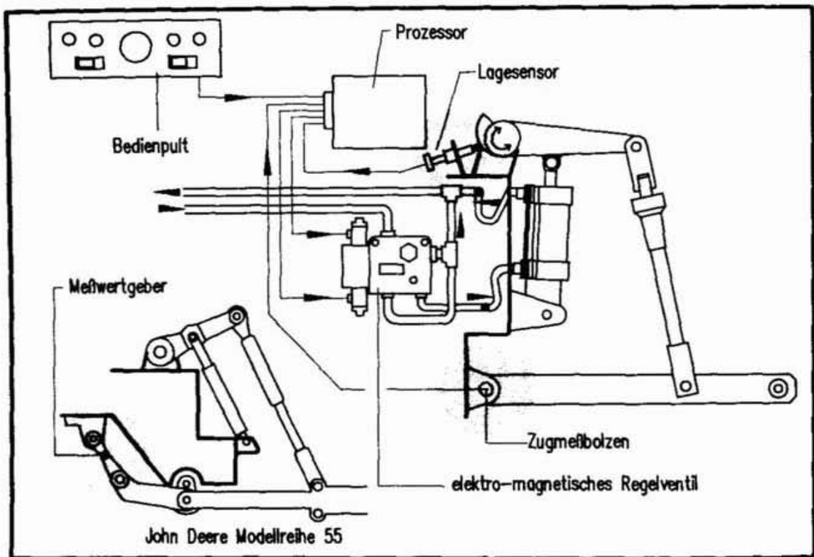
Abbildung 18: Elektronische Hubwerksregelung (schematisch).
