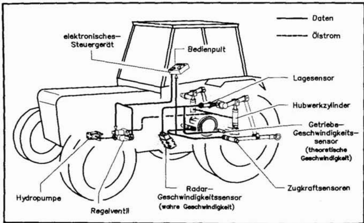
Abbildung 20: Aufbau einer elektronisch gesteuerten Anti-Schlupfregelanlage [1].
