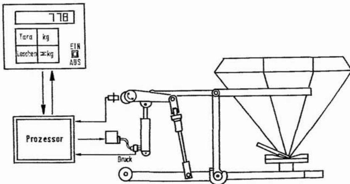
Abbildung 69: Traktorhecklastwaage für das Hydraulikdrucksystem System »eh Elektronik« [11].
