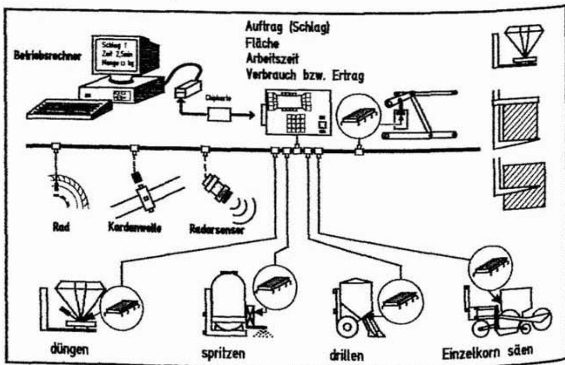
Abbildung 53: Schema des Landtechnik-Bus-Systems.
