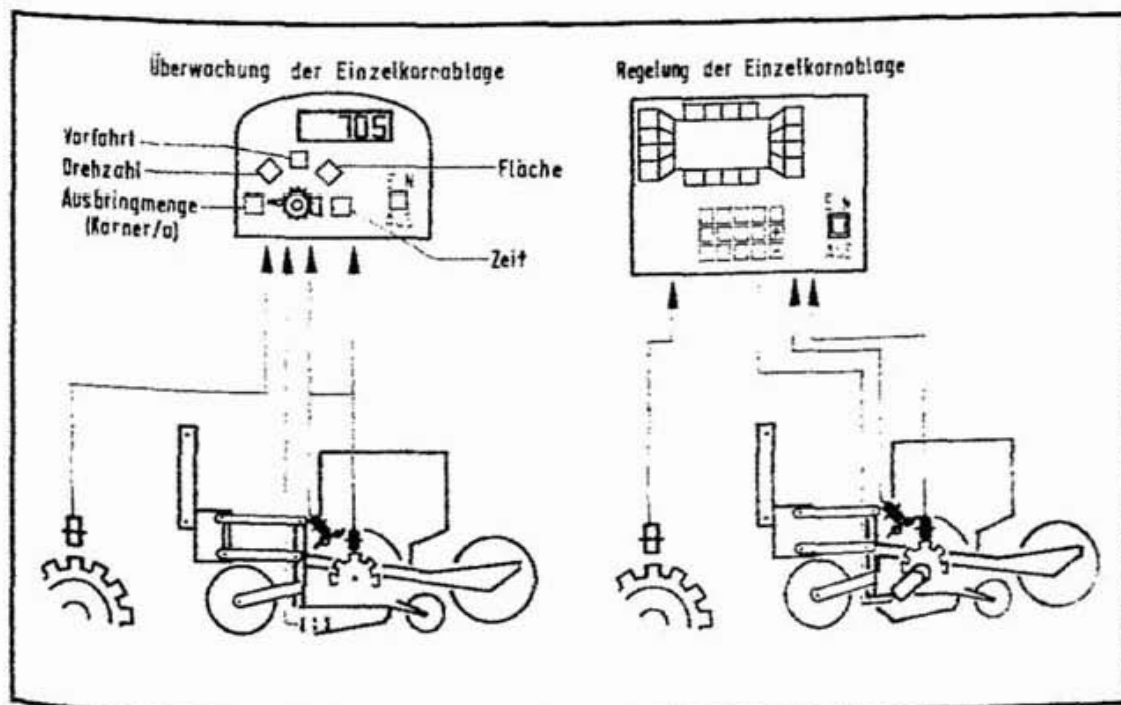
Abbildung 66: Überwachung (links) und Regelung (rechts) der Ausbringmenge bei Einzelkornsägeräten (schematisch).
