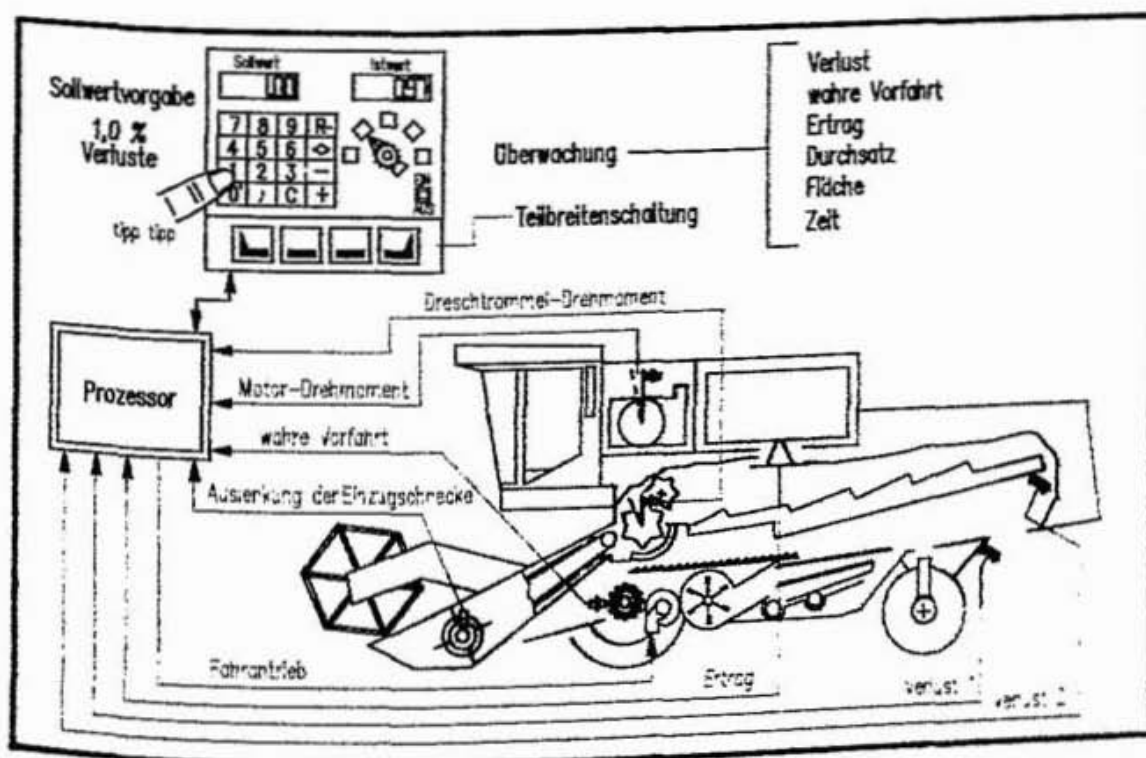
Abbildung 98: Schematischer Aufbau einer elektronischen Durchsatzregelung.
