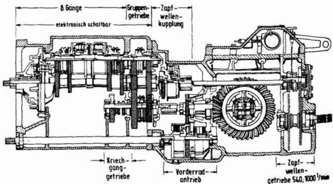
Abbildung 25: Elektronisch schaltbares Stufengetriebe [5].
