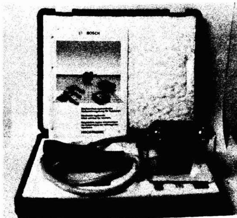
Abbildung 42: Diagnosegerät für die EHR (Testkoffer).
