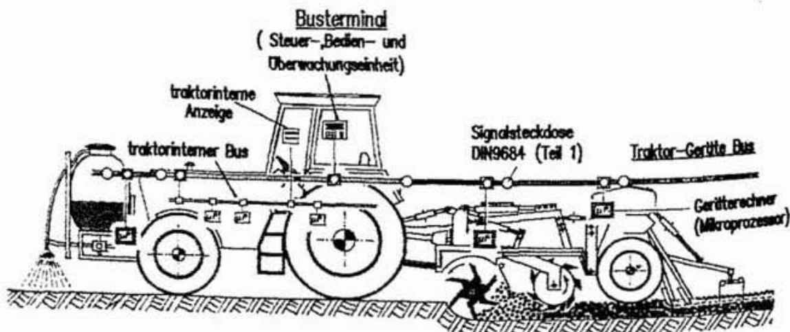
Abbildung 55: Landtechnik-Bus-System (Übersicht).
