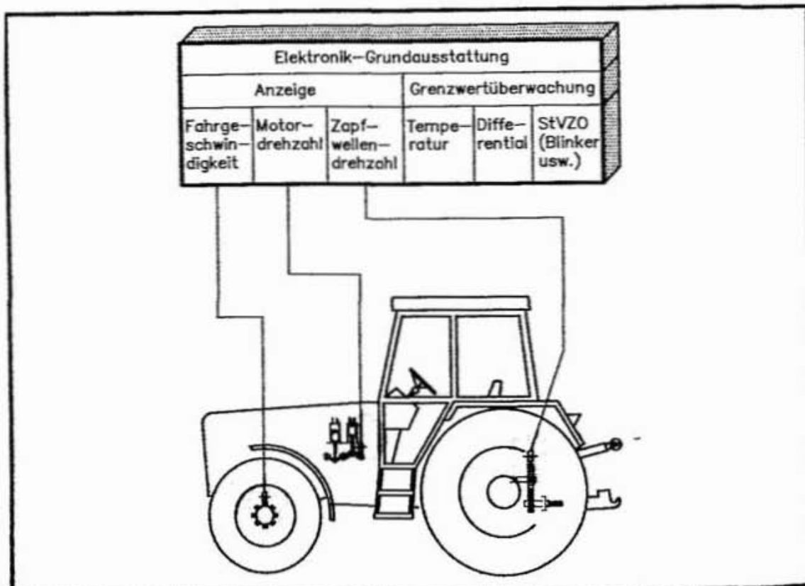
Abbildung 46: Sinnvolle Elektronikgrundausstattung für alle Traktoren.
