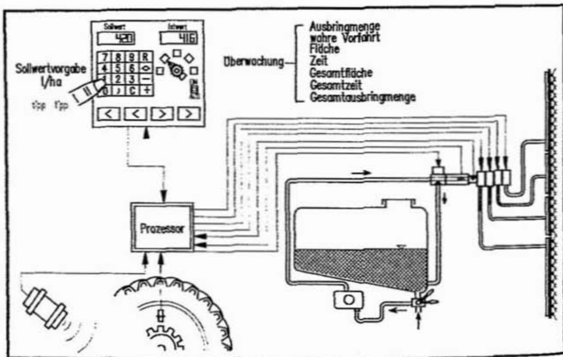
Abbildung 82: Wegabhängige Druckregelung bei Feldspritzen.
