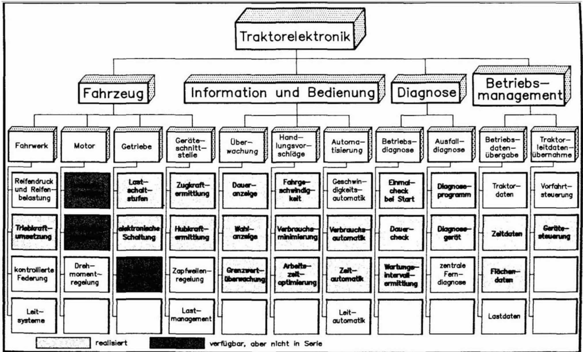
Abbildung 15: Systematischer Überblick über die Einsatzbereiche der Elektronikanwendung im Traktor.
