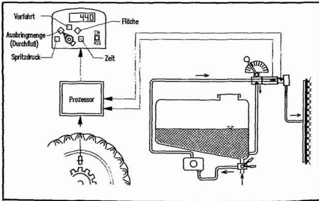
Abbildung 80: Aufbau eines Überwachungssystems für die Feldspritze.
