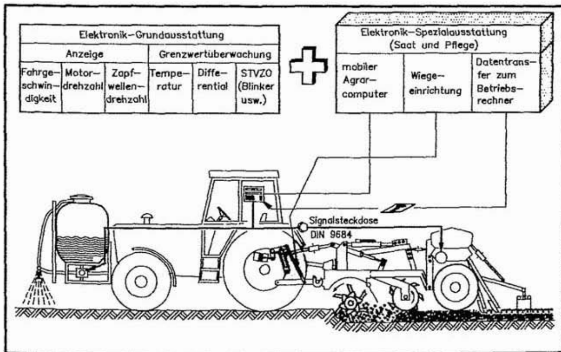
Abbildung 48: Sinnvolle Elektronikanwendungen beim Pflgetraktor.
