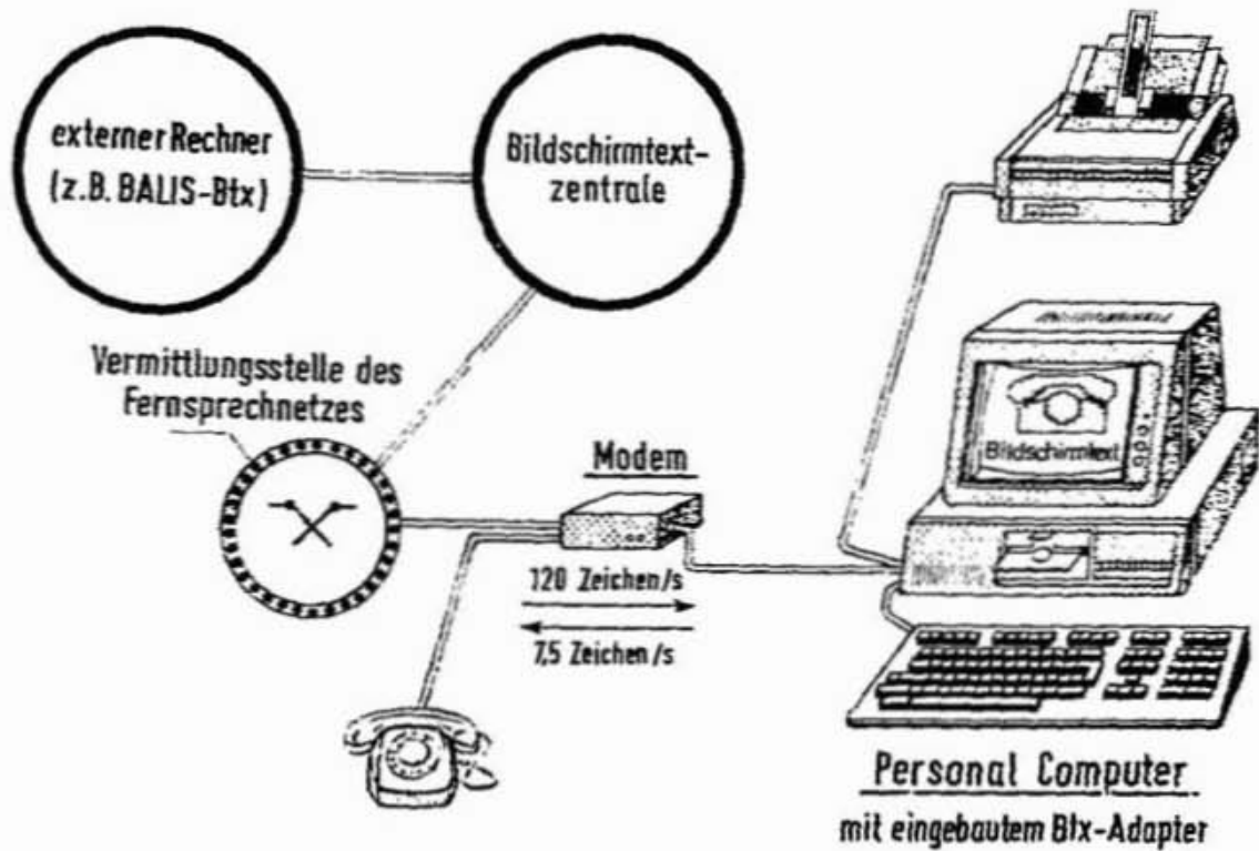
Abbildung 107: Betriebsrechner mit Btx-Anbindung [20].
