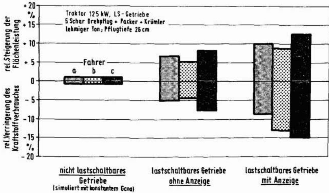
Abbildung 26: Effekte einer Schaltanzeige bei unterschiedlichen Arbeitspersonen [6].
