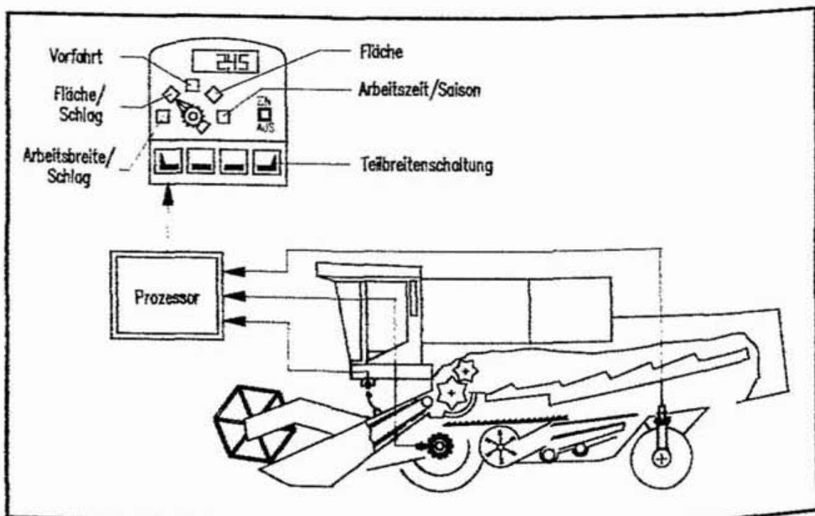
Abbildung 92: Flächenermittlung im Mähdrescher-Bordmonitor.
