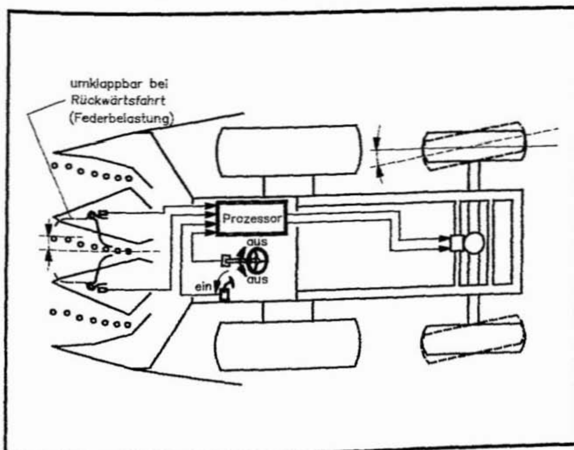
Abbildung 99: Schematischer Aufbau einer automatisierten Lenkung.
