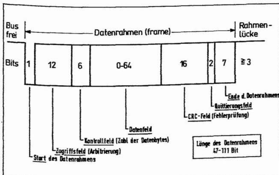
Abbildung 54: CAN-Format im Landtechnik-Bus-System.
