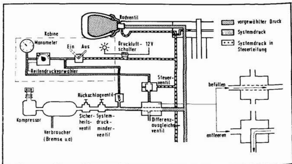
Abbildung 16: Schema einer Reifendruckregelanlage.
