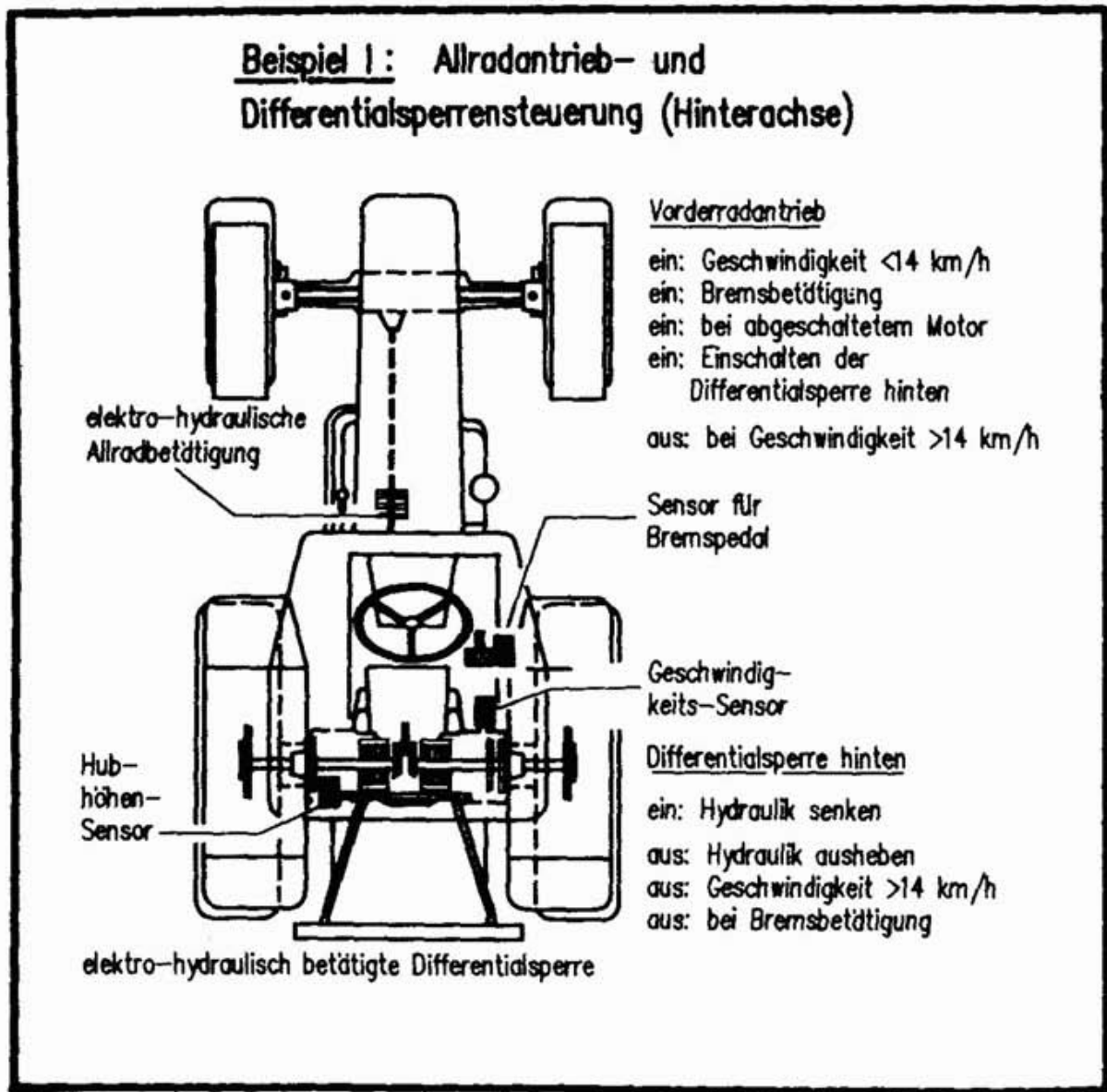
Abbildung 17: Formen des elektronischen Allrad- und Differentialsperrenmanagements (Seite 33 oben).
