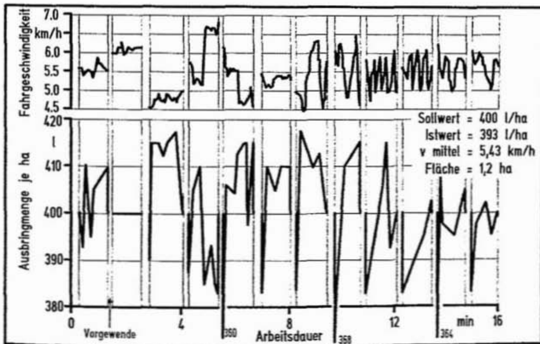
Abbildung 83: Regelgüte bei elektronisch geregelten Feldspritzen [15].
