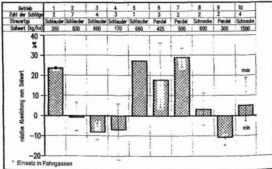
Abbildung 67: Relative Abweichung der ausgebrachten Mineraldüngermengen gegenüber der Soll-Vorgabe.
