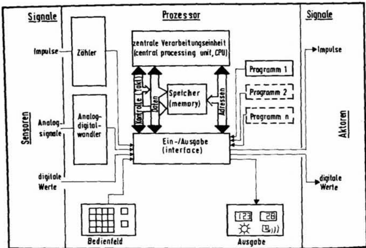
Abbildung 9: Sensorsignale, Prozessor und Aktorsignale.
