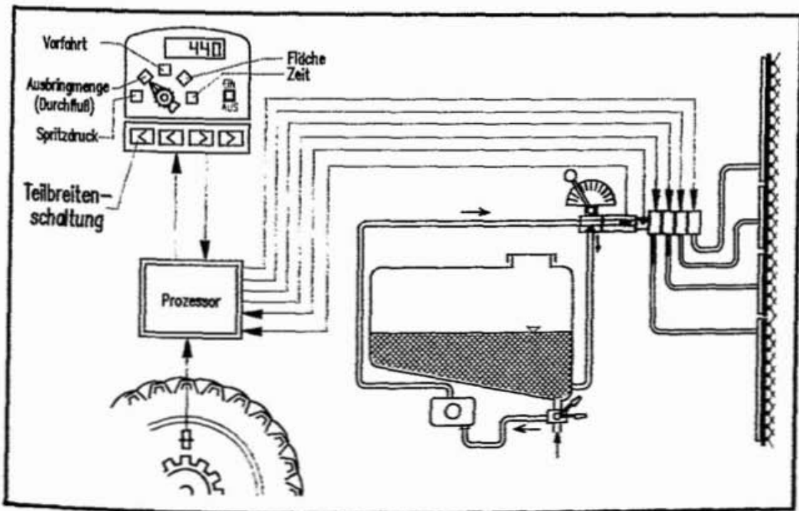
Abbildung 81: Aufbau eines Überwachungssystems für Feldspritzen unter Einbeziehung der Teilbreitenschaltung.
