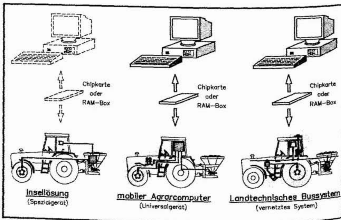
Abbildung 49: Möglichkeiten elektronischer Überwachung, Steuerung und Regelung mit Datentransfer zum Betriebsrechner für Maschinen und Geräten.
