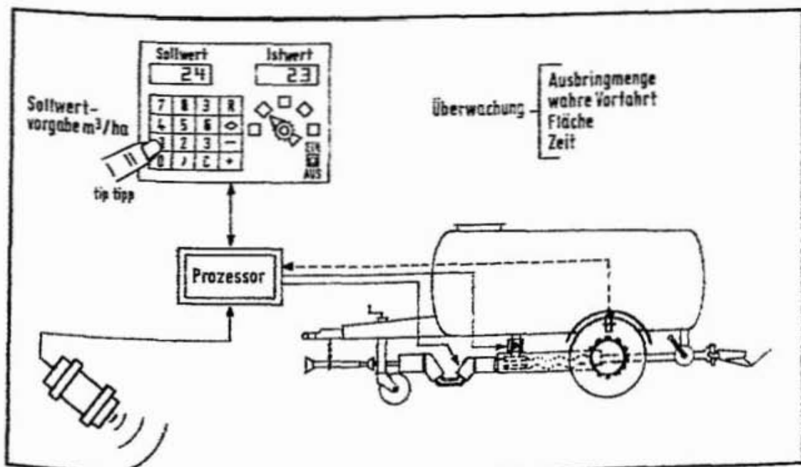
Abbildung 89: Regelsystem für die Gülleausbringung.
