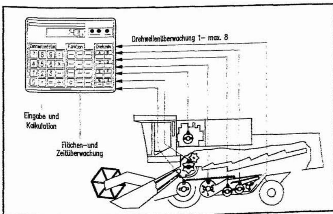
Abbildung 91: Mobiler Agrarcomputer als Drehzahlwächter für den Mähdrescher.
