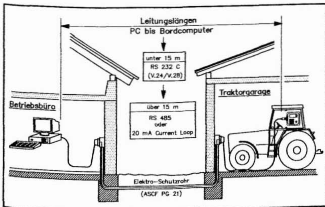
Abbildung 58: Schematische Verbindung von PC und mobiler Prozesstechnik über eine fest installierte Leitung.
