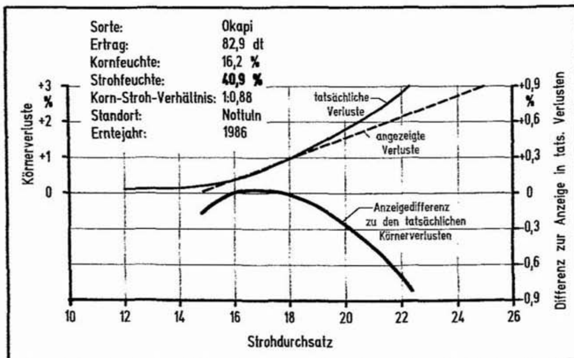
Abbildung 96: Genauigkeit von Körnerverlustsensoren an Mähdreschern bei höherer Strohfeuchte [18].
