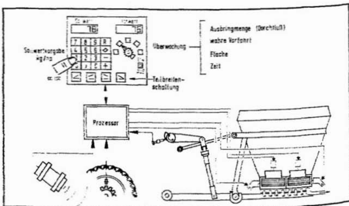
Abbildung 74: Funktion eines elektronisch geregelten Auslegerstreuers.
